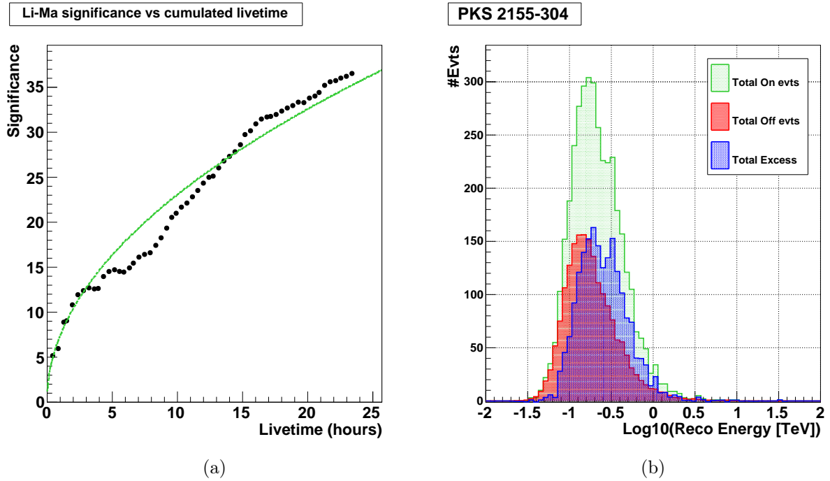
FIGURE 7.5: Détection du BL Lac PKS 2155-304. (a) Significativité en fonction du temps d'observation cumulé. (b) Distributions de l'énergie reconstruite des événements de la région ON (vert), des événements des régions OFF (après normalisation à la région ON, rouge) et de l'excès mesuré (bleu).
