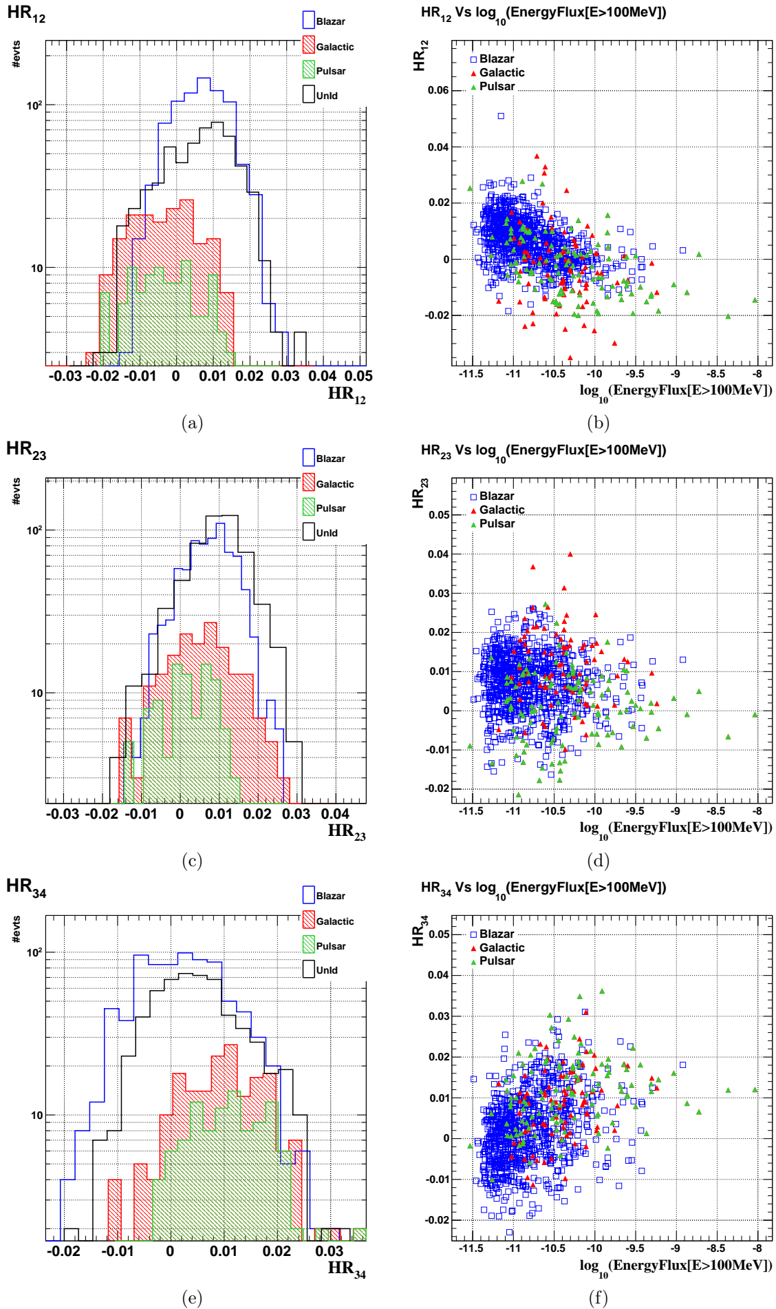
FIGURE 10.3: (a), (c), (e) Distributions des paramètres HR_{12} , HR_{23} , HR_{34} et (b), (d) et (f) leurs corrélations avec le flux en énergie ( E > 100 MeV).
