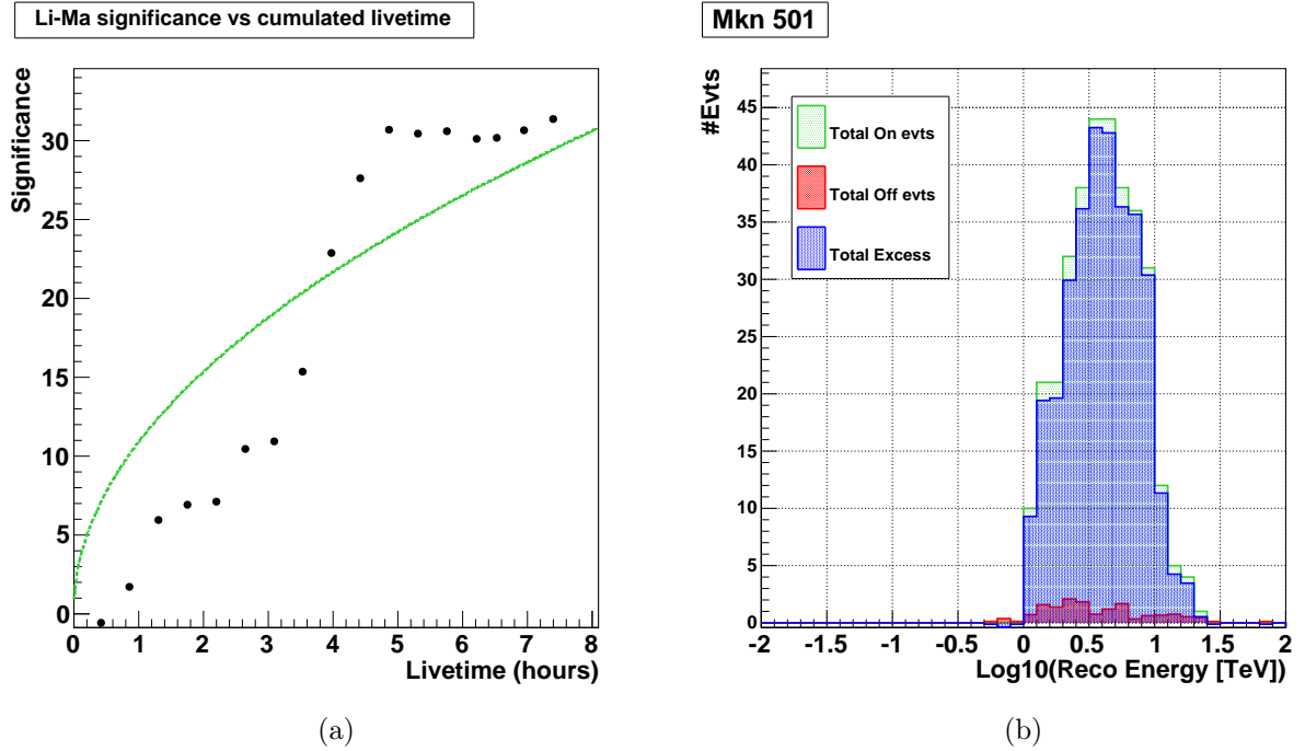
FIGURE 7.7: Détection du BL Lac Mkn 501. (a) Significativité en fonction du temps d’observation cumulé. (b) Distributions de l’énergie reconstruite des évènements de la région ON (vert), des évènements des régions OFF (après normalisation à la région ON, rouge) et de l’excès mesuré (bleu).
