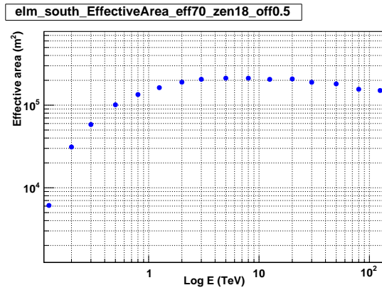
FIGURE 5.17: Surface de collection en fonction de l'énergie vraie pour la configuration « elm » avec \theta = 18^\circ , \delta = 0,5^\circ et \varepsilon = 70\%
