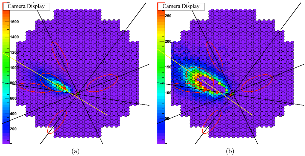
FIGURE 6.4: Évènement \gamma de 7,27 TeV. Illustration de la présence d'un halo dans une image de CT 5 conduisant à une dégradation de la PSF. L'image de droite contient les pixels ayant au plus 15% de la charge du pixel le plus chaud dans l'image entière.
