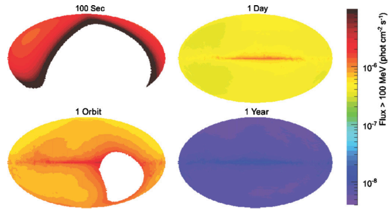
FIGURE 9.3: Sensibilité et couverture du ciel du LAT pour différentes échelles de temps (Crédits : [Atwood et al., 2009]).
