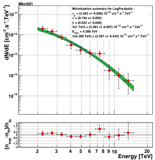
(c) Spectre moyenné sur l'ensemble des données pour une hypothèse de loi de puissance parabolique.
