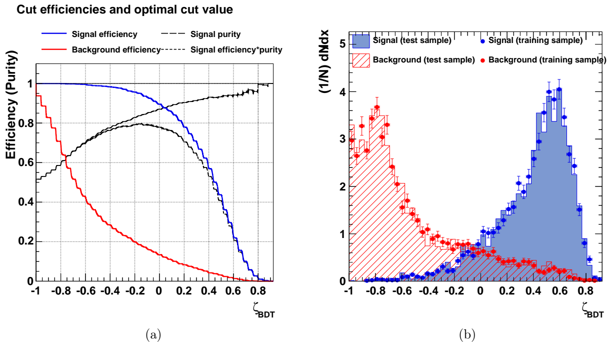
FIGURE 6.19: (a) Efficacités de reconstruction du signal (en bleu) et du fond (en rouge) en fonction de \zeta pour le premier intervalle en N_c et de multiplicité 2. (b) Distributions de \zeta pour les événements \gamma (en rouge), et de fond (en bleu) pour les lots d'entraînements (traits pleins), et de test (points), pour ce même intervalle.
