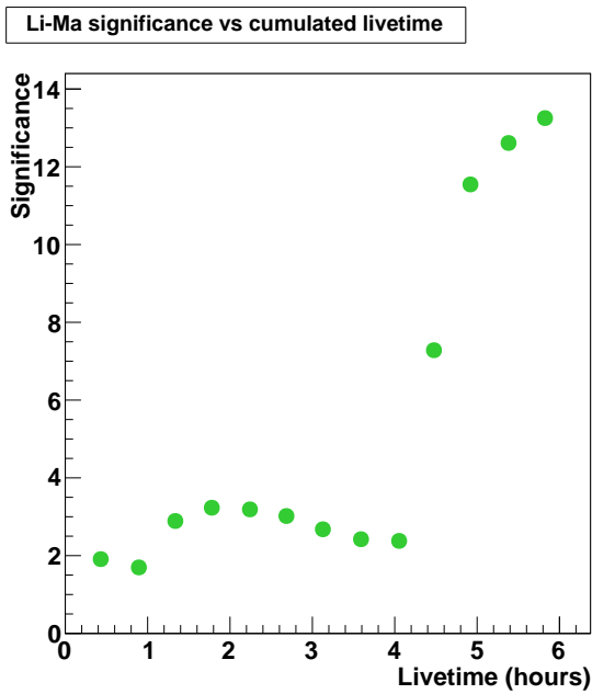
(b) Évolution de la significativité en fonction du temps d'observation effectif.
