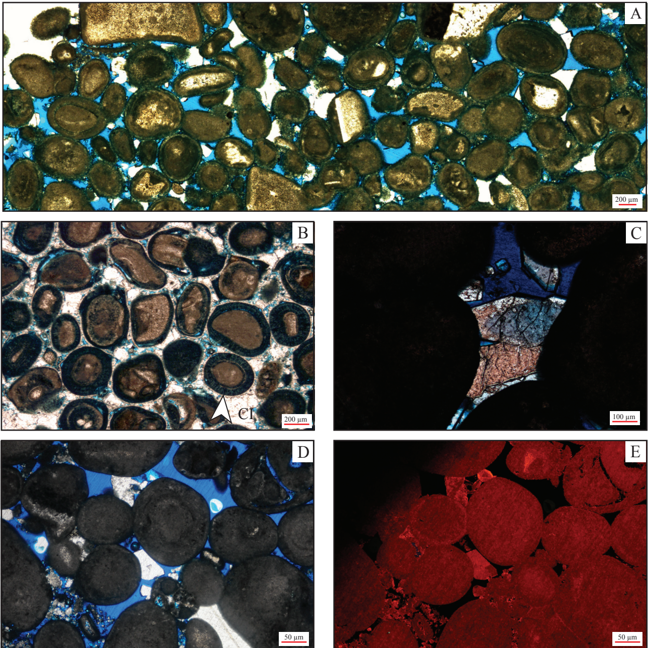
FIGURE 4.18 – Phases diagénetiques observées dans le puits de Banthelu. (A) Echantillon BA-1180 observé en lumière naturelle. Échantillon représentatif de l'intervalle producteur reconnu au top de la carotte. (B) Oolithes dans l'échantillon BA-1253, on remarque la présence d'un ciment isopaque autour des éléments. La macroporosité interparticulaire est mise en évidence par l'inclusion d'une résine bleue. Echantillon représentatif de l'intervalle relativement bien cimenté à la base de la carotte. (C) Echantillon BA-1202, cimentation de blocage après coloration de surface. On note la présence d'une coloration bleue au centre du cristal, signant une calcite ferreuse. (D) Echantillon BA-1202 observé en lumière naturelle. On note la faible microporosité intraparticulaire à la périphérie des grains. (E) Même échantillon observé en cathodoluminescence. Les calcites dans l'espace poreux interparticulaire ne présentent pas de dissolutions.
