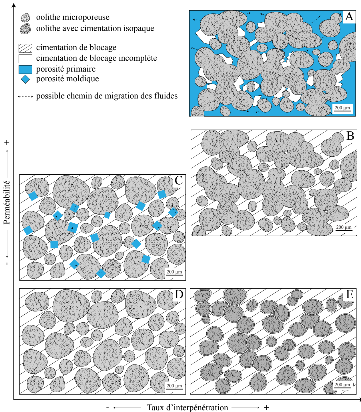
FIGURE 5.20 – Cinq cas de relations entre caractères diagénétiques et perméabilité observés dans la Formation de l’Oolithe Blanche. (A) Grainstone avec des oolithes microporeuses où la porosité interparticulaire initiale est partiellement remplie par de la cimentation de blocage et où le taux d’interpénétration est important. (B) Grainstone avec des oolithes microporeuses où la porosité interparticulaire initiale est totalement remplie par de la cimentation de blocage et où le taux d’interpénétration est important. (C) Grainstone avec des oolithes microporeuses et de la macroporosité moldique. L’interpénétration est nulle. (D) Même grainstone mais sans la macroporsité moldique. (E) Grainstone à oolithes microporeuses avec une phase de cimentation isopaque. La cimentation isopaque est piégée entre les grains durant l’interpénétration.
