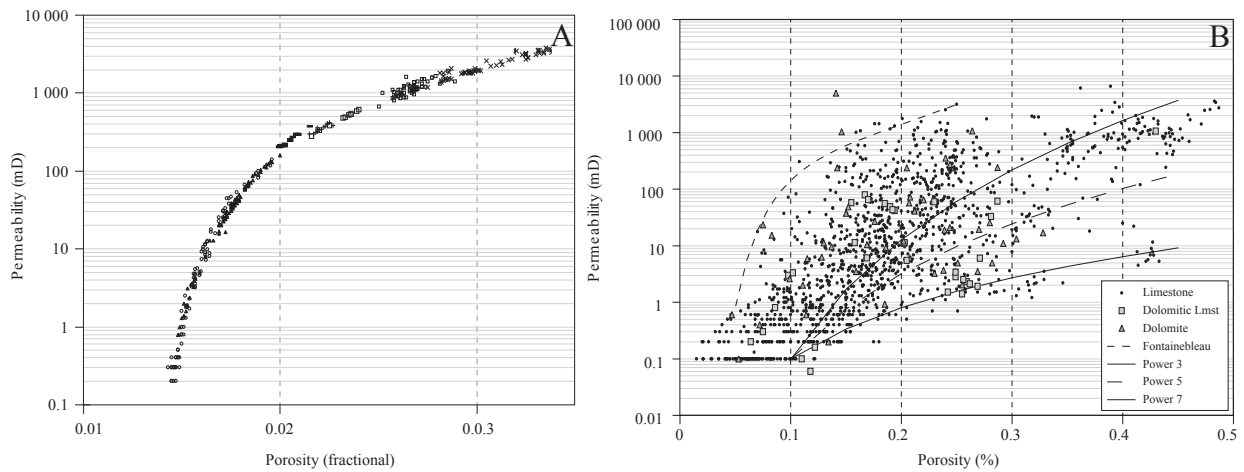
FIGURE 1.4 – Comparaison de la relation perméabilité - porosité dans les grès et les carbonates. (A) Grès de Fontainebleau. (B) Compilation des données de perméabilité et de porosité pour différents réservoirs carbonatés. Modifié d'après Zinszner & Pellerin (2007).
