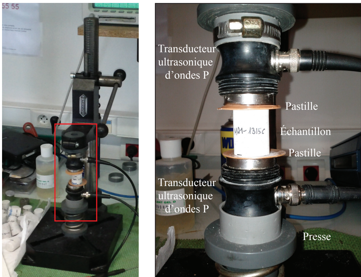
FIGURE 3.12 – Dispositif de mesure de la vitesse de propagation des ondes acoustiques (Université de Cergy-Pontoise).
