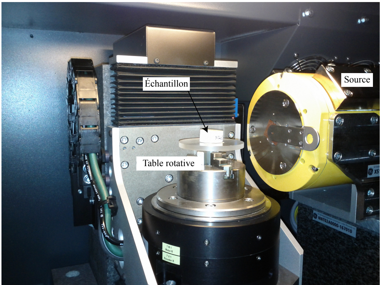
FIGURE 3.14 – Intérieur d'un micro-tomographe Phoenix nanotom GE assisté par ordinateur (Université Catholique de Louvain, Belgique).
