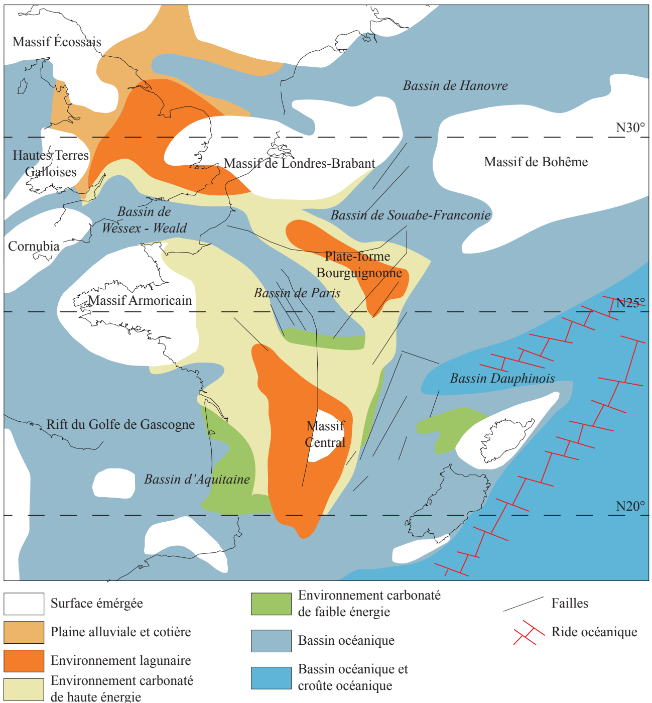
FIGURE 2.2 – Paléogéographie de l'Europe Occidentale au Bathonien. Modifié d'après Enay & Cariou (1980) ; Thierry & Barrier (2000) dans Brigaud et al. (2009). Les paléolatitudes au Bathonien sont indiquées. Le tracé des côtes (actuel) n'est reporté que pour faciliter la lecture.
