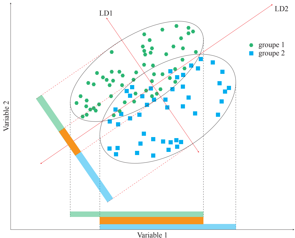
FIGURE 3.15 – Principe de la LDA. La recherche des axes discriminants permet une meilleur séparation d'au moins deux groupes de données (dans le cas ici présenté) en minimisant le chevauchement des champs de variance inter-classe (zone orange).
