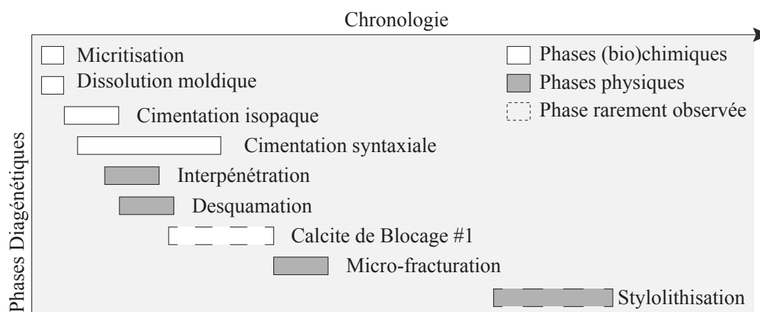
FIGURE 4.19 – Chronologie relative de mise en place des phases diagénétiques reconnues dans le secteur centre. La stylolithisation est une phase physique associée à des phénomènes de dissolution chimique.
