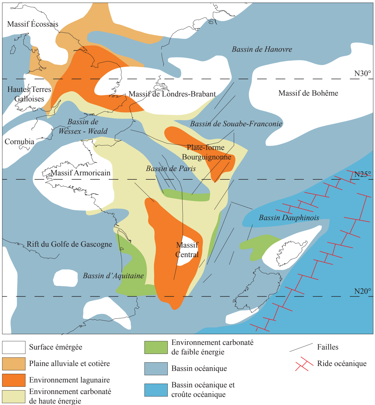
FIGURE 2.2 – Paléogéographie de l'Europe Occidentale au Bathonien. Modifié d'après Enay & Cariou (1980) ; Thierry & Barrier (2000) dans Brigaud et al. (2009). Les paléolatitudes au Bathonien sont indiquées. Le tracé des côtes (actuel) n'est reporté que pour faciliter la lecture.
