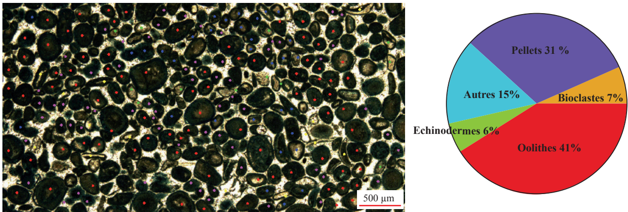
FIGURE 3.5 – Exemple de comptage et représentation graphique du résultat.
