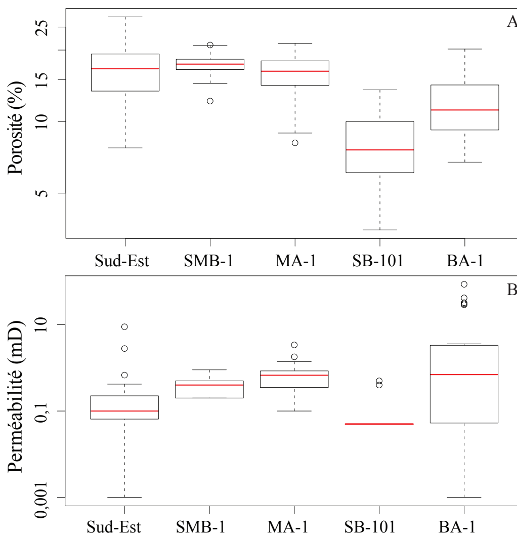
FIGURE 5.15 – Boîtes à moustaches de la porosité (A) et de la perméabilité (B) pour tous les puits et les carrières des secteurs étudiés. SMB-1 : Saint-Martin-de-Bossenay, MA-1 : Mailly-le-Camp, SB-101 : Saint-Brice et BA-1 : Banthelu.
