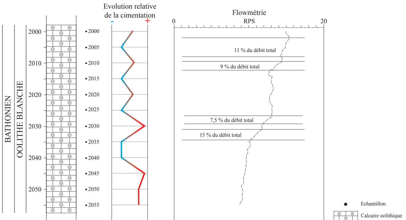
FIGURE 2.13 – Log du puits de Sucy-en-Brie (GSUC3). Stratigraphie et position des échantillons.
