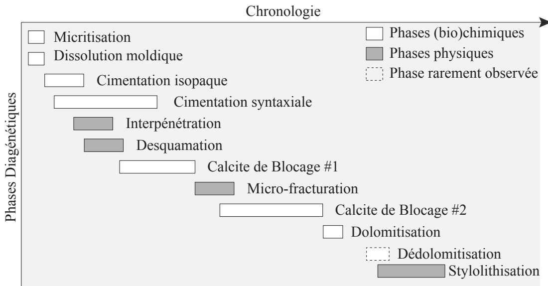
FIGURE 4.14 – Chronologie relative de mise en place des phases diagénétiques pour le secteur médian. La stylolithisation est une phase physique associée à des phénomènes de dissolution chimique.
