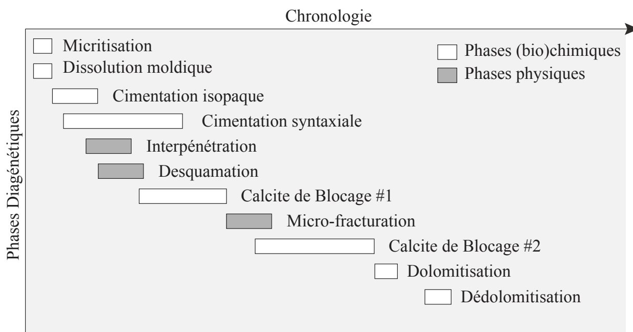
FIGURE 4.4 – Chronologie relative de mise en place des phases diagenétiques reconnues dans le secteur sud-est du bassin de Paris.
