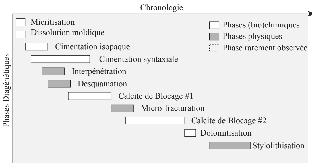
FIGURE 4.7 – Chronologie relative de mise en place des phases diagénétiques reconnues dans le puits de Saint-Martin-de-Bossenay. La styolithisation est une phase physique associée à des phénomènes de dissolution chimique.
