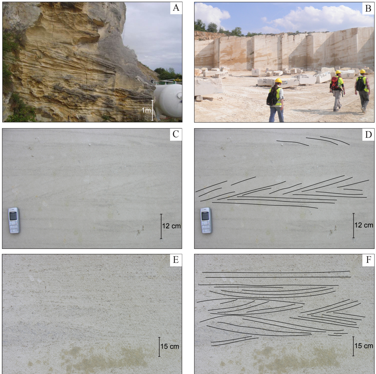
FIGURE 2.6 – Exemples de structures sédimentaires observées dans les carrières de Bourgogne. (A) Mégarides et litages plans de haute énergie, sous-faciès de shoal oolithique, carrière de Ravières. (B) Grandes structures composées d'un empilement de clinofformes progradants. On remarque la morphologie en lobe quand la surface des structures est observable, sous-faciès de Lobe Oolithique Progradant, carrière de Massangis. (C) Rides sigmoïdes, stratifications en arrêtes de poissons ou herring-bones et laminations planes, sous-faciès Tidal, carrière de Massangis. (D) Schéma des structures sédimentaires observée en C. (E) Stratification en arrêtes de poisson, sous-faciès Tidal, carrière de Massangis. (F) Schéma des structures sédimentaires observée en E.
