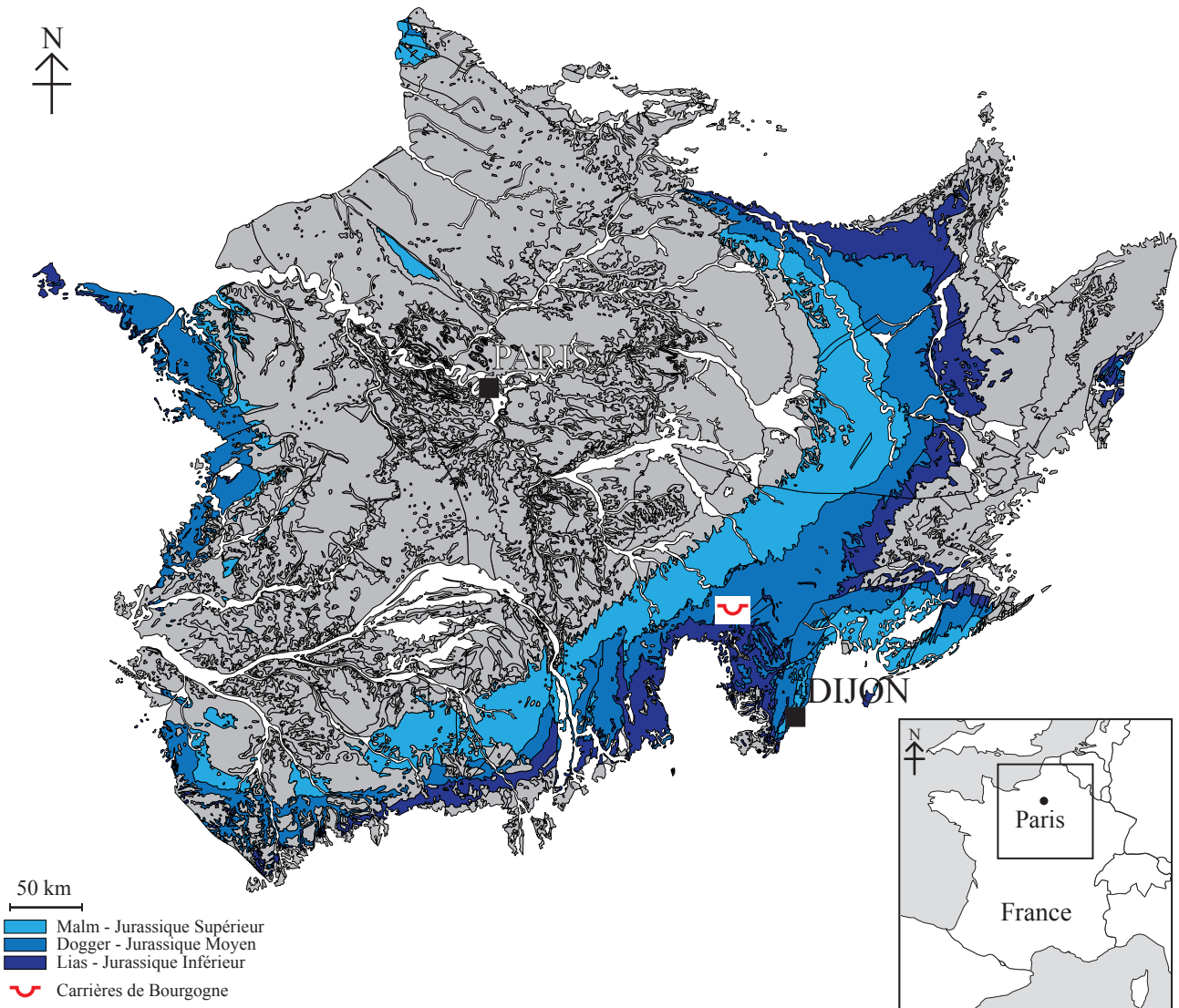
FIGURE 2.1 – Carte simplifiée du bassin de Paris. Seuls les terrains Jurassiques sont distingués (en bleu). Les terrains sous- (Trias) et sus-jacents (Crétacé et Cénozoïque) étant uniformément figurés en gris.
