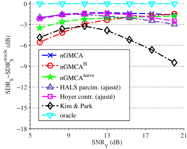
Figure IV.12 – SDR de la reconstruction ( SDR_S ) moins celui de l'oracle en fonction du niveau de bruit sur les données en dB ( SNR_Y ) ( p_S = 50\% , r = 15 , moyenné sur 192 simulations)
