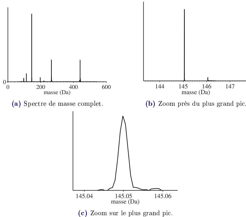
Figure VI.2 – Exemple de spectre de masse à un temps t .
