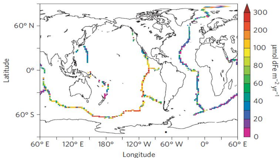
Figure II-II. Estimation des flux hydrothermaux de fer dissous en \mu\text{mol}/\text{m}^2/\text{an} [Tagliabue et al., 2010].
