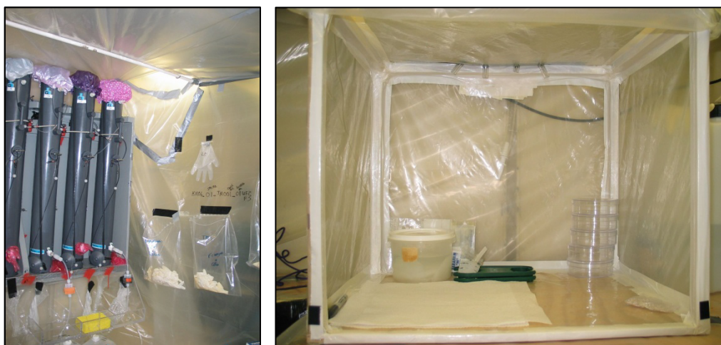
Figure II-3. Le laboratoire « bulle » durant la campagne EUCFe. A gauche, zone de prélèvement. A droite, aménagement d'une hotte à air filtré au sein de la bulle.
