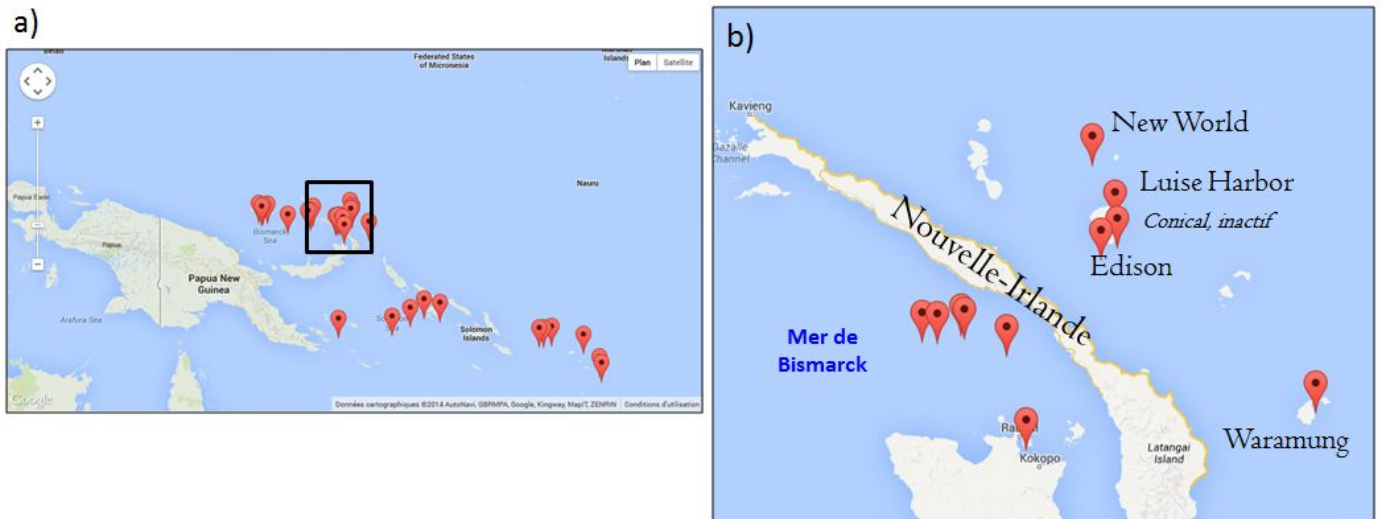
Figure II-3. Carte des monts hydrothermaux actifs dans a) le Pacifique Equatorial Ouest, le carré noir représente un zoom sur la Nouvelle-Irlande dans la figure b). Seuls les monts hydrothermaux localisés au large de la Nouvelle Irlande sont spécifiés. Lorsque les monts hydrothermaux sont inactifs, cela est spécifié à côté de leur nom. Source = http://vents-data.interridge.org/ventfields-geofield-map .
