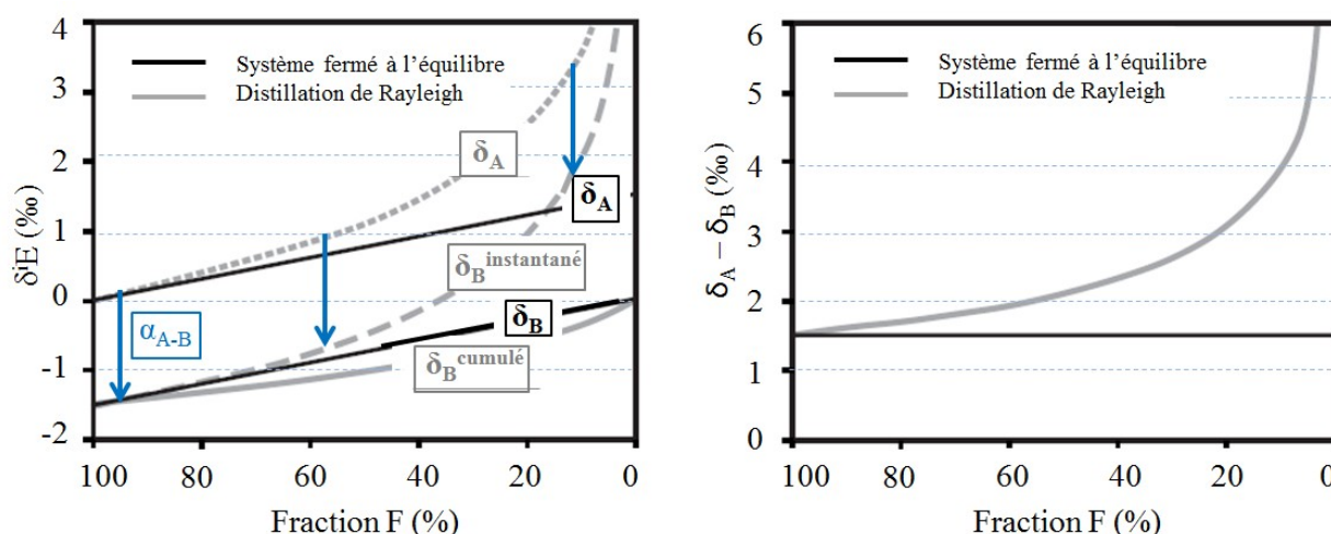
Figure III-3. Comparaison entre les fractionnements isotopiques produits dans un système fermé à l'équilibre et pendant la distillation de Rayleigh. Ici A est le produit et B le réactif et on regarde l'évolution de leur propriété au cours de la transformation de A en B, F étant la fraction de A restante exprimé en %. La composition isotopique de l'élément, \delta^E (‰), est représentée sur l'axe des ordonnées du graphique de gauche. Sur ce graphique, les droites noires en trait plein représentent les contraintes imposées par un système fermé à l'équilibre où A et B sont constamment maintenus en équilibre isotopique. Les lignes grises modélisent la distillation de Rayleigh. Le produit B est instantanément isolé des échanges isotopiques avec A après sa formation, produisant ainsi des variations isotopiques plus importantes que dans le cadre d'un système fermé à l'équilibre. Les \delta^E de la phase A restante sont représentées en petits tirets, celles du produit B instantané avec des longs tirés, et le produit B cumulé et représenté par la ligne grise en trait plein. La différence des compositions isotopiques, \delta_A - \delta_B (‰), est représentée sur l'axe des ordonnées du graphique de droite. Elle est constante pour les fractionnements dans un système fermé à l'équilibre (ligne noire). En revanche, cette différence isotopique varie pendant le fractionnement de Rayleigh (ligne grise incurvée), même pour un facteur de fractionnement \alpha_{A-B} constant (qui reflète alors les conditions d'équilibre). Ce facteur de fractionnement constant est représenté par les flèches bleues [Johnson et al., 2004].
