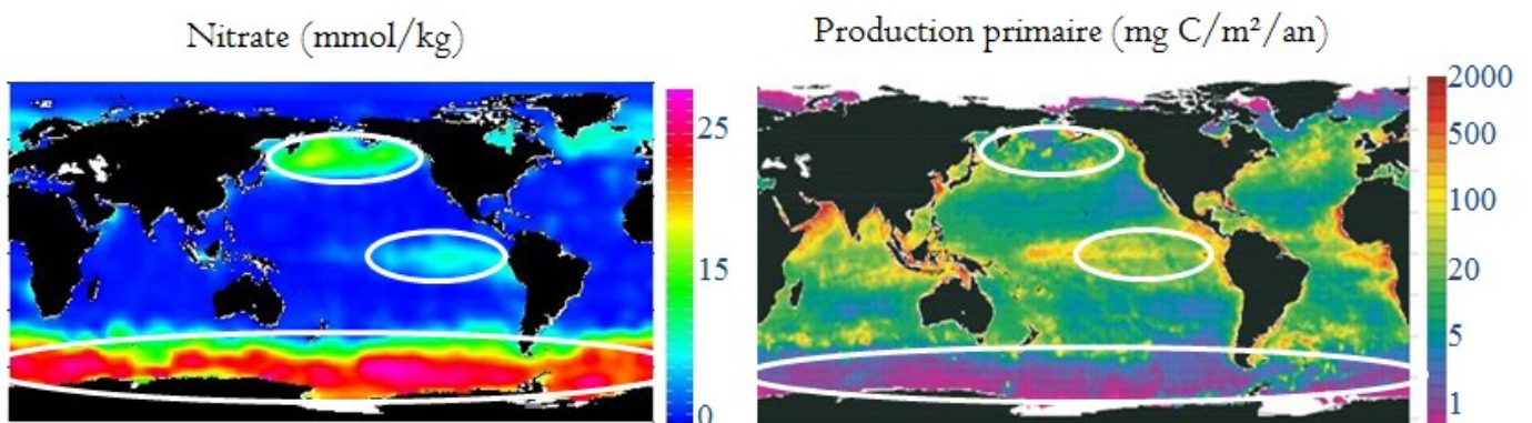
Figure I-2. Distribution des concentrations de surface des nitrates (à gauche) en \text{mmol}/\text{kg} , et distribution de la production primaire dans les eaux de surfaces (à droite) en \text{mg}(\text{C})/\text{m}^2/\text{an} . Les trois zones HNLC sont représentées par des ellipses blanches ( http://earthobservatory.nasa.gov/GlobalMaps/ ).
