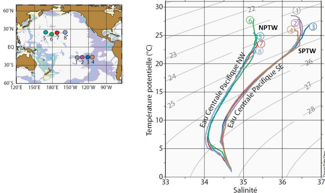
Figure IV-1. Diagrammes \theta - S de stations situées dans les deux régions où le maximum de salinité subtropical est en surface. Les stations 1 à 4 sont situées dans le gyre anticyclonique sud et les stations 5 à 8 sont situées dans le gyre anticyclonique nord. Profils issus de la base de données WOCE. [Fieux, 2010]
