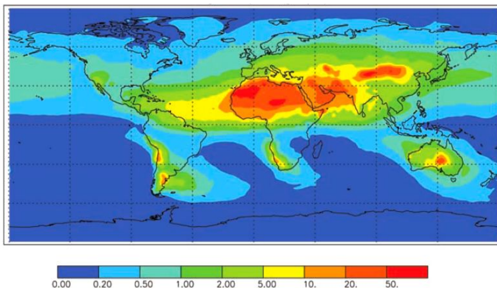
Figure II-4. Carte des flux en \text{g}/\text{m}^2/\text{an} de poussières basée sur la compilation de trois études de modélisation (elles-mêmes basées sur des observations in situ de déposition, [ Ginoux et al., 2001; Mahowald, 2003; Hand et al., 2004; Mahowald et al., 2005 ]
