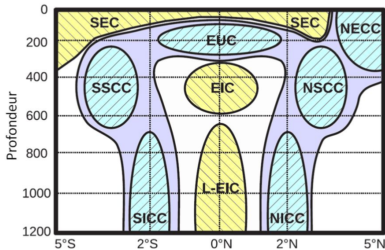
Figure III-4. Schéma de la structure du système des courants équatoriaux dans l'océan Pacifique central (165°E). Les flux d'eau colorés en bleu représentent les flux dirigés vers l'est. Ceux en bleu clair hachuré représentent les forts courants dirigés vers l'est. Ceux colorés en jaune représentent les courants dirigés vers l'ouest. EIC = Courant Equatorial Intermédiaire, L-EIC = Courant Equatorial Intermédiaire inférieur, EUC = Sous Courant Equatorial, NECC = Contre-Courant Equatorial Nord, NICC = Contre-Courant Intermédiaire Nord, NSCC = Sous-Courant Equatorial Nord, SEC = Courant Equatorial Sud, SICC = Contre-Courant Intermédiaire Sud, SSCC = Sous-Courant Equatorial Sud. [Tomczak and Godfrey, 2003; Marin et al., 2010]
