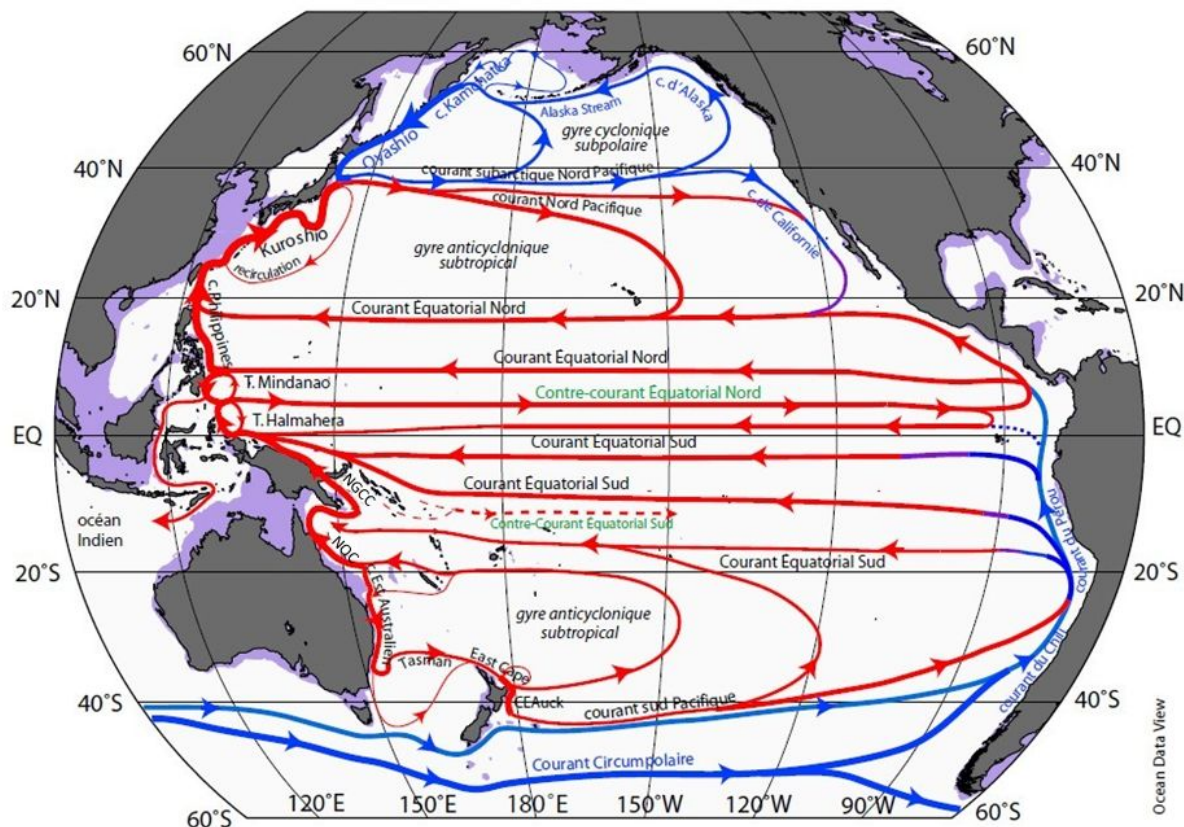
Figure III-I. Schéma de la circulation de surface de l'océan Pacifique (de mai à décembre). NGCC = Courant Côtier de Nouvelle-Guinée, CNQ = Courant du Nord Queensland, CEAuk = Courant Est Auckland, T. = tourbillon (de Mindanao et d'Halmahera). Les courants froids sont représentés en bleus et courants chauds en rouge. Les profondeurs inférieures à 250 m sont représentées en violet [Tomczak and Godfrey, 2003; Fioux, 2010].
