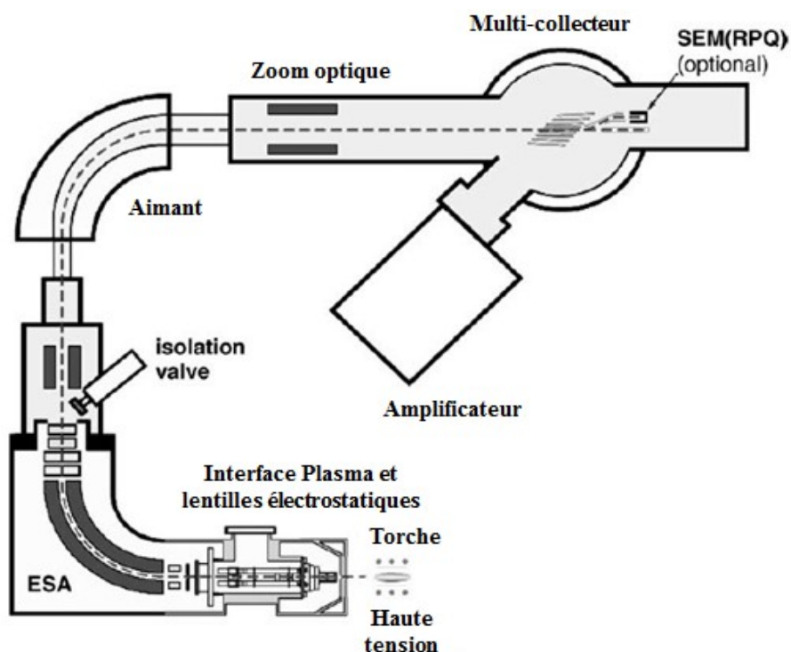
Figure III-1. Principe de fonctionnement d'un MC-IPMS ou spectromètre de masse couplé à une torche plasma et à multi-collection [Weyer and Schwieters, 2003].
