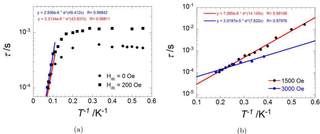
Figure 9: (a) Diagramme d'Arrhenius semi-logarithmique du temps de relaxation \tau en fonction de 1/T pour le complexe [\text{Dy}(\text{Op})_2\text{Cl}(\text{HOp})(\text{EtOH})] . La susceptibilité magnétique fut mesurée pour un champ magnétique externe nul ainsi que pour un champ statique externe de 200 Oe. La courbe obtenue par régression linéaire pour l'intervalle de température d'activation termique est tracée sur le diagramme. (b) Diagramme d'Arrhenius semi-logarithmique du temps de relaxation \tau en fonction de 1/T pour le complexe [\text{Dy}(\text{Op})_3(\text{HOp})] - [\text{Dy}(\text{Op})_3(\text{EtOH})] . La susceptibilité magnétique fut mesurée pour deux valeurs champs magnétiques externes: 1500 Oe et 3000 Oe. La courbe obtenue par régression linéaire pour l'intervalle de température d'activation termique est tracée sur le diagramme.
