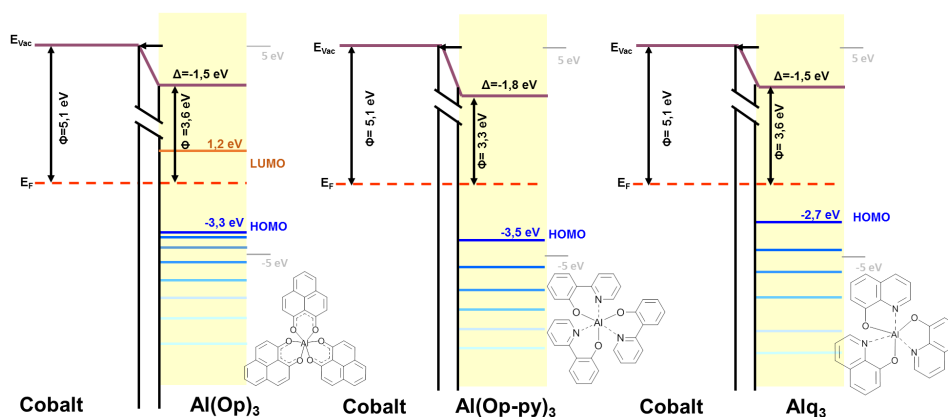
Figure 7: Alignement des niveaux d'énergie pour les interfaces \text{Co}/[5 \text{ nm}] \text{Al}(\text{Op})_3 et \text{Co}/[2.8 \text{ nm}] \text{Al}(\text{Op-py})_3 . Ces données sont extraites des spectres UPS et 2PPE. L'alignement des niveaux d'énergie pour l'interface \text{Co}/\text{Alq}_3 est indiqué à titre de comparaison.
