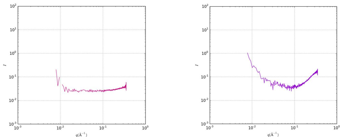
FIGURE D.4 – Diagramme SAXS de la phase organique ( \text{HMA/EGDMA} = 95/5 en masse) avant polymérisation (à gauche) et après polymérisation (à droite).
