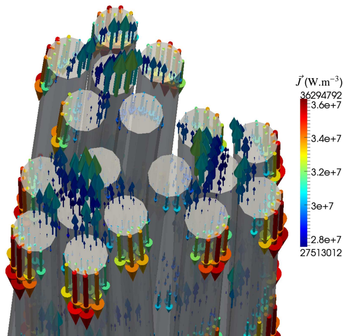
FIGURE 4.6 – Distribution de la partie réelle de la densité de courant dans l'inducteur 3\times 6 à 400 kHz (modèle volumique).
