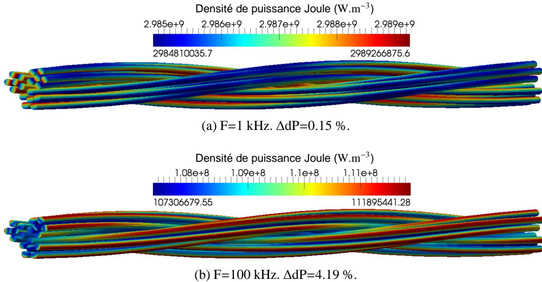
FIGURE 4.5 – Répartition locale de la densité de puissance Joule dans l'inducteur 3\times 6 à 1 kHz et 100 kHz (modèle volumique).
