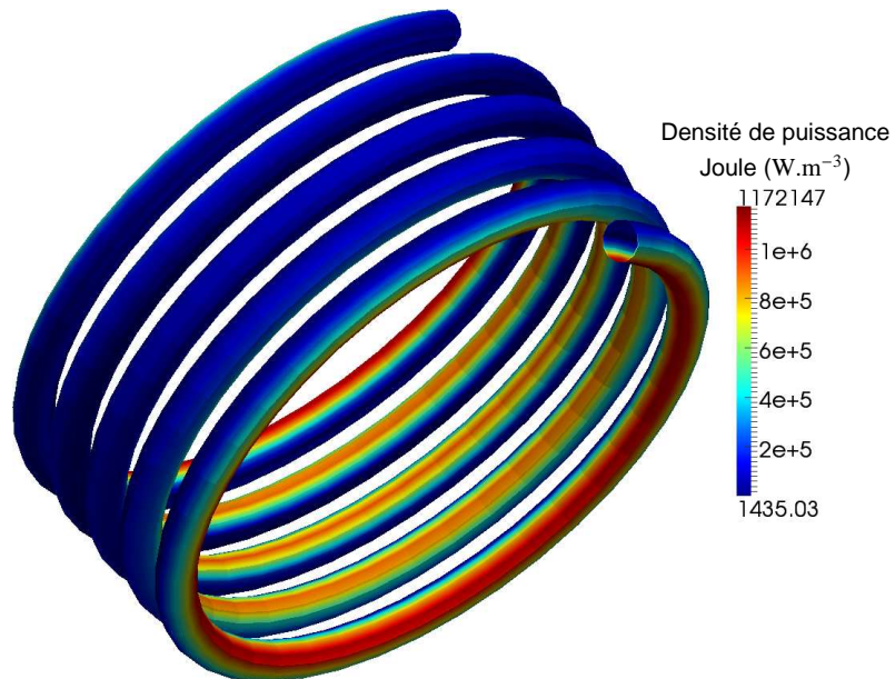
FIGURE 4.9 – Répartition de la densité de puissance dissipée par l'inducteur plein à 50 kHz.
