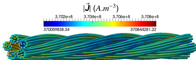
FIGURE C.5 – Répartition de la densité de courant (en module) au sein de l'inducteur.
