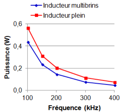
FIGURE 4.8 – Évolution de la puissance Joule dissipée dans l'inducteur 6 \times 14 \times 18 et dans l'inducteur plein en fonction de la fréquence.
