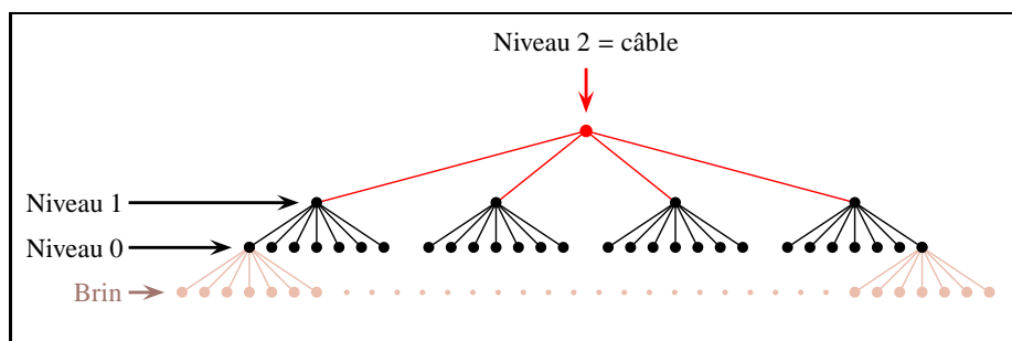
FIGURE 2.4 – Principe d'agencement des paquets et des brins pour le câble 4x7x7. Chaque paquet de niveau 0 contient sept brins.
