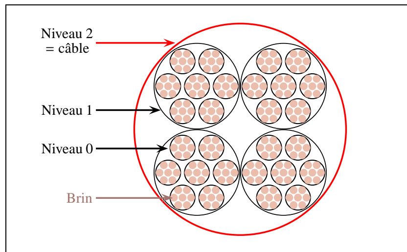
FIGURE 2.2 – Schéma en coupe de l'agencement d'un câble multibrins 4x7x7.
