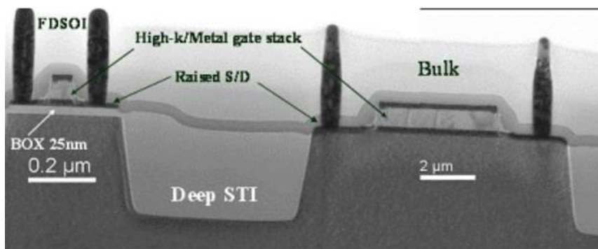
Figure 1.15 Vue en coupe d'un transistor MOS en technologie FD-SOI à BOX mince co-intégré avec un transistor BULK après ouverture du BOX [Fen'09].
