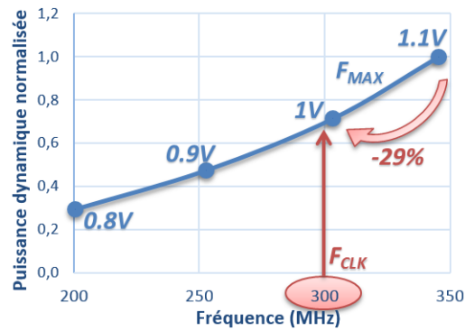
Figure 2.20 Evolution de la puissance dynamique en fonction de la fr quence par modulation de la tension d'alimentation V_{DD} .
