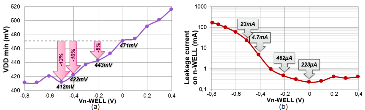
Figure 4.17 (a) Réduction de la tension d'alimentation minimale par ajustement de la polarisation du caisson-n. (b) Augmentation exponentielle du courant statique dans le caisson-n lorsque Vn-WELL est négatif.
