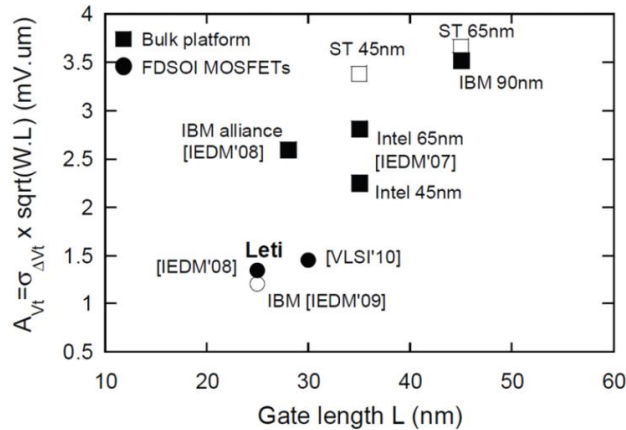
Figure 1.13 Comparaison des coefficients de Pelgrom dans différentes technologies en fonction de la longueur de grille [Fay'10].
