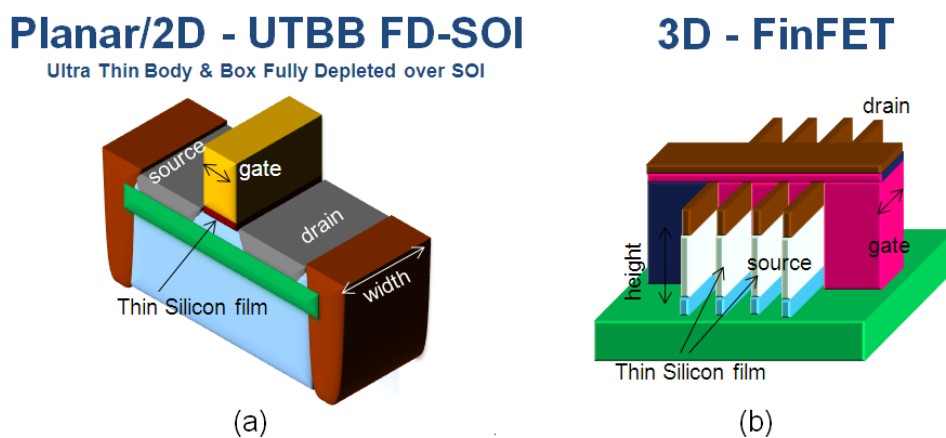
Figure 1.7 Représentation schématique d'un transistor (a) planaire FD-SOI et d'un transistor (b) 3D FinFET.
