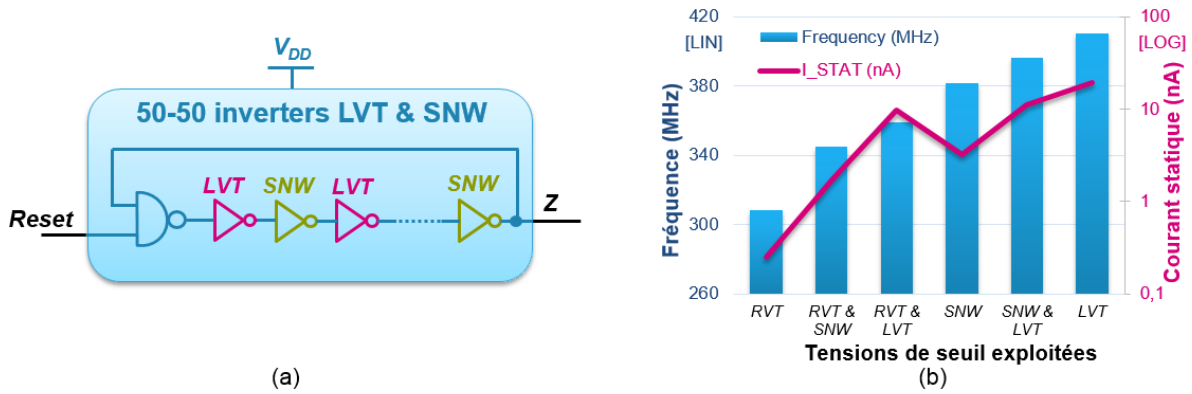
Figure 3.19 (a) Schéma de co-intégration par alternance de deux différents V T . (b) Résultats en fréquence et en courant statique à V DD =1V des circuits disposant soit d'une co-intégration de V T , soit d'un seul V T .
