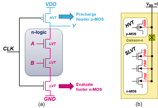
Figure 3.12 (a) Représentation d'une porte logique NAND2 intégrant une architecture de type domino logic classique. (b) Projection de l'approche domino logic sur une structure single n-Well.
