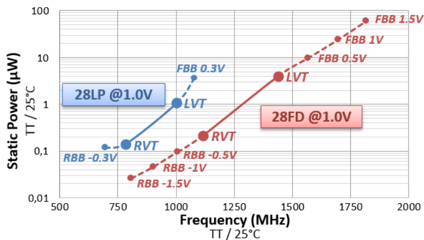
Figure 2.8 Evolution de la puissance statique en fonction de la fréquence à V_{DD}=1V , en technologie BULK et FD-SOI. En pointillé, l'extension de la gamme de performance grâce au back-biasing [-1.5 ; 1.5V].
