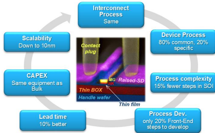
Figure 1.29 Synthèse des différences de fabrication en technologie FD-SOI en comparaison au BULK.
