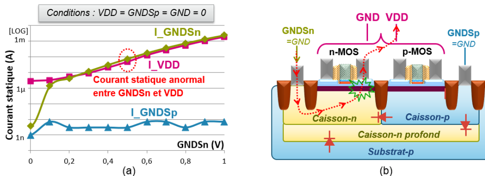
Figure 4.8 (a) Evolution des courants statiques en fonction de la tension GNDSn . (b) Représentation du courant circulant entre V_{DD} et GNDSn au sein du LDPC III.
