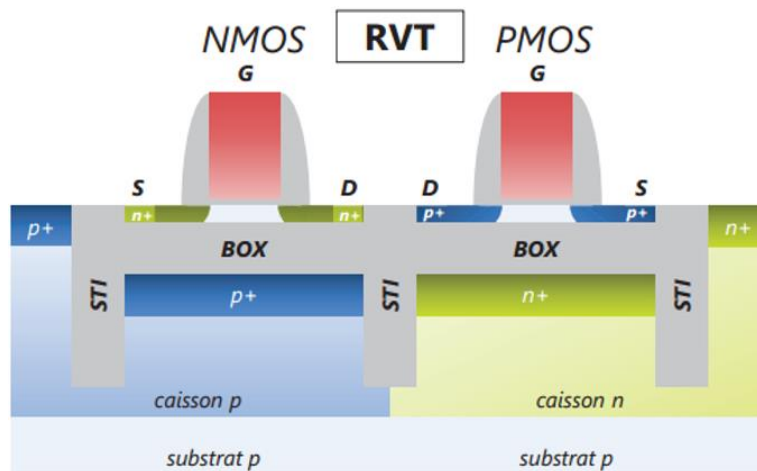
Figure 1.16 Vue schématique de deux transistors de type RVT. Un transistor n-MOS (gauche) et un p-MOS (droite).
