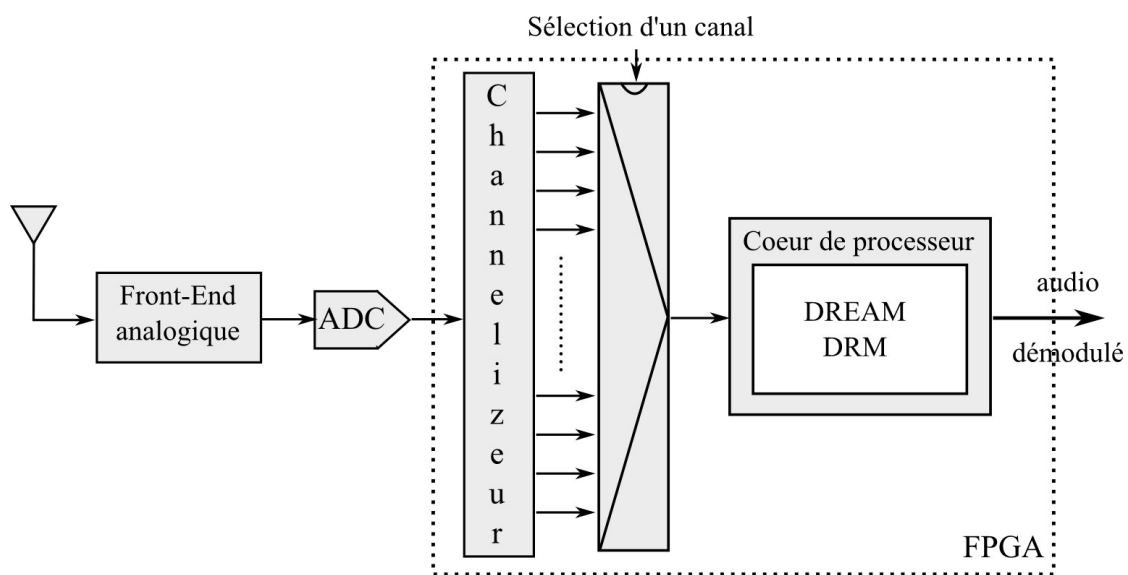
Figure 3.43 – Architecture du récepteur DRM mono-canal basé sur le logiciel Dream DRM
