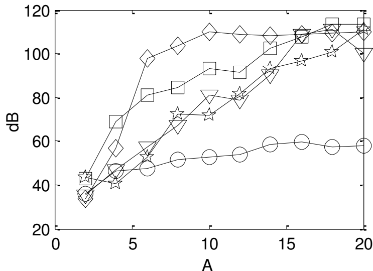
Figure 4.20 – SFDR expérimentaux obtenus pour le sur-échantillonneur lorsque A \leq 20 . O Rectangulaire, ☆ Parks-McClellan, □ Hann, ▽ Moindres carrés, ◇ Blackman Harris
