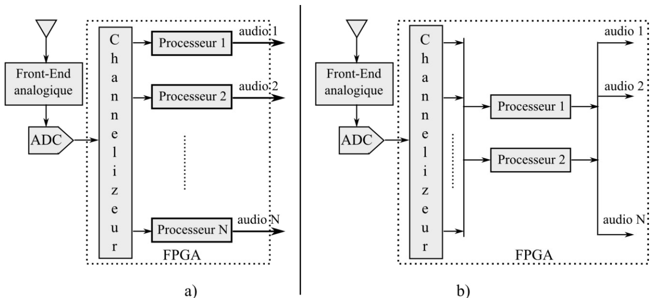
Figure 3.44 – Architecture du récepteur DRM multi-canaux basé sur le logiciel Dream DRM. a) plusieurs processeurs instanciés (un processeur par canal). b) Deux processeurs partagés en temps
