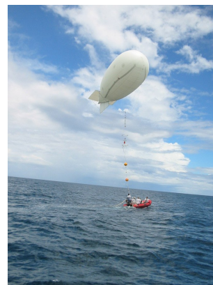
FIG. 4.3 – Aéroclipper ©CNES/LMD
