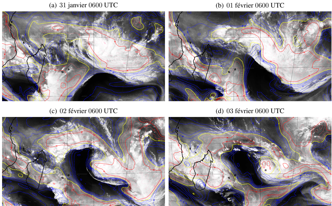
FIG. 4.9 – Humidité relative à 400 hPa (contours en %) dans les analyses ERA-Interim, superposée aux images satellitaires Météosat 7 dans le canal vapeur d'eau, du (a) 31/01/2007 à 0600 UTC au (d) 03/02/2007 à 0600 UTC par pas de 24 h. Le trait jaune délimite l'isoligne 50 % ; les valeurs inférieures sont en pointillé bleu ; les valeurs supérieures en traits roses ; l'isoligne 80 % est renforcée en rouge. Le domaine couvre la zone [2^{\circ}\text{-}32^{\circ}\text{S}] \times [35^{\circ}\text{-}95^{\circ}\text{E}] de l'océan Indien Sud.
