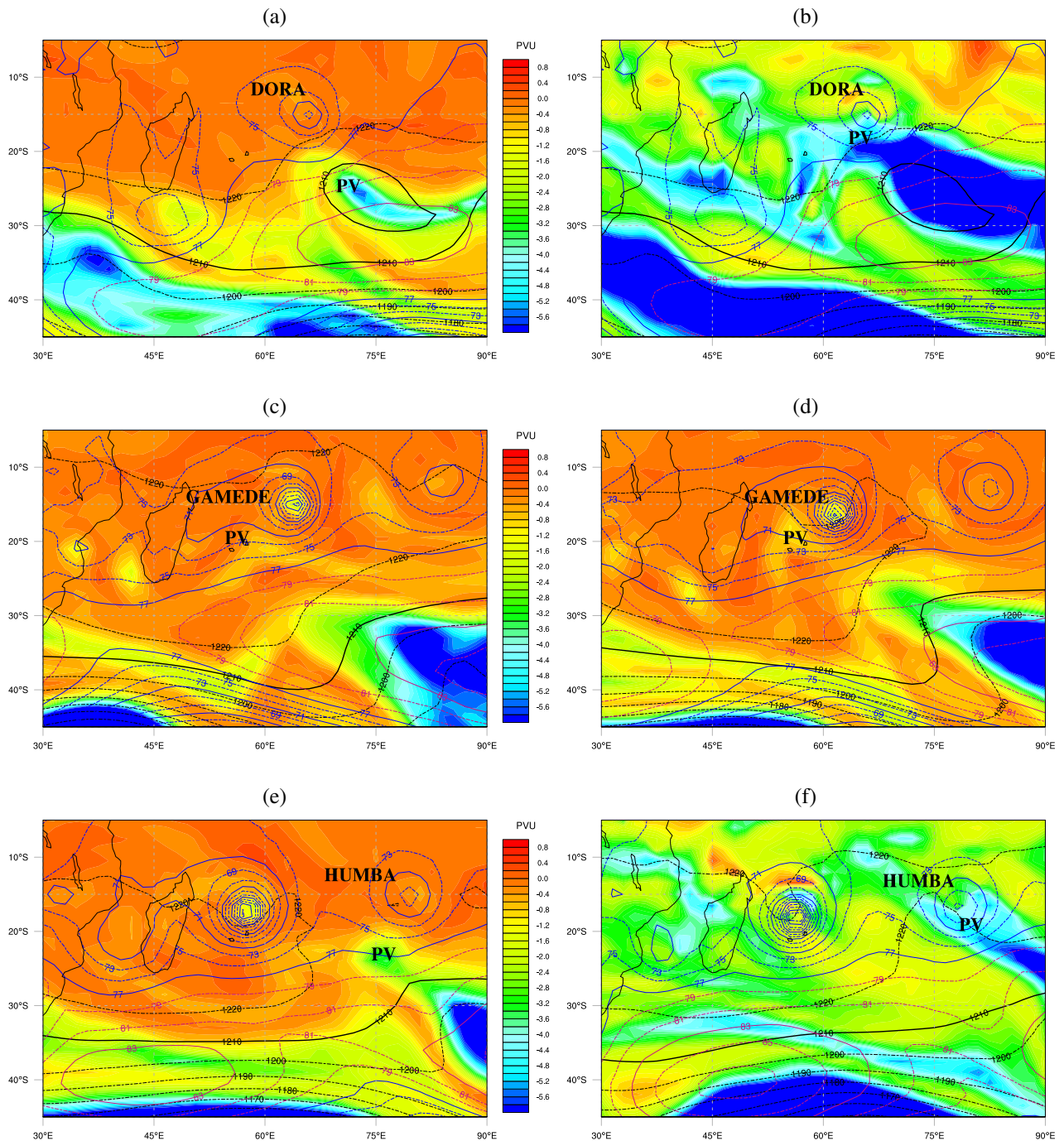
FIG. 3.13 – Similaire à la figure 3.12 mais pour des cyclones dans la configuration « possible interaction proche » en début d'intensification rapide avec, quand une signature existe, les champs de tourbillon potentiel sur la surface 370 K également. Dans l'ordre : (a) et (b) cyclone Dora le 01/02/2007 à 0000 UTC sur les isentropes 350 K et 370 K respectivement, cyclone Gamède sur l'isentrope 350 K le (c) 22/02/2007 à 1200 UTC et le (d) 23/02/2007 à 0000 UTC et cyclone Humba le 24/02/2007 à (e) 0000 UTC sur l'isentrope 350 K et à (f) 1200 UTC sur l'isentrope 370 K. Le mot « PV » désigne le déferlement (ou son résidu) qui advecte du tourbillon potentiel (PV) à proximité du cyclone. Humba est situé à l'est de Gamède dans les figures (e) à (d).
