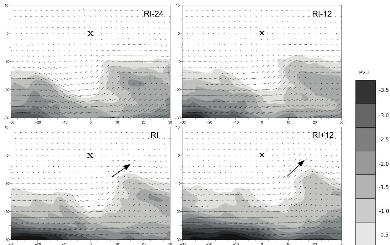
FIG. 3.11 – Cartes composites des déferlements en classe 3, lorsque le thalweg est situé au sud-est du centre cyclonique au moment de l'intensification ( t=RI ). Même légende qu'en figure 3.9.
