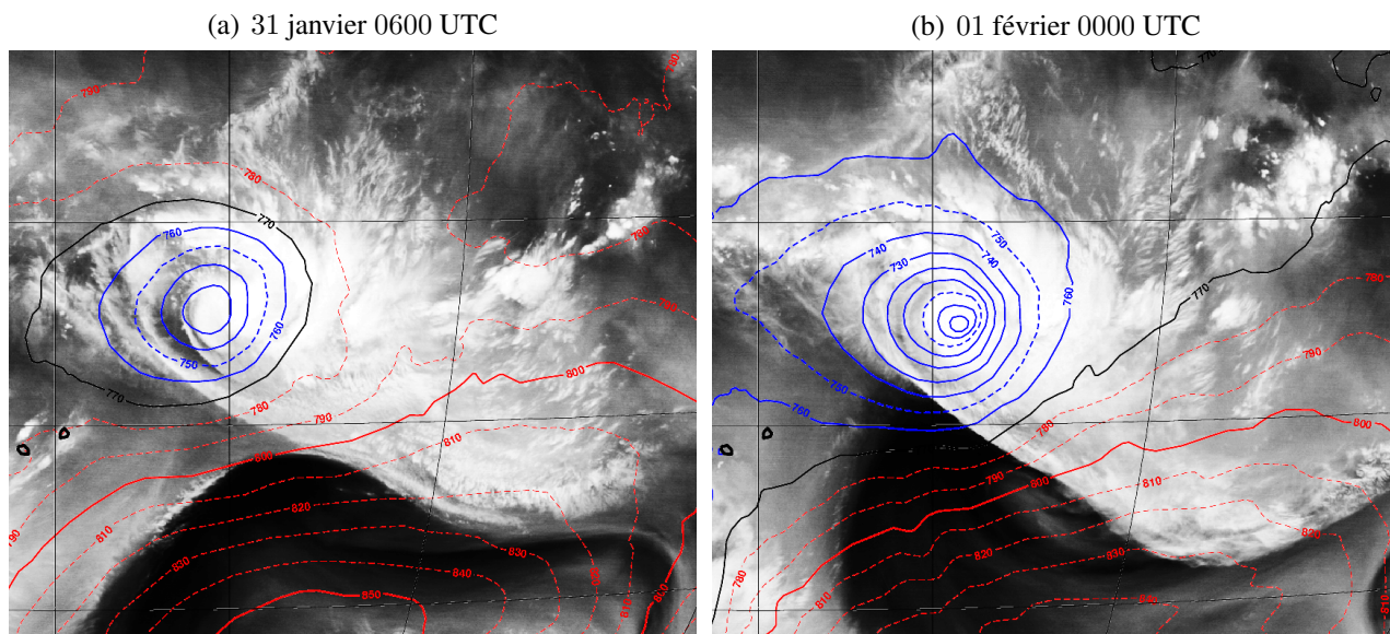
FIG. 4.13 – Similaire à la Fig. 4.10 mais pour le champ de géopotentiel à 925 hPa (contours en mgp) dans les analyses opérationnelles IFS du (a) 31/01/2007 à 0600 UTC et du (b) 01/02/2007 à 0000 UTC. Le trait noir marque l'isoligne 770 mgp ; les valeurs inférieures (zone dépressionnaire) sont tracées en bleu par pas de 10 mgp ; les valeurs supérieures (zone anticyclonique) sont tracées en rouge par pas de 10 mgp.
