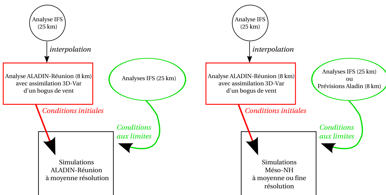
FIG. 4.15 – Schémas récapitulant la stratégie de modélisation pour les deux modèles de simulation ALADIN-Réunion (à gauche) et Méso-NH (à droite). L'état initial apparaît en rouge et le(s) modèle(s) coupleur en vert.
