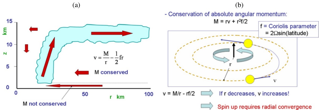
FIG. 2.10 – (a) Conservation du moment angulaire absolu M au-dessus de la couche limite. (b) Implication pour un fluide non visqueux : augmentation du vent tangentiel en présence d'un flux radial convergent (principe de spin-up). Source : figure 2 et 4 de Montgomery et Smith (2011).
