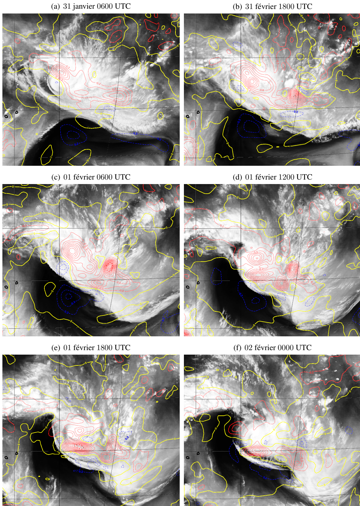
FIG. 4.12 – Similaire à la figure 4.10 mais pour le champ de vitesse verticale à 500 hPa (contours en \text{Pa.s}^{-1} ) du (a) 31/01/2007 à 0600 UTC au (f) 02/02/2007 à 0000 UTC, aux dates précisées en haut de chaque figure. Le contour de vitesse nulle est de couleur jaune ; les subsidences (omega positif) sont indiquées en trait pointillé bleu par pas de 0,2 \text{ Pa.s}^{-1} ; les ascendances (omega négatif) sont tracées en rose par pas de 0,2 \text{ Pa.s}^{-1} , avec le contour -2 \text{ Pa.s}^{-1} renforcé par un trait pointillé rouge.
