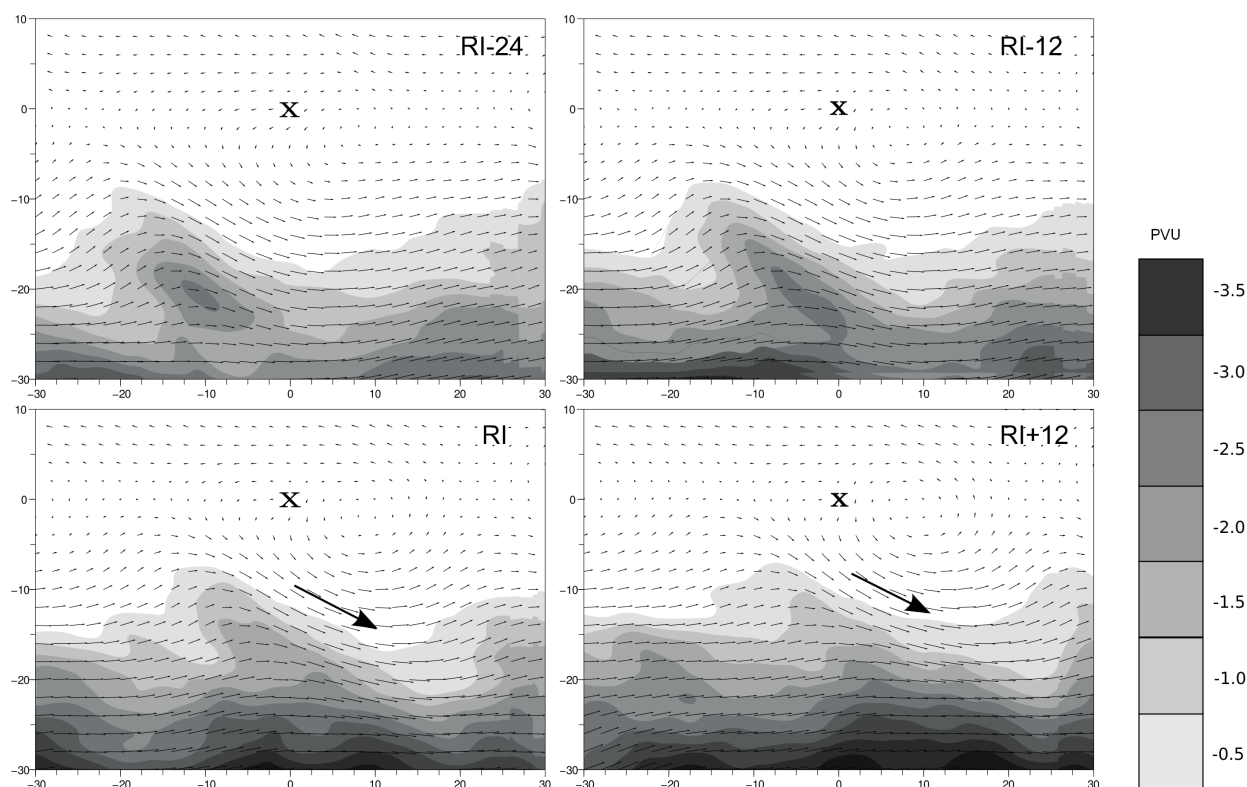
FIG. 3.9 – Cartes composites des déferlements en classe 1, lorsque le thalweg est situé au sud-ouest du centre cyclonique au moment de l'intensification. Le centre du cyclone composite est localisé en (0,0) et matérialisé par une croix. Abscisse et ordonnée sont les distances relatives au centre cyclonique mesurées en degrés de longitude et latitude. Le champ de tourbillon potentiel sur la 200 hPa est en couleurs grisées (échelle à droite, en unité de PVU) et les vents à 200 hPa sont indiqués par des flèches. Les cartes sont affichées à différents instants entourant le début de la phase d'intensification rapide : 24 h avant (RI-24), 12 h avant (RI-12), à l'instant initial d'intensification (RI) et 12 h après (RI+12). La grande flèche noire matérialise le renforcement du canal d'évacuation côté polaire du cyclone par le thalweg d'altitude.
