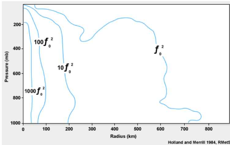
FIG. 2.11 – Distribution verticale et radiale de la stabilité inertielle au sein d'un cyclone tropical type. Les valeurs sont exprimées en fonction de la valeur de référence f_0 \sim 10^{-5} s^{-1} valable dans un cyclone. Source : figure 6a de Holland et Merrill (1984) .
