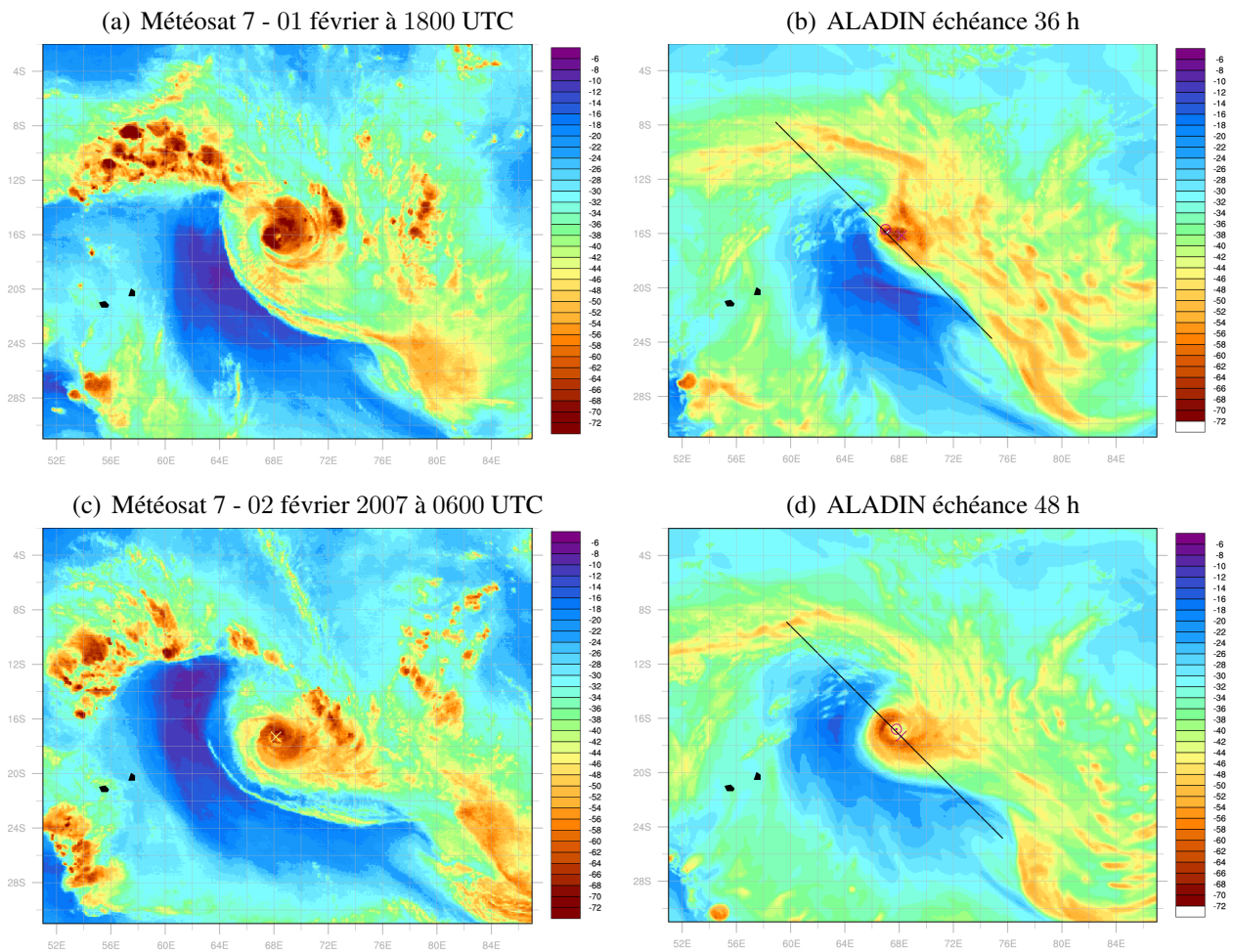
FIG. 4.24 – Températures de brillance dans le canal vapeur d’eau observées par Météosat 7 (à gauche), ou simulées par ALADIN -Réunion (à droite) obtenues par le modèle de transfert radiatif RTTOV , pour les dates du 01 février à 1800 UTC (échéance 36 h) et du 02 février 2007 à 0600 UTC (échéance 48 h). La palette de couleurs du canal vapeur d’eau de Météosat 7 a été reproduite pour tracer les images satellitaires simulées ; le domaine est identique et les lignes sont quadrillées tous les 2° de latitude-longitude.
