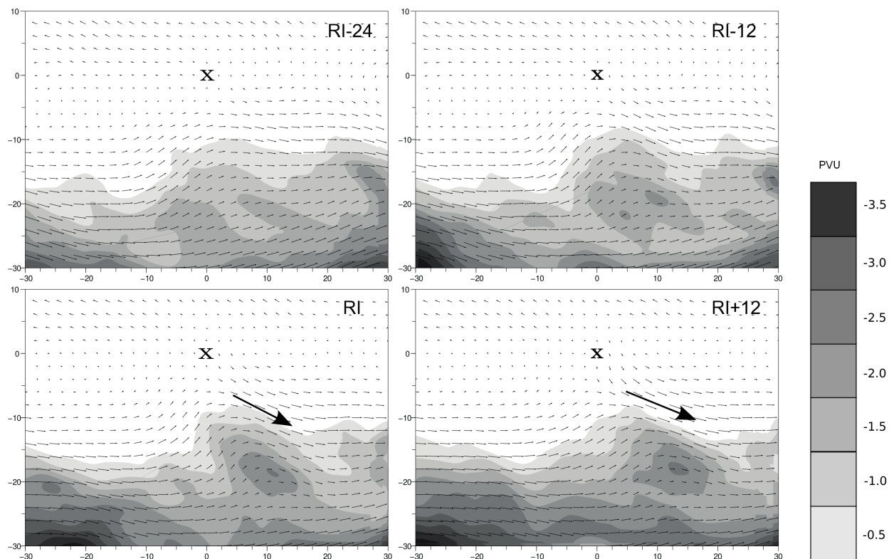
FIG. 3.10 – Cartes composites des déferlements en classe 2, lorsque le thalweg est situé au sud du centre cyclonique au moment de l'intensification ( t=RI ). Même légende qu'en figure 3.9.
