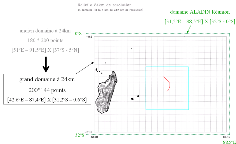
FIG. A.2 – Domaines retenus pour les différentes simulations MésO-NH . En haut sont représentés les domaines des simulations emboîtées à 24 et 12 km de résolution, ainsi que les domaines des simulations à une seule grille de 8 ou 4 km de résolution, accompagnés de leur nombre de points de grille respectifs. Les domaines étendus, nommés 8kBIG et 24kBIG, à 8 km et 24 km de résolution figurent respectivement au milieu et en bas. La trajectoire du système Dora est tracée en rouge sur la période 31 janvier 1200 UTC - 03 février 1200 UTC (données Best track toutes les 6 h).
