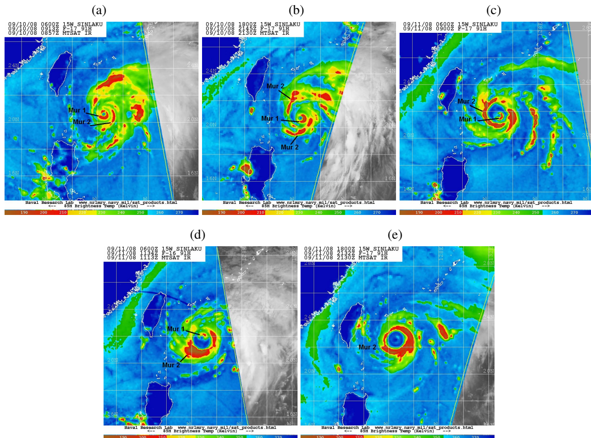
FIG. 2.19 – Exemple de changement de structure observé par satellite défilant : le cycle de remplacement du mur de l'œil, pour lequel un mur externe (mur 2) se développe autour du mur originel (mur 1) qui finit par s'effondrer. Les températures de brillance dans le canal micro-ondes sont illustrées pour le typhon Sinlaku autour des instants : (a) 0900 UTC et (b) 2130 UTC le 10 septembre, (c) 0900 UTC, (d) 1130 UTC et (e) 2130 UTC le 11 septembre 2008. La grille est tracée tous les 2° de latitude-longitude. Source : images du Naval Research Laboratory (NRL) : http : //www.nrlmry.navy.mil/tc_pages/tc_home.html
