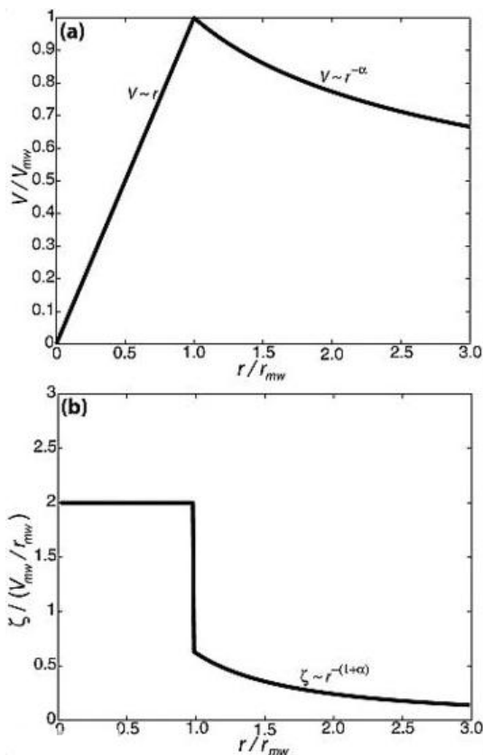
FIG. 2.12 – Profil radial (a) du vent tangential et (b) du tourbillon relatif dans un vortex de Rankine modifié. Le paramètre \alpha représente la décroissance non linéaire du vent tangential au delà du RVM, noté r_{mw} (pour « radius of maximum wind »). \alpha = 0,4 pour l'illustration. Le rayon en abscisse est normalisé par r_{mw} . Le vent est normalisé par sa valeur maximale notée V_{mw} (a) et le tourbillon est normalisé par la quantité V_{mw}/r_{mw} (b). Source : figure 1 de Swanson (2008).
