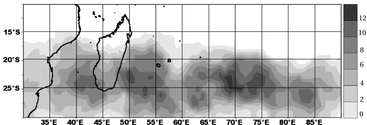
FIG. 3.7 – Densité des déferlements d'onde de Rossby à 200 hPa situés à proximité de cyclones en début d'intensification rapide entre 1989 et 2009 (bassin SOOI ). Les contours indiquent le nombre de déferlements qui sont comptabilisés par carré de 2^\circ \times 2^\circ , de 0 (blanc) à 14 (gris foncé).
