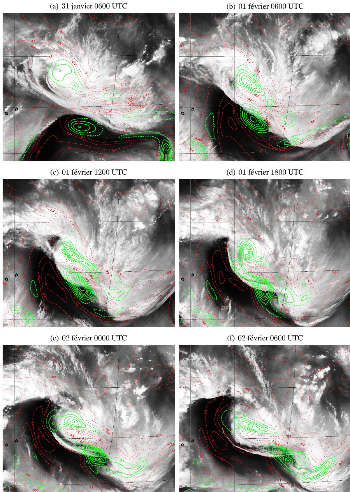
FIG. 4.10 – Similaire à la figure 4.9 mais pour le champ de tourbillon potentiel à 400 hPa (contours en PVU) du (a) 31/01/2007 à 0600 UTC au (f) 02/02/2007 à 0600 UTC, aux dates précisées en haut de chaque figure avec un domaine rogné à 55°E à l'ouest. Les isolignes -0,4 PVU, -0,2 PVU et 0 PVU sont dessinées en trait pointillé rouge ; les valeurs inférieures ou égales à -0,7 PVU sont tracées en vert par pas de 0,3 PVU avec des pointillés toutes les 4 isolignes ( -0,7 PVU et -1,9 PVU).
