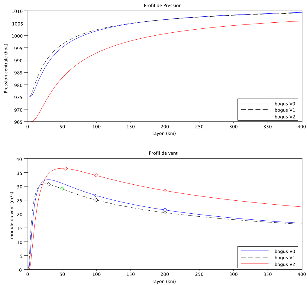
FIG. 4.18 – Profils radiaux de pression et de vent en surface le 31 janvier 2007 à 0600 UTC pour les bogus retenus V0, V1 (ou Vf), et V2, selon la formule de Holland (1980) . Le rayon varie jusque 400 km en abscisse. Les losanges sur les courbes indiquent les rayons où sont assimilées les pseudo-observations de vent extraites de ces profils. Le losange vert sur la courbe noire (bogus V1) correspond au cercle d'assimilation supplémentaire ajouté pour le bogus Vf.
