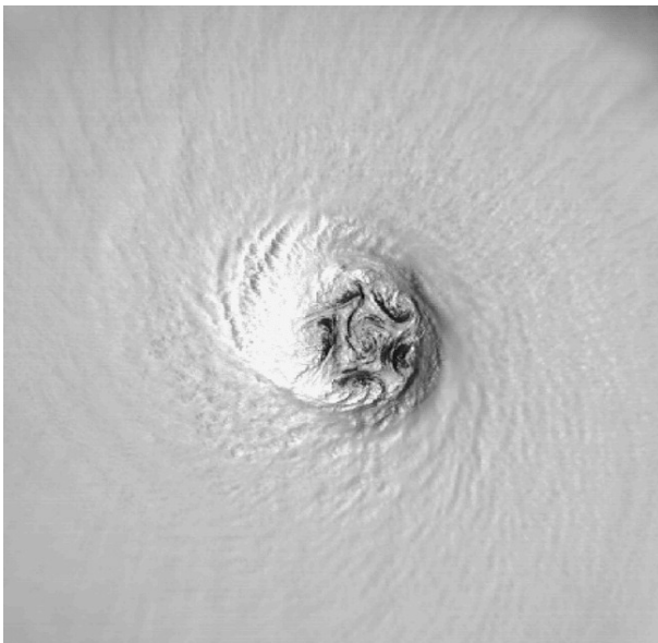
FIG. 2.17 – Image visible du satellite DMSP (F15) dans le cœur de l'ouragan Isabel le 12 Septembre 2003 à 1315 UTC (pression centrale d'environ 930 hPa, vents max de 70\text{ m.s}^{-1} , RVM de 32 km). La forme pentagonale de l'œil en allure d'étoile de mer est due à la présence de 5 méso-vortex arrangés symétriquement autour d'un méso-vortex central, le tout en rotation cyclonique. Dimensions approximatives du domaine : 200\text{ km} \times 200\text{ km} . Source : figure 10 de Rozoff et al. (2006) .
