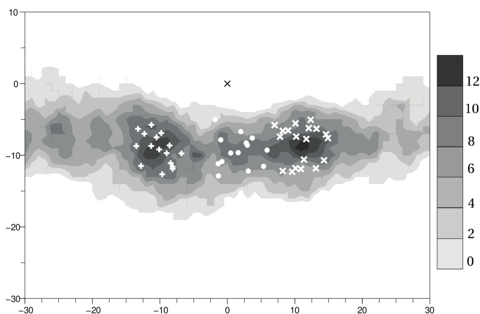
FIG. 3.8 – Composite de la densité des déferlements d'onde de Rossby autour du centre cyclonique à l'instant initial d'intensification rapide. Le centre du cyclone composite est localisé en (0,0) et matérialisé par une croix. Abscisse et ordonnée sont les distances relatives au centre cyclonique mesurées en degrés de longitude et latitude. Les contours indiquent le nombre de déferlements comptabilisés par carré de 2^\circ \times 2^\circ , de 0 (blanc) à 14 (gris foncé). Les différents symboles blancs matérialisent les centres des déferlements dans chacune des 3 classes identifiées (symbole + pour un thalweg au sud-ouest, ● au sud, × au sud-est).
