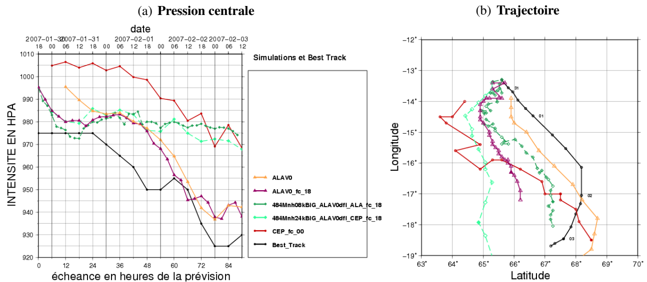
FIG. A.5 – Prévission de (a) la pression centrale (en hPa) de Dora et (b) la trajectoire de Dora, pour diverses simulations numériques figurant en légende, initialisées à divers réseaux entre le 30 janvier 1800 UTC et le 31 janvier 2007 0600 UTC. En noir la Best track ; en rouge foncé la prévission opérationnelle IFS de 2007 pour le réseau 0000 UTC du 31 janvier 2007; en orange la prévission ALADIN avec le bogus V0 spécifié par les observations en temps réel du réseau 0600 UTC le 31 janvier; en mauve la prévission ALADIN avec le même type de bogus (V0) mais au réseau 1800 UTC le 30 janvier; en vert foncé pointillé la simulation Més0-NH à 8 km de résolution, sur un grand domaine, initialisée par l'analyse ALADIN précédente avec bogus V0 (courbe mauve) et couplée aux analyses IFS ; en vert clair pointillé la simulation Més0-NH à 24 km de résolution, sur un grand domaine, initialisée par la même analyse ALADIN et couplée à la prévission correspondante (courbe mauve).
