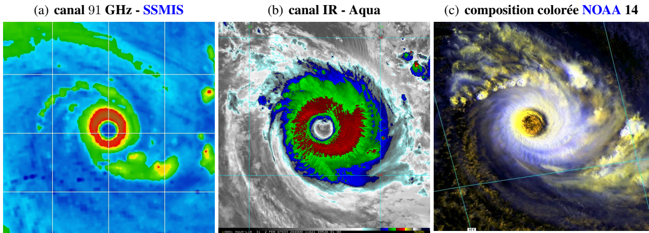
FIG. 2.18 – Structure annulaire de Dora capturée par divers satellites et canaux explicités en légende. (a) image micro-ondes du capteur SSMIS le 02 février à 1600 UTC ; (b) image IR colorée de l'instrument MODIS sur Aqua le 02 février à 2040 UTC ; (c) composition colorée du satellite NOAA 14 le 03 février à 0500 UTC. Les domaines varient mais la grille est tracée tous les 2° (a) et 5° (b,c).
