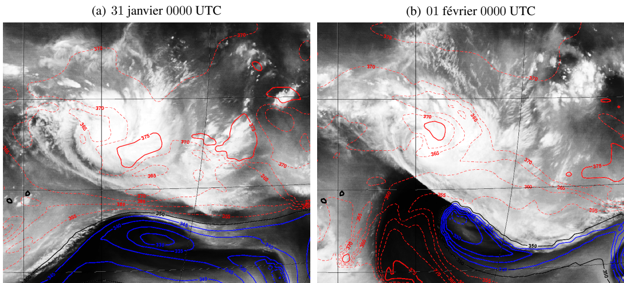
FIG. 4.11 – Similaire à la Fig. 4.10 mais pour le champ de température potentielle \Theta sur la surface -2 PVU (contours en K) le (a) 31/01/2007 à 0000 UTC et le (b) 01/02/2007 à 0000 UTC. Les isolignes sont tracées par pas de 5 K ; en noir la 350 K ; en trait plein bleu les valeurs inférieures, avec des pointillés pour la 325 K ; en pointillés rouges les valeurs supérieures, avec un trait continu pour la 375 K.
