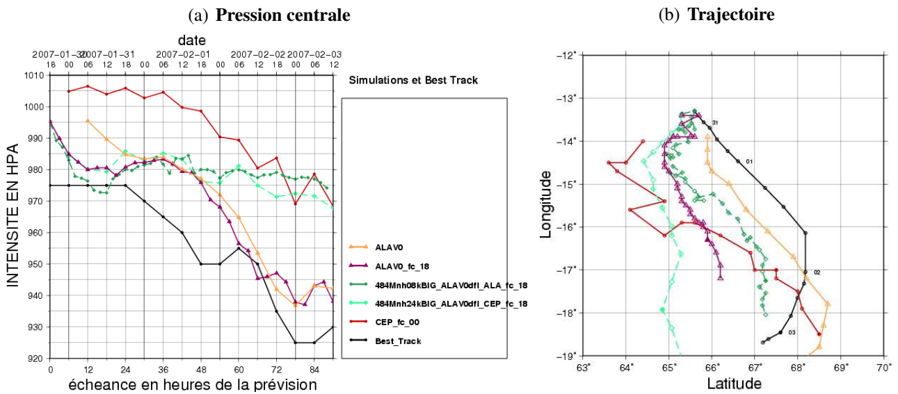
FIG. A.5 – Prédiction de (a) la pression centrale (en hPa) de Dora et (b) la trajectoire de Dora, pour diverses simulations numériques figurant en légende, initialisées à divers réseaux entre le 30 janvier 1800 UTC et le 31 janvier 2007 0600 UTC. En noir la Best track ; en rouge foncé la prédiction opérationnelle IFS de 2007 pour le réseau 0000 UTC du 31 janvier 2007; en orange la prédiction ALADIN avec le bogus V0 spécifié par les observations en temps réel du réseau 0600 UTC le 31 janvier; en mauve la prédiction ALADIN avec le même type de bogus ( V0 ) mais au réseau 1800 UTC le 30 janvier; en vert foncé pointillé la simulation Més0-NH à 8 km de résolution, sur un grand domaine, initialisée par l'analyse ALADIN précédente avec bogus V0 (courbe mauve) et couplée aux analyses IFS ; en vert clair pointillé la simulation Més0-NH à 24 km de résolution, sur un grand domaine, initialisée par la même analyse ALADIN et couplée à la prédiction correspondante (courbe mauve).
