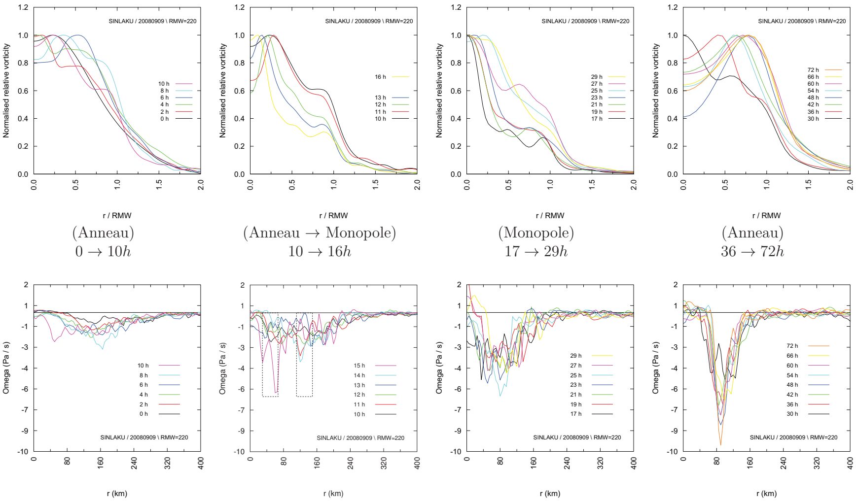
FIG. 6.1 – Evolution des profils radiaux du tourbillon relatif moyen normalisé ( s^{-1} , graphiques du haut) et de la vitesse verticale moyenne ( Pa \cdot s^{-1} , en bas) dans la couche limite, au cours de la prévision à 5 km de résolution du typhon Sinlaku initialisée par un RVM de 220 km (SS18). Les deux rectangles pointillés sur le deuxième panneau du bas indiquent les zones d'ascendances principales (murs de l'œil) qui fusionnent ensuite.
