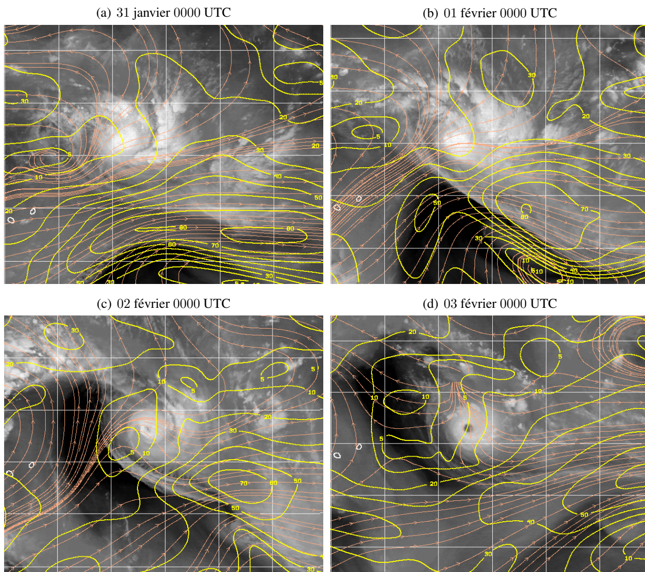
FIG. 4.2 – Amplitude du cisaillement vertical de vent (contours jaunes, en nœuds) dans l’océan Indien Sud superposé aux images satellitaires Météosat 7 dans le canal vapeur d’eau, du (a) 31/01/2007 à 0000 UTC au (d) 03/02/2007 à 0000 UTC, par pas de 24 h. Ces analyses sont produites par le CIMSS à partir des vecteurs déplacements atmosphériques déduits des observations satellitaires. Le vecteur cisaillement est déterminé en calculant, pour chaque composante zonale et méridienne du vent, la différence de la valeur moyenne du vent sur une couche mince de haute troposphère (niveaux 150, 200, 250, et 300 hPa) et de basse troposphère (niveaux 700, 775, 850, et 925 hPa). Les lignes de flux (en orange) indiquent la direction du cisaillement. Le domaine est maintenu constant en longitude et s’étend sur [55^{\circ}-85^{\circ}E] avec les îles Maurice et Réunion à l’extrême gauche ; il couvre 25^{\circ} de latitude mais ses bornes sont variables pour suivre la progression du système vers le sud ; le parallèle 20^{\circ}S se trouve juste au nord des 2 îles. La grille est tracée tous les 5^{\circ} de latitude-longitude.
