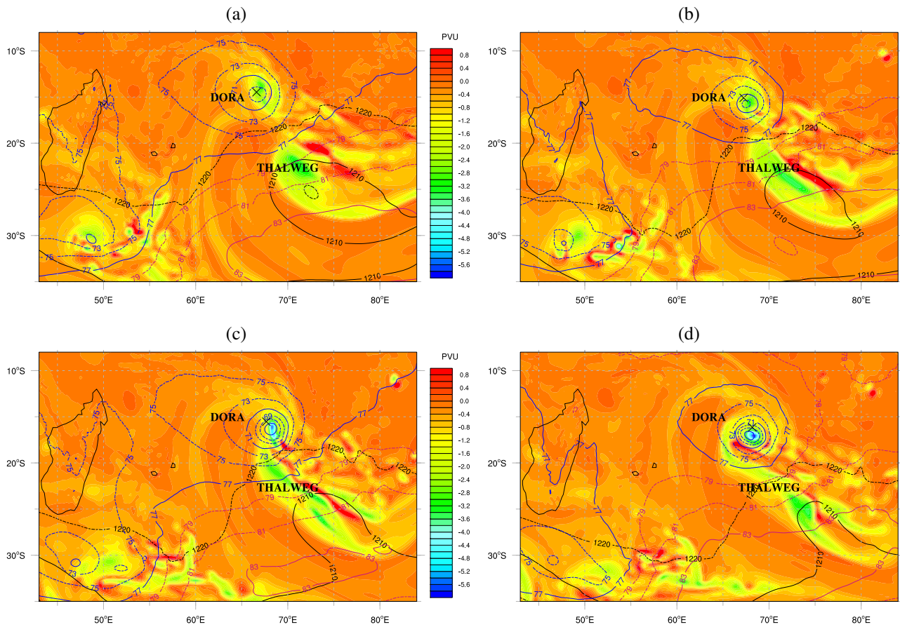
FIG. 4.7 – Similaire à la Fig. 3.12 mais pour les analyses opérationnelles du CEPMMT à 25 km de résolution sur l'isentrope 330 K, durant la 1 ère phase d'intensification rapide de Dora : du (a) 01/02/2007 à 0000 UTC au (d) 01/02/2007 à 1800 UTC, par pas de 6 heures. La croix représente la position du minimum dépressionnaire de surface selon la Best track .
