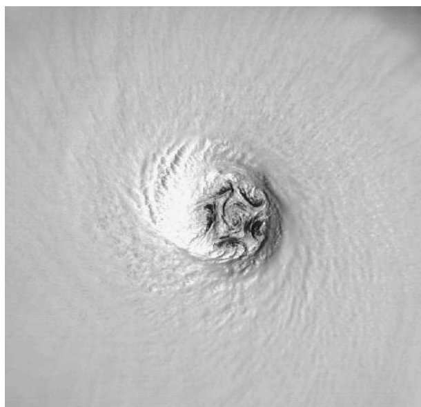
FIG. 2.17 – Image visible du satellite DMSP (F15) dans le cœur de l'ouragan Isabel le 12 Septembre 2003 à 1315 UTC (pression centrale d'environ 930 hPa, vents max de 70\text{ m.s}^{-1} , RVM de 32 km). La forme pentagonale de l'œil en allure d'étoile de mer est due à la présence de 5 méso-vortex arrangés symétriquement autour d'un méso-vortex central, le tout en rotation cyclonique. Dimensions approximatives du domaine : 200\text{ km} \times 200\text{ km} . Source : figure 10 de Rozoff et al. (2006).
