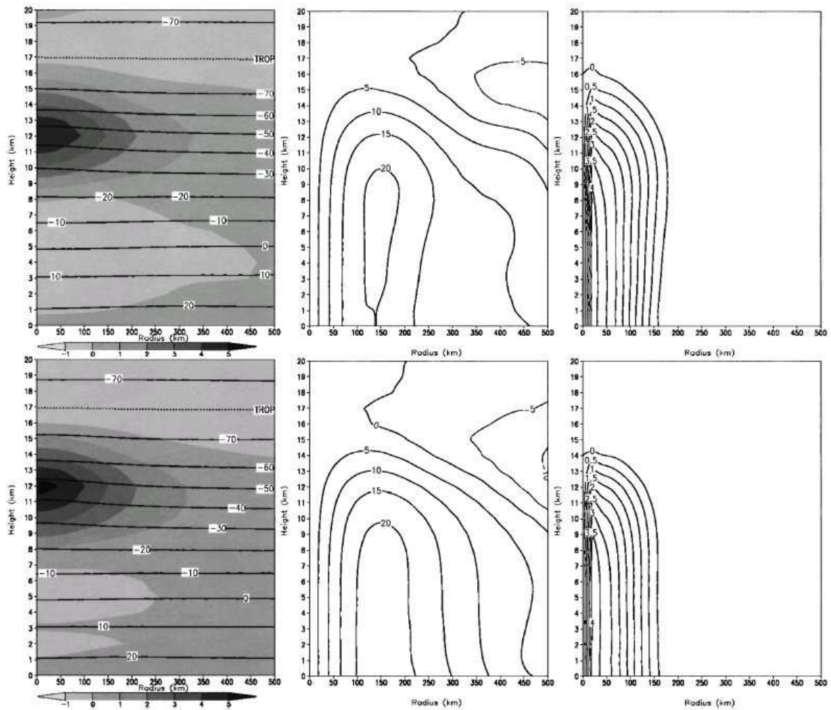
FIG. 2.28 – Coupes verticales composites obtenues à partir de cyclones d'intensité comprise entre 46 et 52 m.s -1 évoluant dans des cisaillements de vent inférieur (haut) ou supérieur (bas) à 7,5 m.s -1 ; à gauche les températures (contours en °C) et anomalies de température (zones grises en °C, le cœur chaud apparaît en noir) ; au milieu le vent tangential moyen (contours en m.s -1 ) ; à droite le tourbillon vertical (10 -4 s -1 ). Source : figure 5 de Knaff et al. (2004).
