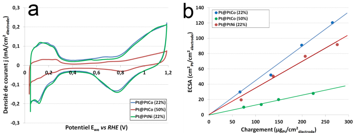
Figure 89 : (a) Voltampérogrammes sous \text{N}_2 des particules Pt@PtM à 250 \mu\text{g}_{\text{métal}}/\text{cm}^2 et 1 mV/s; (b) Evolution de la surface active ECSA en fonction du chargement en platine à 5 mV/s ( \text{H}_2\text{SO}_4 0,5M, \text{N}_2 )
