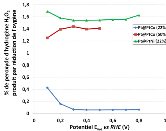
Figure 93 : Evolution du pourcentage de peroxyde d'hydrogène produit par la réduction de l'oxygène en fonction du potentiel ( 1\text{mV/s} ; 900\text{rpm} ; 250\mu\text{g}_{\text{métal}}/\text{cm}^2 ; \text{H}_2\text{SO}_4\ 0,5\text{M} ; \text{O}_2 )
