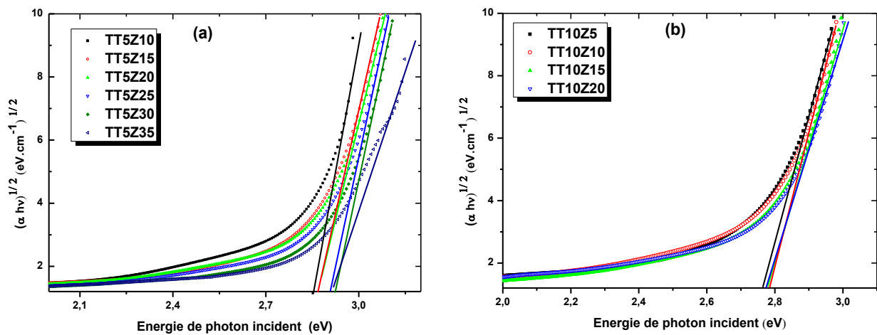
Figure V- 7. Détermination du gap en énergie à partir de la variation de (\alpha hv)^{1/2} en fonction de hv pour les verres TT5Zy (a) et TT10Zy' (b) pour différentes concentrations en ZnO .
