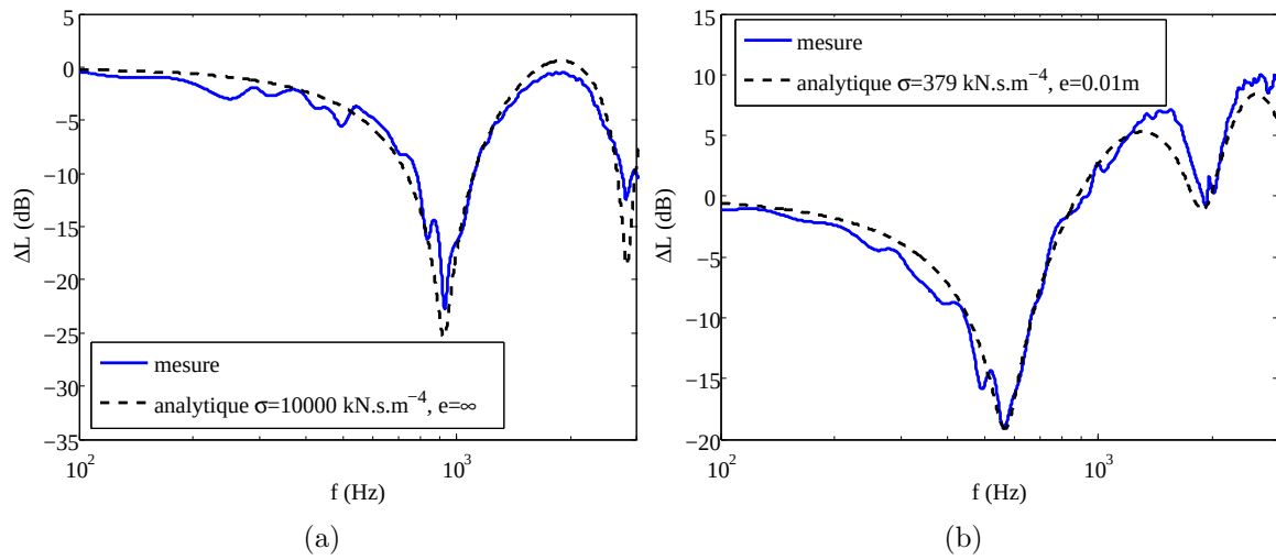
FIGURE 3.8 – Estimation des paramètres d'impédance des plaques planes à pleine échelle. (a) Surface enduite de résine époxy ; (b) Surface enduite de résine époxy et recouverte de feutrine.
