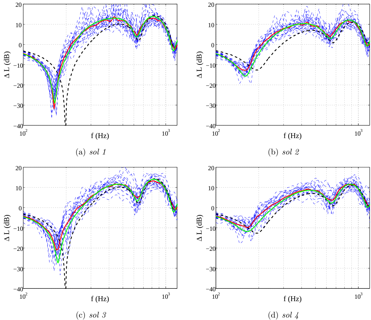
FIGURE 4.8 – Spectres d'atténuation \Delta L à une distance de 50 m au-dessus de 20 réalisations du différents types de sol. (—) Résultats TLM (—) Résultat TLM moyen; (—) Solution analytique avec impédance effective (modèle MPP); (—) Solution analytique pour le sol plat absorbant.
