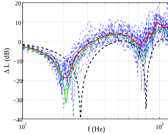
FIGURE 4.7 – Spectres d’atténuation \Delta L à une distance de 50 m au-dessus de 20 réalisations d’un profil rugueux réfléchissant au spectre de rugosité gaussien ( \sigma_h = 0.05 m, l_c = 0.2 m). (–) Résultats TLM; (—) Résultat TLM moyen; (—) Solution analytique avec impédance effective (modèle MPP); (–) Solution analytique pour le profil plat réfléchissant.
