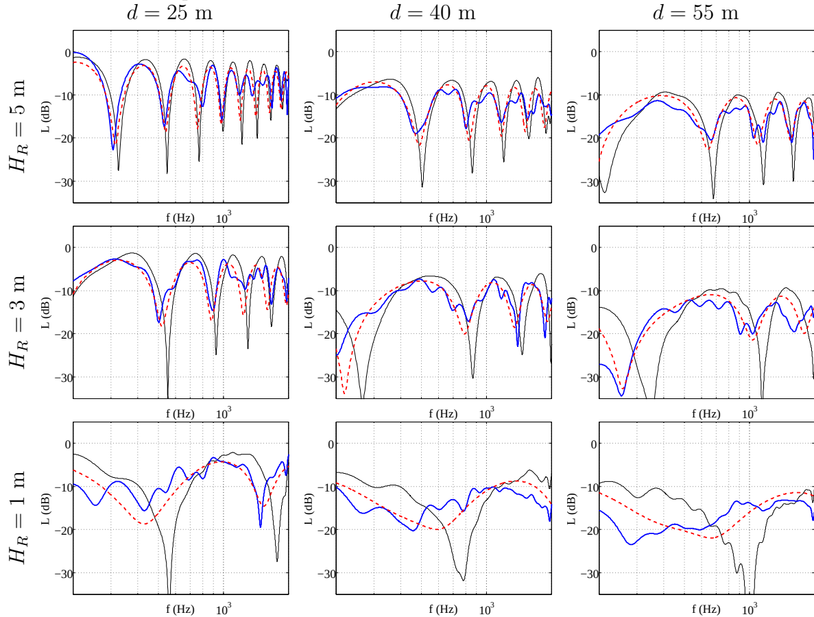
FIGURE C.6 – Niveaux de pression à différentes positions au-dessus des surfaces réfléchissantes pour H_S = 4 m : (—) mesure au-dessus de la surface plane, (—) mesure au-dessus de la surface rugueuse, (- -) solution analytique avec impédance effective.
