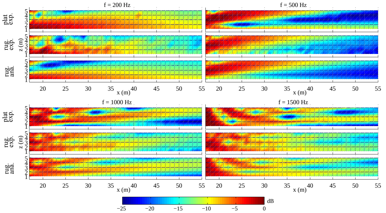
FIGURE 3.13 – Source située à H_S = 2 m au-dessus des surfaces réfléchissantes, cargographies : (haut) des niveaux de pression acoustique mesurés au-dessus de la surface plane, (centre) des niveaux mesurés au-dessus de la surface rugueuse, (bas) du résultat analytique avec le modèle d'impédance effective.
