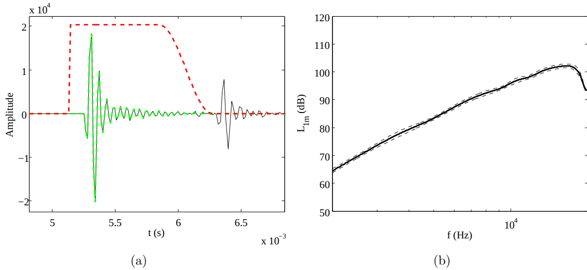
FIGURE 3.9 – (a) Fenêtrage des réponses impulsionnelles pour ne garder que le signal direct : (—) fenêtrage, (—) signal brut, (—) signal direct fenêtré ; (b) Estimation du niveau de pression en champ libre à 1 m : (—) valeur moyenne, (—) valeur moyenne \pm un écart-type.
