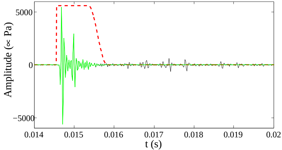
FIGURE 3.10 – Fenêtrage des signaux pour supprimer les réflexions parasites : (—) fenêtré, (—) signal brut, (—) signal fenêtré.
