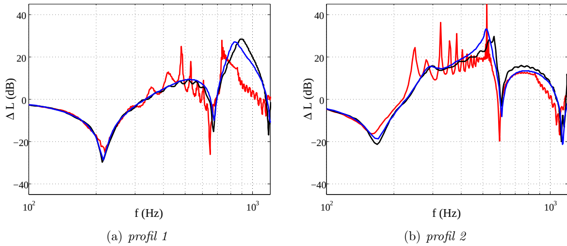
FIGURE 4.5 – Spectres d'atténuations \Delta L obtenus par simulations FDTD et TLM avec impédance effective. (—) Résultat FDTD ; (—) Résultat TLM ; (—) Résultat FDTD obtenu en 4.1.1 avec maillage des diffuseurs.
