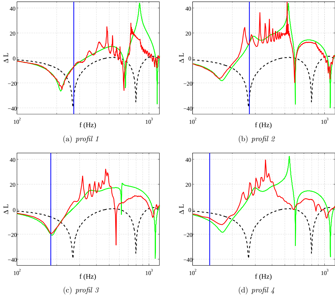
FIGURE 4.3 – Spectres d'atténuation \Delta L à une distance de 50 m au-dessus de profils rugueux composés de diffuseurs. (—) Résultat FDTD ; (—) Solution analytique avec impédance effective (modèle à bosses) ; (- -) Solution analytique pour le profil plat réfléchissant ; (—) Limite fréquentielle théorique du modèle d'impédance effective.
