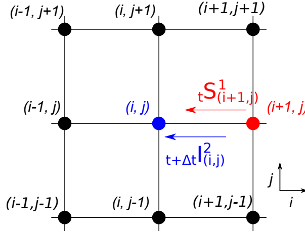
FIGURE 2.6 – Connexion entre deux noeuds pour l'itération temporelle (pas de temps \Delta t ).
