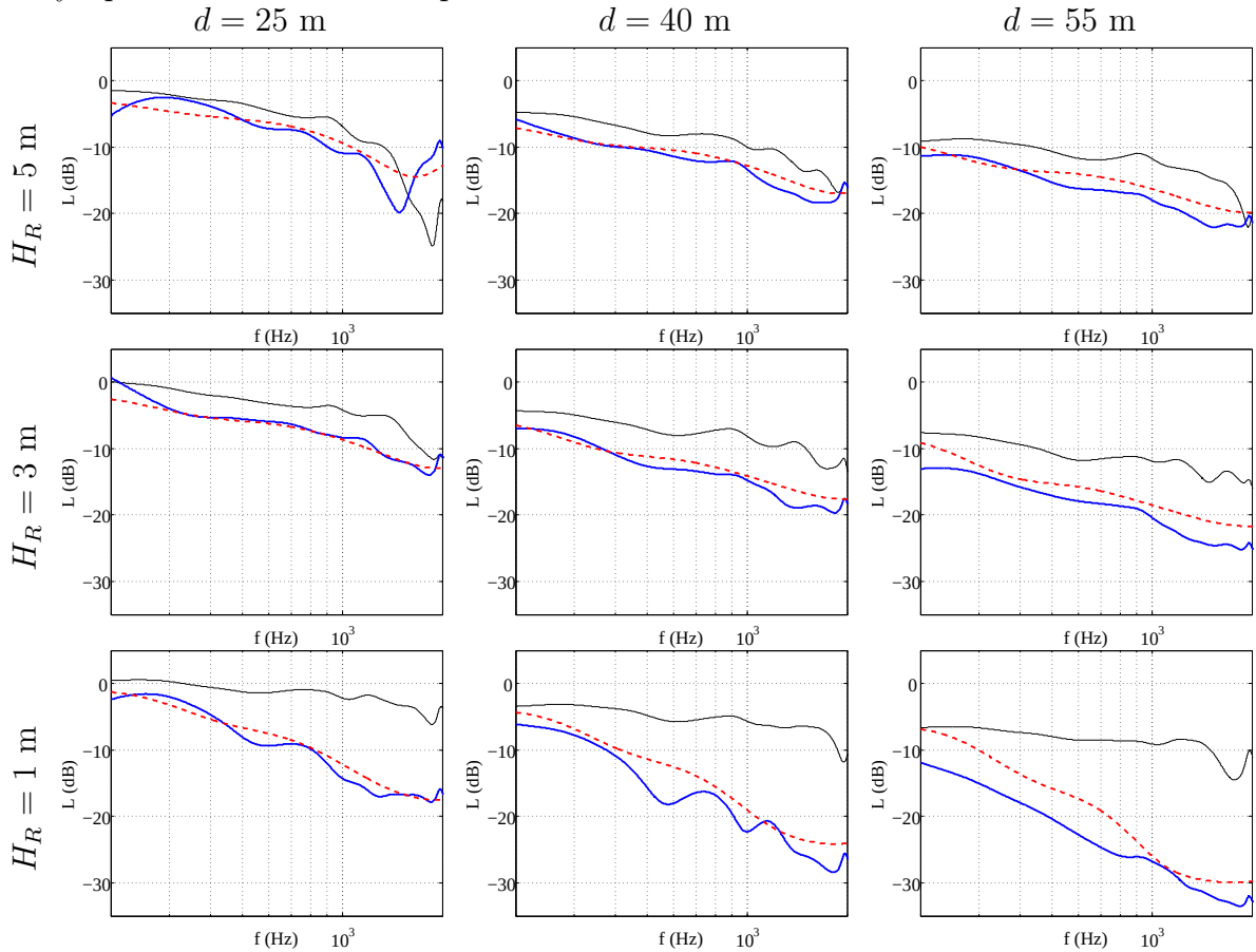
FIGURE 3.12 – Niveaux de pression à différentes positions au-dessus des surfaces réfléchissantes pour H_S = 0.2 m : (—) mesure au-dessus de la surface plane, (—) mesure au-dessus de la surface rugueuse, (- -) solution analytique avec impédance effective.
