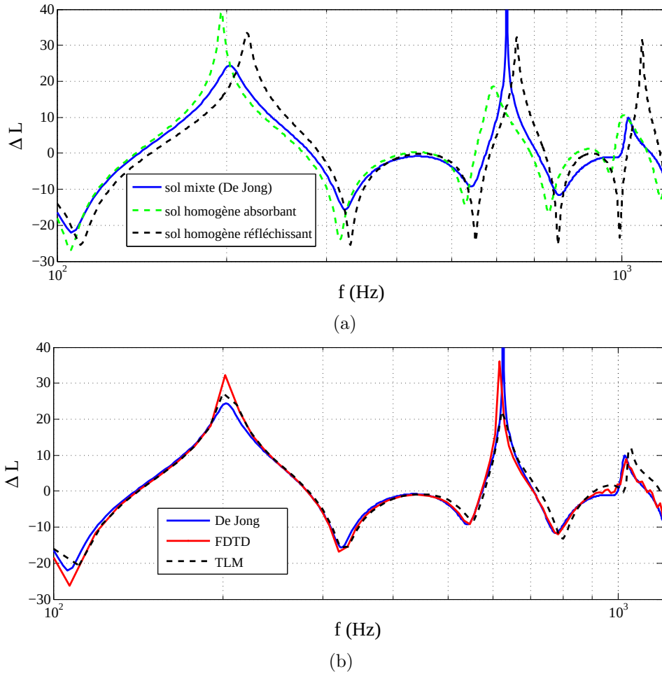
FIGURE 2.14 – (a) Solutions analytiques pour le sol mixte et pour des sols homogènes absorbant ( \sigma = 200 \text{ kN.s.m}^{-4} , e = 0.01 \text{ m} ) et réfléchissant ; (b) Résultats des simulations numériques FDTD et TLM pour le sol mixte.
