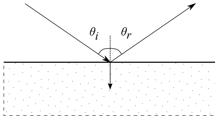
FIGURE 1.5 – Sol à réaction localisée, \theta_i = \theta_r = \theta .
