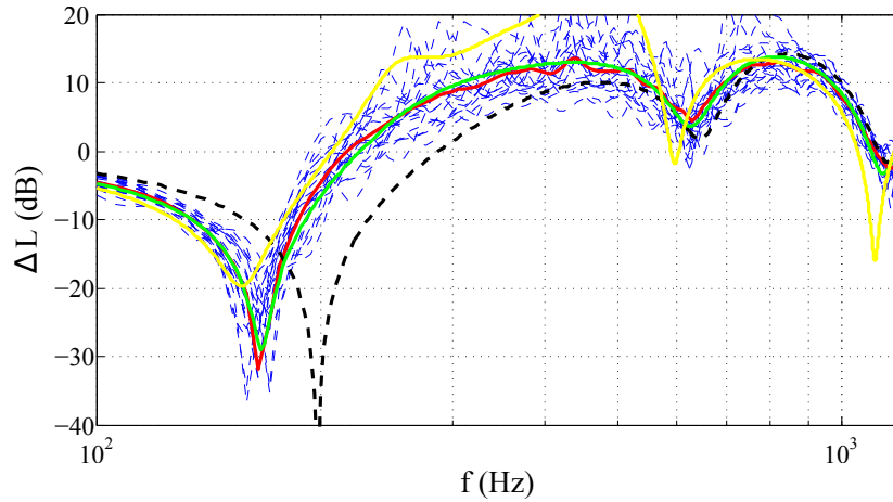
FIGURE 4.9 – Spectres d'atténuation \Delta L au-dessus de 20 tirages aléatoires du sol 1 , H_S = 4 m, H_{R1} = 4 m, H_{R2} = 0.3 m, d = 50 m. (—) Résultats TLM; (—) Résultat TLM moyen; (—) Solution analytique avec le modèle MPP; (—) Solution analytique avec le modèle à bosses formulé par l'équation (4.1); (---) Solution analytique pour le sol plat absorbant
