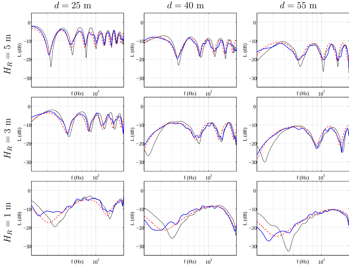
FIGURE C.14 – Niveaux de pression à différentes positions au-dessus des surfaces absorbantes pour H_S = 4 m : (—) mesure au-dessus de la surface plane, (—) mesure au-dessus de la surface rugueuse, (- -) solution analytique avec impédance effective.
