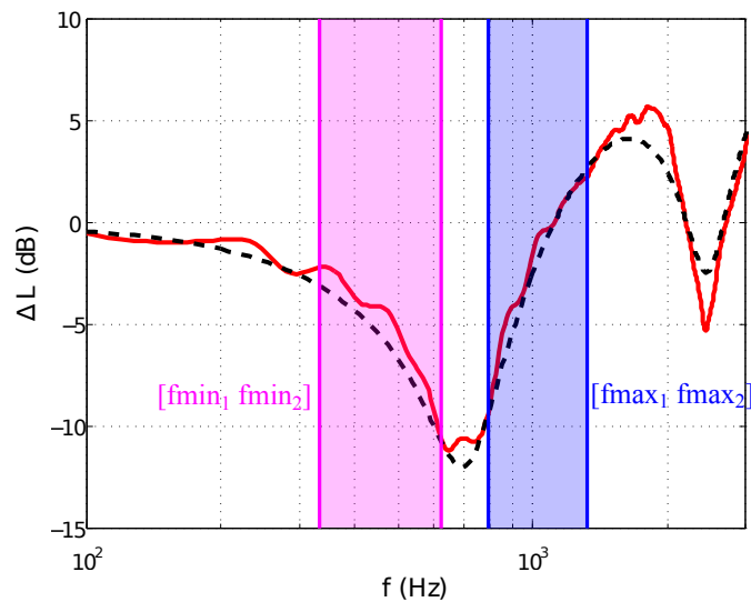
FIGURE 5.8 – Exemple de recalage par la méthode de minimisation sous contraintes. (–) spectre analytique recalé, (—) spectre expérimental bruité dont le creux d'effet de sol est bruité.
