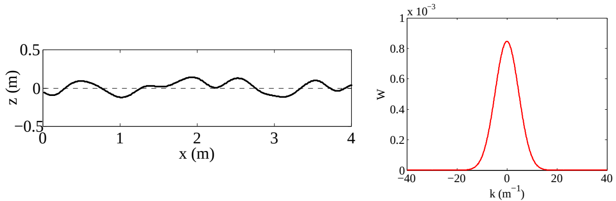
FIGURE 3.2 – Exemple de profil rugueux (à gauche) dont le spectre de rugosité gaussien (à droite) est défini par l'équation (3.2) avec \sigma_h = 0.1m et l_c = 0.3m .
