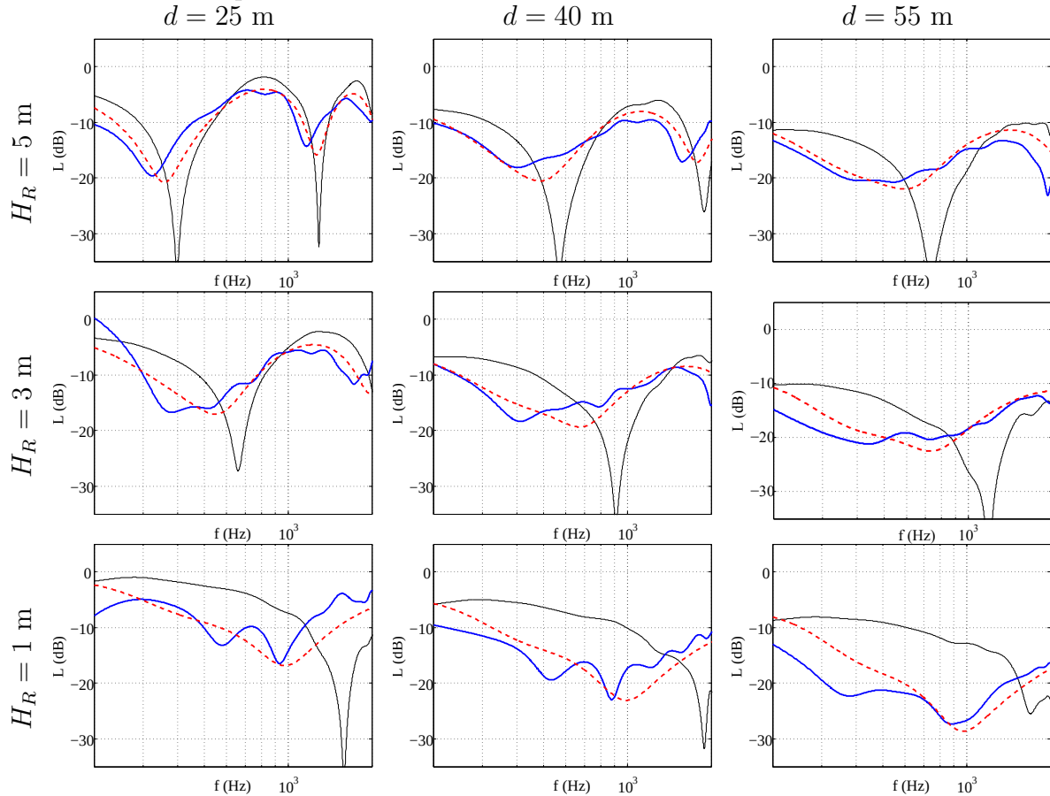
FIGURE C.2 – Niveaux de pression à différentes positions au-dessus des surfaces réfléchissantes pour H_S = 1 m : (—) mesure au-dessus de la surface plane, (—) mesure au-dessus de la surface rugueuse, (- -) solution analytique avec impédance effective.
