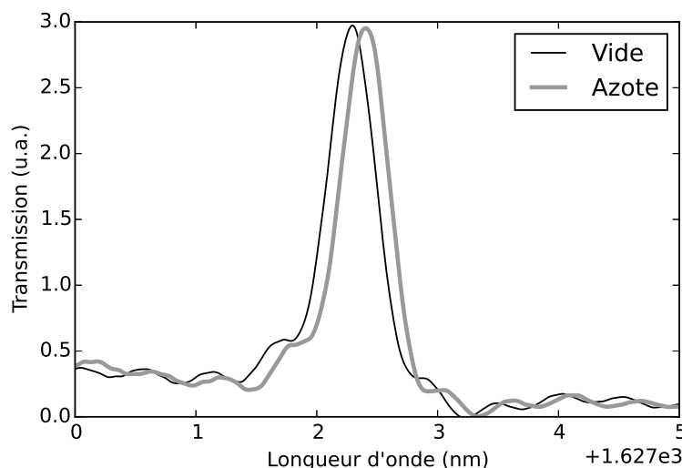
FIGURE 4.10 – Spectre en transmission de la cavité mesurée près de la résonance ( Q=5000 ) lorsque l'indice de réfraction du milieu environnant passe de celui du vide ( n_{\text{vide}}=1 ) à celui de l'azote ( n_{\text{azote}}=1.000294 )
