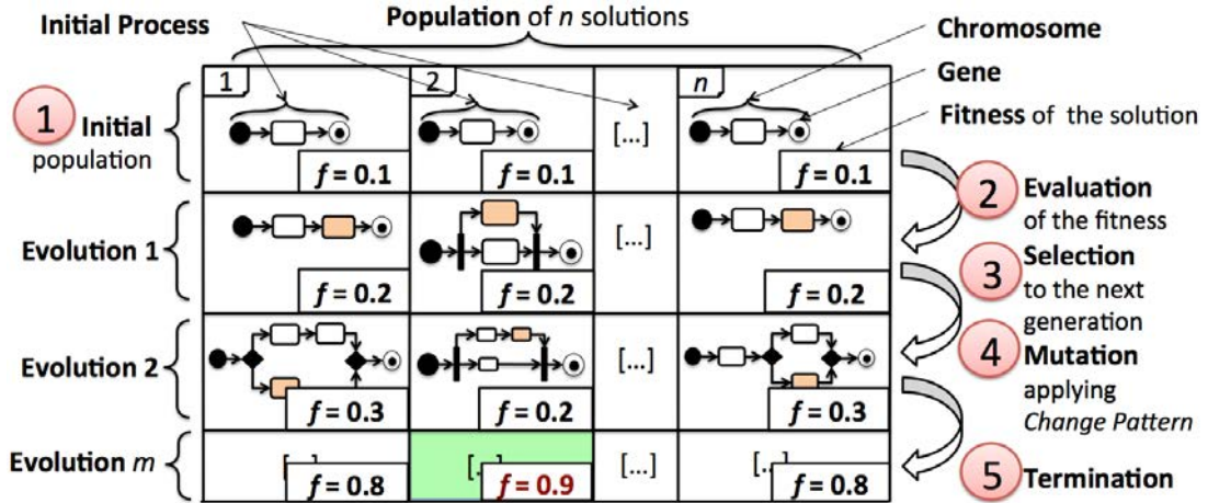
FIGURE 5.5 – Vue globale de l'utilisation d'un GA pour la génération d'un procédé [156]
