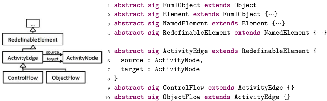
FIGURE 4.7 – Aperçus de la partie pour représenter les ActivityEdge du module Syntax.als
