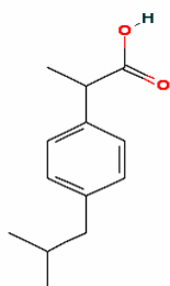
Ibuprofen (IBP)
