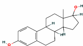
17β-estradiol (E2)
