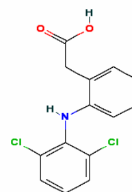
Diclofenac (DCF)
