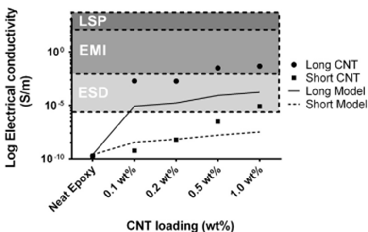
Figure 32. Conductivité électrique en fonction de la charge en NTC pour deux longueurs différentes (échelle log) [76].
