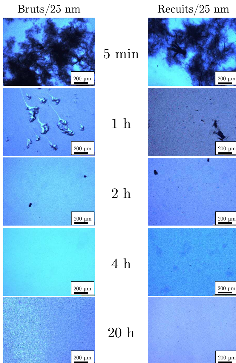
Figure 7. Micrographies de microscopie optique montrant l'évolution de l'état de dispersion en fonction de la durée d'ultrasons pour des suspensions contenant des NTC bruts et recuits de diamètre 25 nm.
