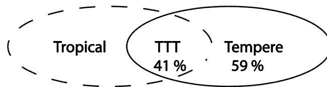
Figure 2. 4 : Schéma conceptuel de la relation entre les TTT et les perturbations tempérées (cercle noir) et les mécanismes tropicaux (pointillés noirs).
