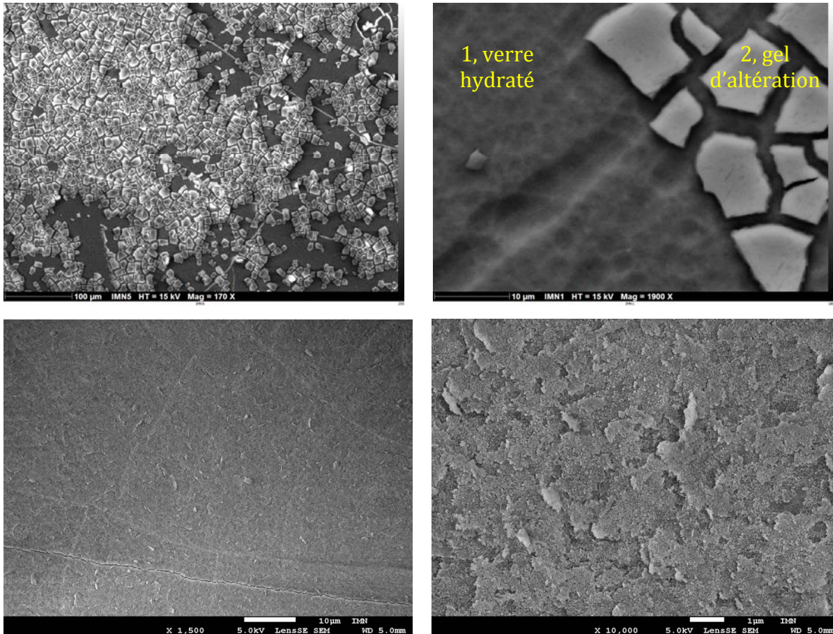
Image V-2. Images MEB de la couche d'altération formée sur la surface d'un échantillon de verre ISG non irradié après 236 jours de lixiviation dans une eau ultra pure à 90°C.
