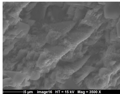
Image V-16. Observation de calcites de formule \text{CaCO}_3 provenant des solutions de lixiviations d'échantillons de verre Planilux.
