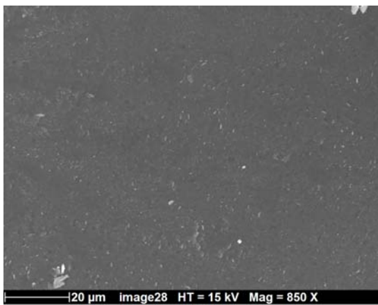
Image V-8. Image MEB du gel d'altération à la surface d'un échantillon de verre ISG préalablement irradié à la fluence de 6,4 \times 10^{13} Au/cm 2 .
