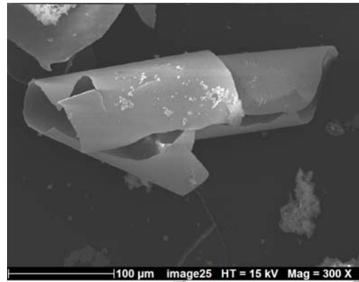
Image V-15. Images MEB de précipités contenus dans les solutions de lixiviations des échantillons de verres Planilux altérés pendant une durée comprise entre 236 et 260 jours.
