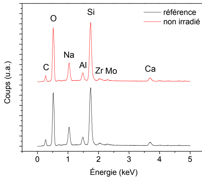
Figure IV-37. Spectres EDX du verre SON68 mesurés sur la surface non irradiée et sur la surface irradiée du verre SON68 endommagée avec des ions Au de 7 MeV à une fluence de 3 \times 10^{14} Au.cm -2 .
