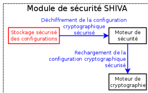
(c) 3ème étape : sécurisation du moteur cryptographique
