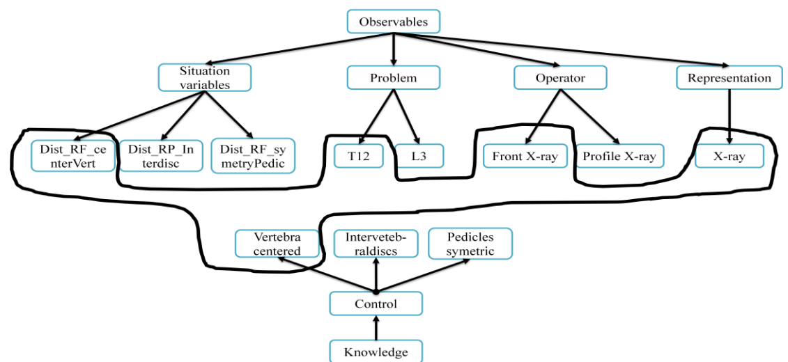
Figure 26 : En haut : rappel de la trace utilisée dans cet exemple. En bas, graphe d'instanciation avec l'arête issue de la trace, reliant T12 , Front\ X-ray , X-ray et Dist\_RF\_centervert à Vertebra\ centered .
