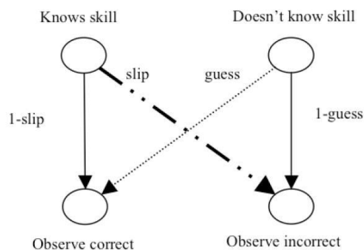
Figure 1 : Schéma illustrant la prédiction des réponses de l'apprenant (correct ou incorrect) à partir des deux états ( Knows skill et doesn't know skill ) d'une connaissance et des paramètres slip et guess associés à cette connaissance (Beck et Sison, 2006).
