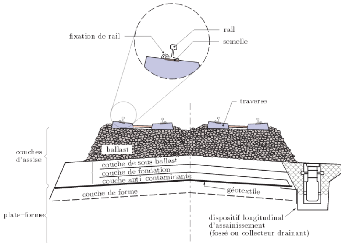
Figure I.1-15 : Structure d'une plateforme ferroviaire [KOU 09]
