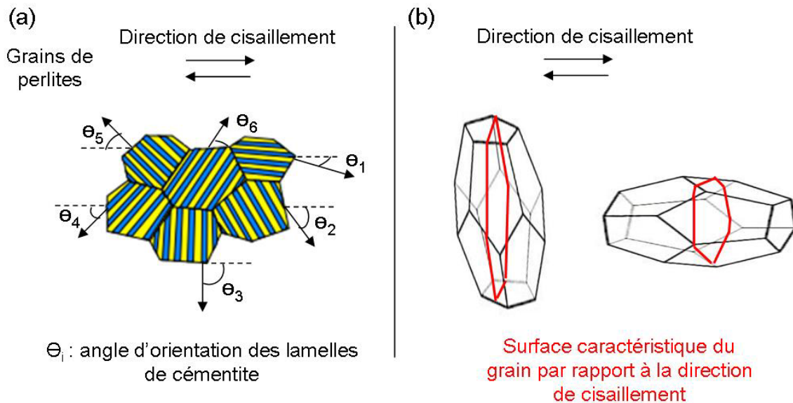
Figure V.2-17 : Positionnement de la microstructure par rapport à la direction de cisaillement : (a) Orientation des lamelles, (b) Orientation de la matrice ferritique
