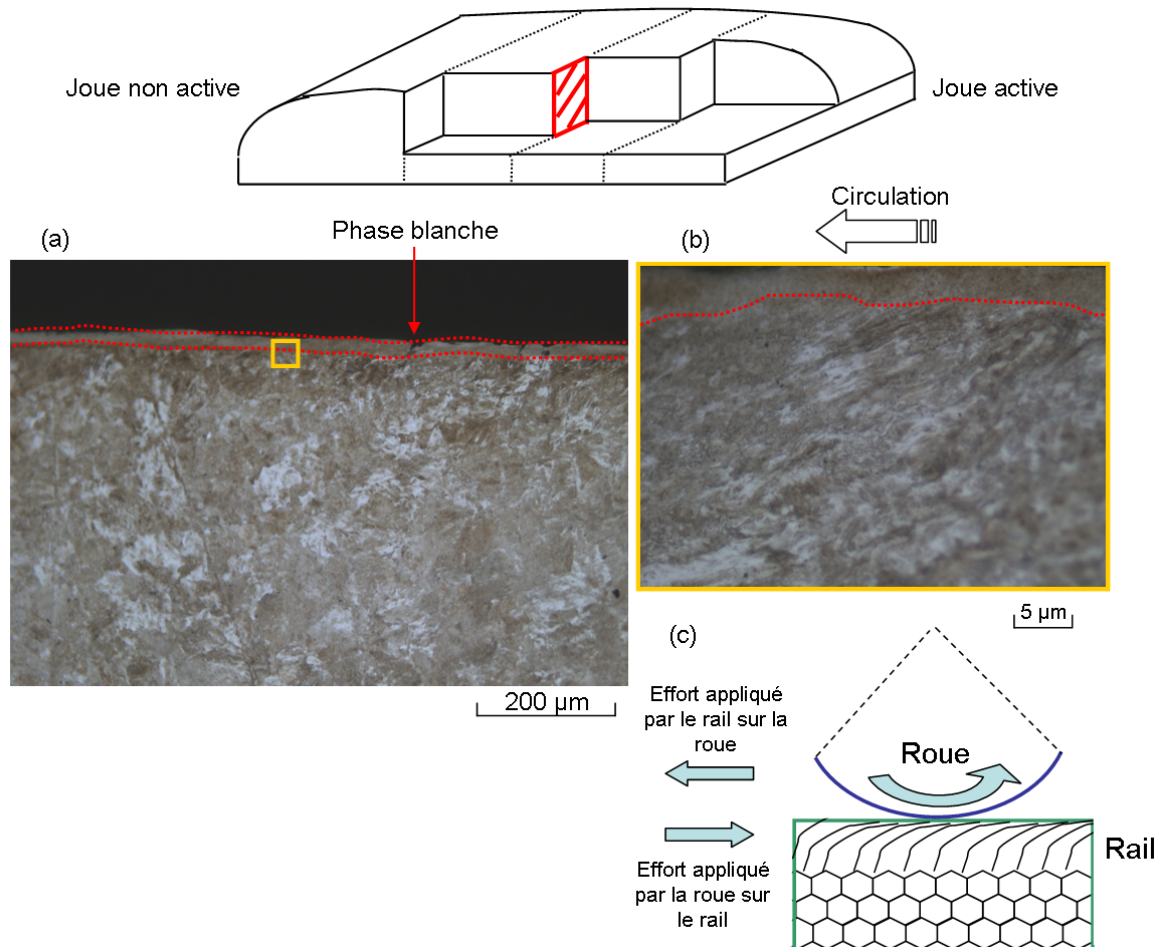
Figure V.1-16 : Coupe longitudinale au centre du rail R260, (a) Phase blanche continue, (b) Ecroûssage et réorientation de la matière
