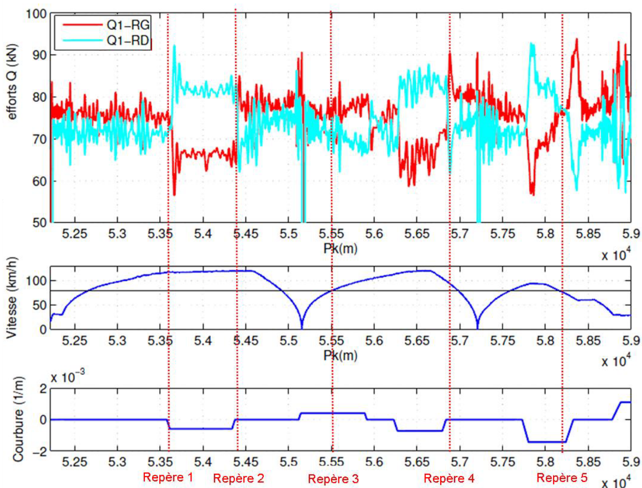
Figure 35 : Efforts verticaux des roues gauche et droite de l'essieu 1 pour la marche 34-2-10 (Circulation vers les PK croissants)
