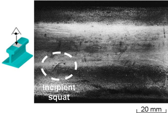
Figure II.1-3 : Fissure naissante de squat identifiée par Clayton [CLA 82]
