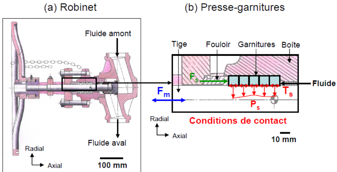
Figure 1-2 : vue en coupe d'un robinet à soupape : (a) robinet, (b) presse-garnitures
