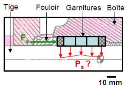
Figure 2-1 : principe de la caractérisation volumique des garnitures
