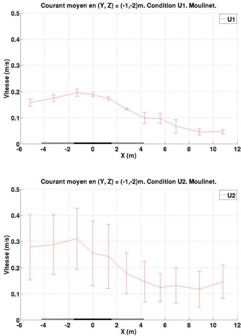
Figure VII.1 – Intensité du courant mesurée avec le moulinet à hélice. En haut : U_1 . En bas : U_2
