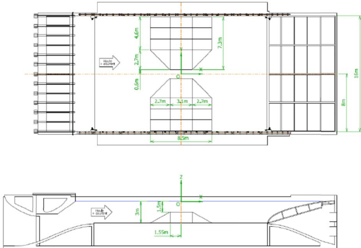
Figure III.3 – Plan de masse de la topographie (Océanide, 2013)
