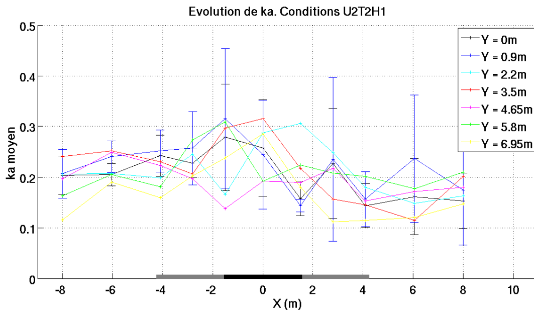
Figure VII.12 – Evolution de la cambrure de la houle
