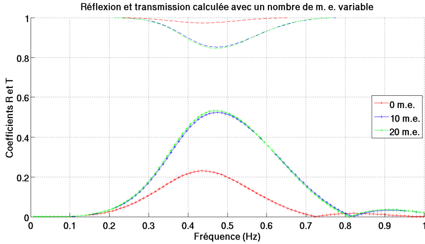
Figure II.4 – Evolution des coefficients de réflexion (+) et de transmission (-) en fonction de la fréquence et du nombre de modes évanescents (m.e.) au dessus d'une plaque plane. L = 1.53m , h_0 = 3m , h_s = 0.5m , h_f = 0.6m
