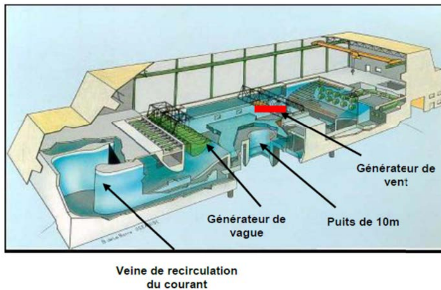
Figure III.1 – Vue en coupe du Bassin de Génie Océanique FIRST (Océanide (2013))
