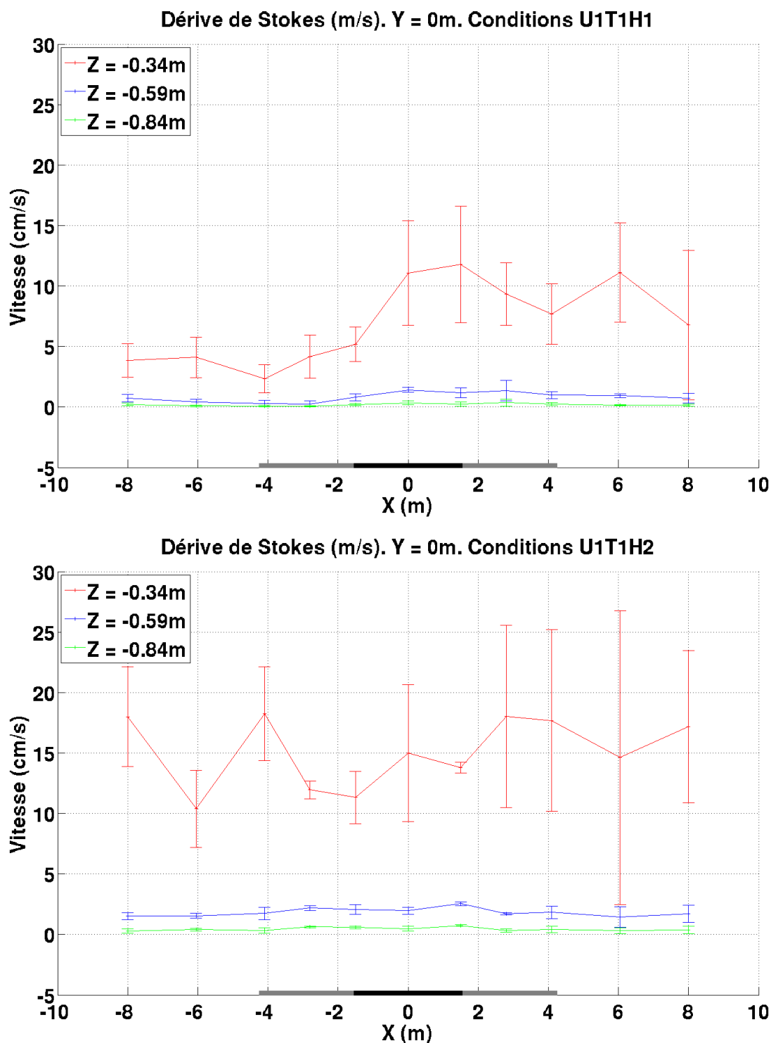
Figure VII.27 – Estimation de la dérive de Stokes en Y = 0 . Conditions U_1, T_1, H_1 et U_1, T_1, H_2
