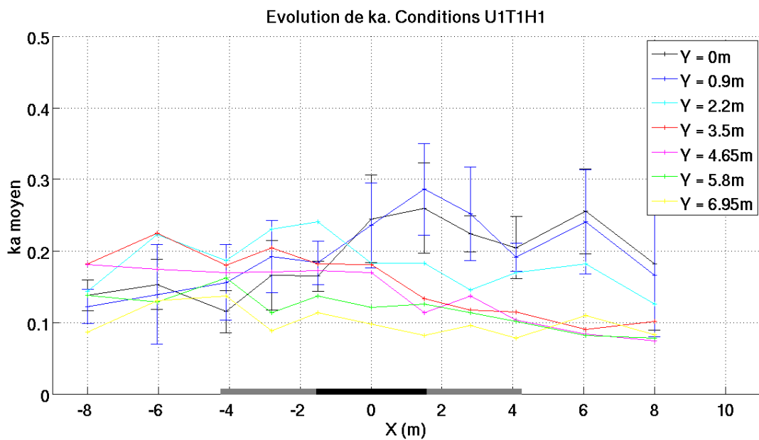
Figure VII.8 – Evolution de la cambrure de la houle
