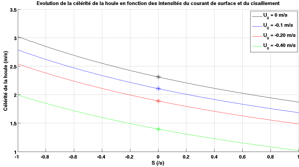
Figure III.9 – Influence du cisaillement sur la célérité de la houle pour différentes valeurs du courant de surface. (-) : Célérité de la houle avec un courant de la forme U(z) = Sz + U_0 . (*) : Célérité de la houle avec un courant non cisailé pour les différentes valeurs du courant de surface
