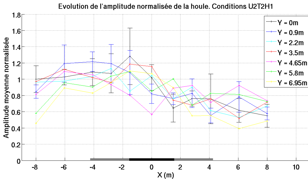
Figure VII.11 – Evolution de l'amplitude de la houle normalisée par l'amplitude mesurée au point (-8, 0)m , pour la condition de houle U_2 T_2 H_1 .
