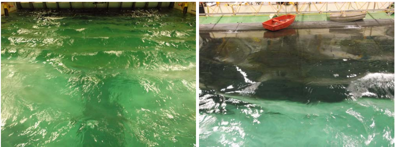
Figure VII.24 – Phase de la houle en amont des bosses (à gauche) et en aval des bosses (à droite) pour les conditions hydrodynamiques U_2, T_2, H_1 .
