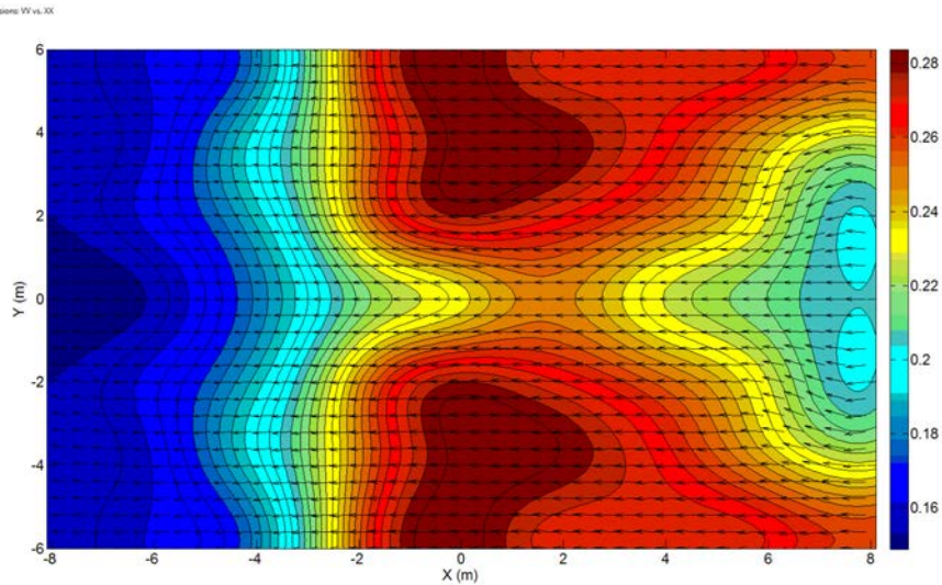
Figure III.7 – Champ de courant U_0 extrapolé à partir des données du courantomètre immergé à 25cm de profondeur. Extrait de Rey et al. (2014).
