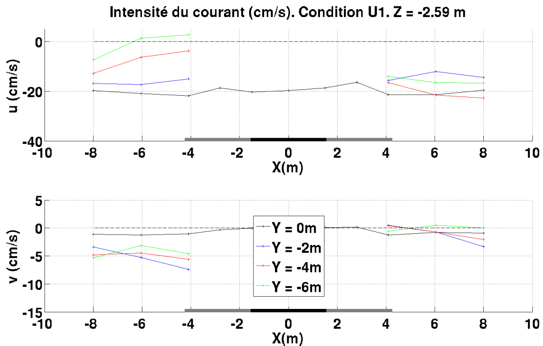
Figure VII.3 – Evolution du contre-courant U_1 . Z = -2.59m . En haut : composante longitudinale. En bas : composante transverse
