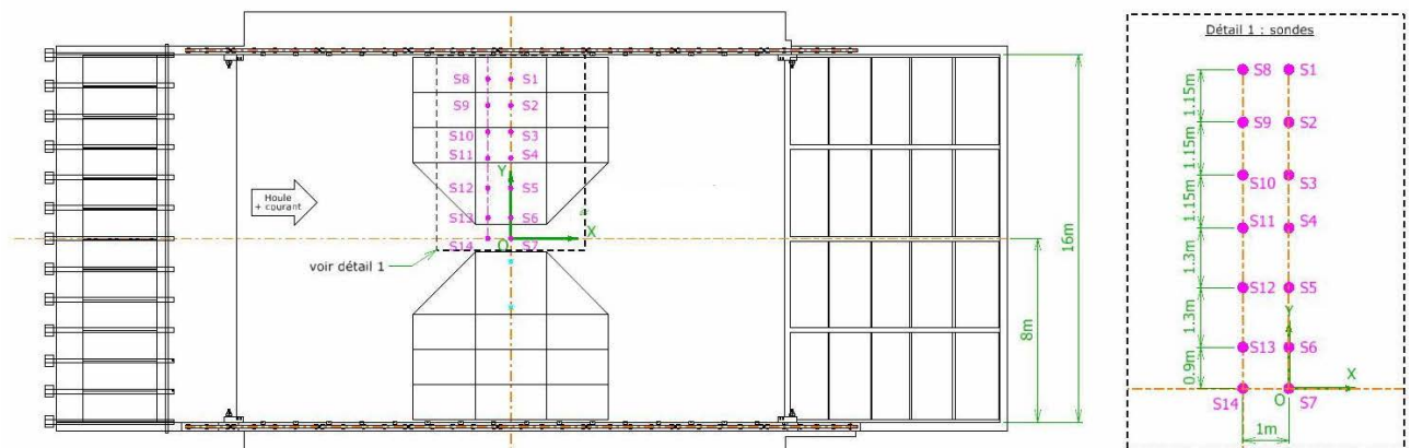
Figure VI.4 – Disposition des sondes à houles dans le bassin (Océanide, 2013)
