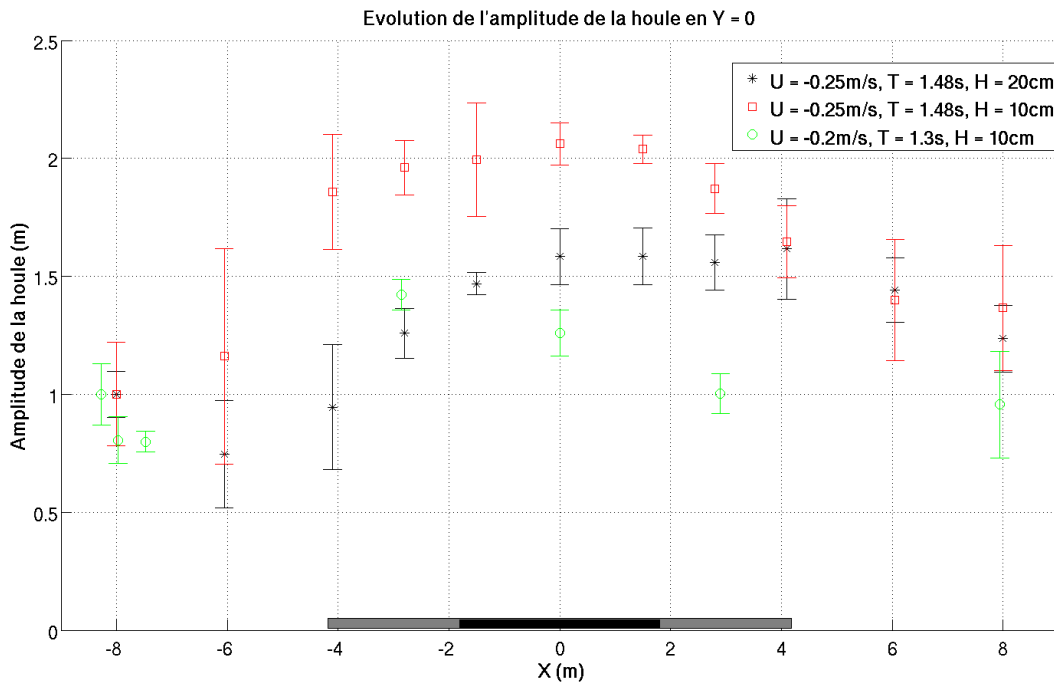
Figure VII.18 – Amplitude moyenne de la houle normalisée par la valeur moyenne de l’amplitude en X = -8m et écart-types. Campagnes de 2007 et de 2008
