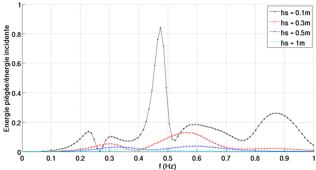
Figure IV.6 – Rapport entre l'énergie piégée par les modes évanescents et le flux d'énergie incident par unité de période lorsque la profondeur d'immersion h_s varie. Les autres dimensions sont h_0 = 3m , e = 0.1m et L = 1.53m
