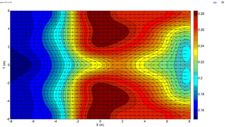
Figure III.7 – Champ de courant U_0 extrapolé à partir des données du courantomètre immergé à 25cm de profondeur. Extrait de Rey et al. (2014).
