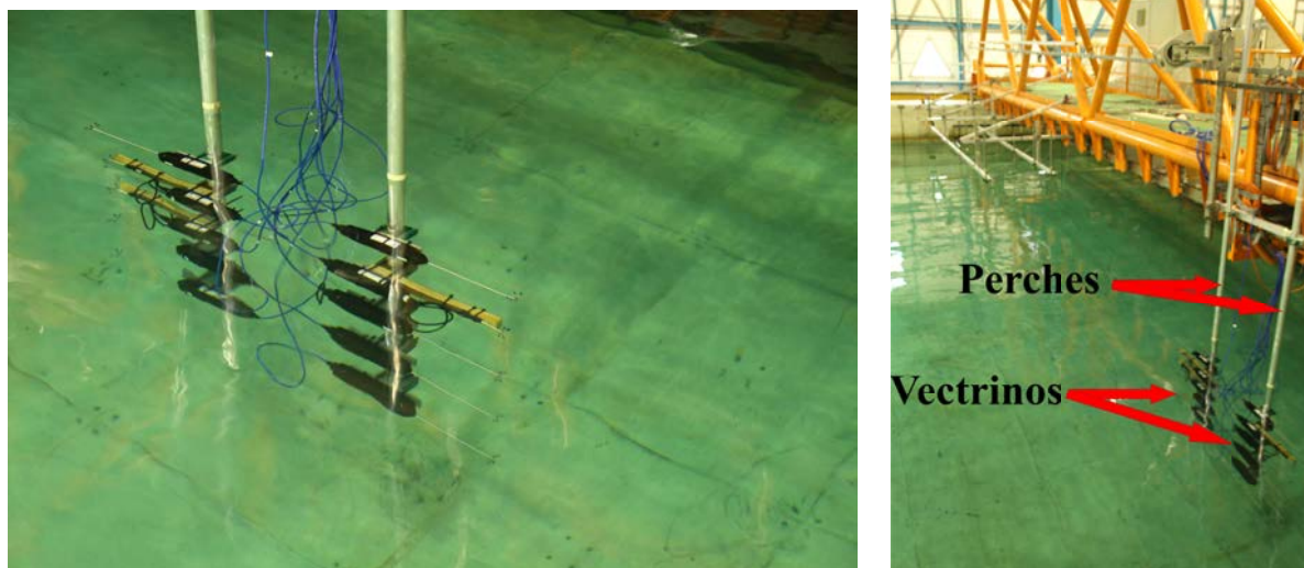
Figure VI.5 – Installation des dix Vectrino sur les deux perches (à gauche), et installation des deux perches sur le chariot mobile selon l'axe Y (à droite)
