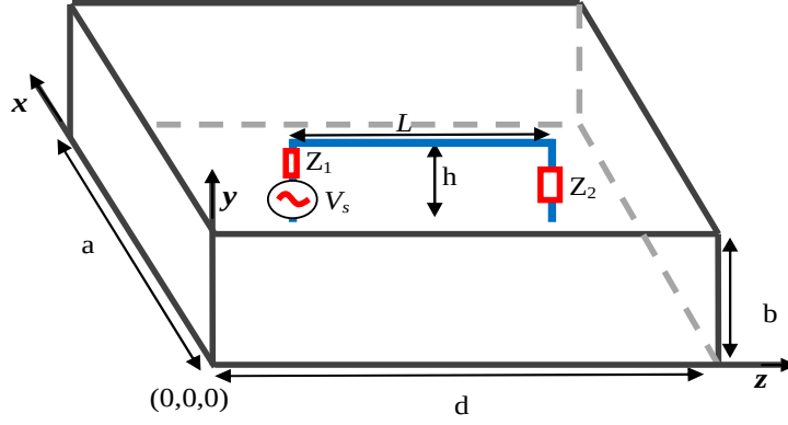
Figure V. 24: Enceinte contient une LT excitée par une source de tension.
