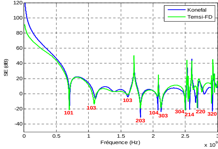
Figure III. 34: Comparaison entre le résultat de S_E calculé par le modèle de Konefal et celui simulé par Temsi-FD.
