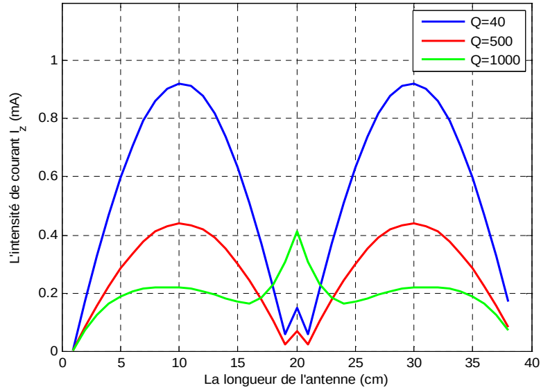
Figure II. 9: Courant distribué le long de l'antenne pour différentes valeurs de Q .
