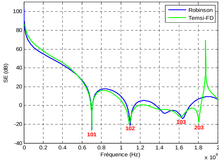
Figure III. 12: Calcul de S_E obtenu par Tamsi-FD et le modèle de Robinson.
