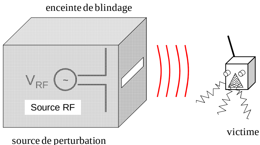
Figure I. 6: Contenir les émissions rayonnées à l'intérieur de l'enceinte blindée.
