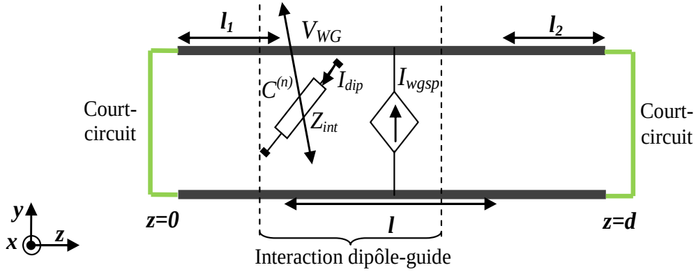
Figure IV. 4: Couplage mutuel dipôle-enceinte [21].
