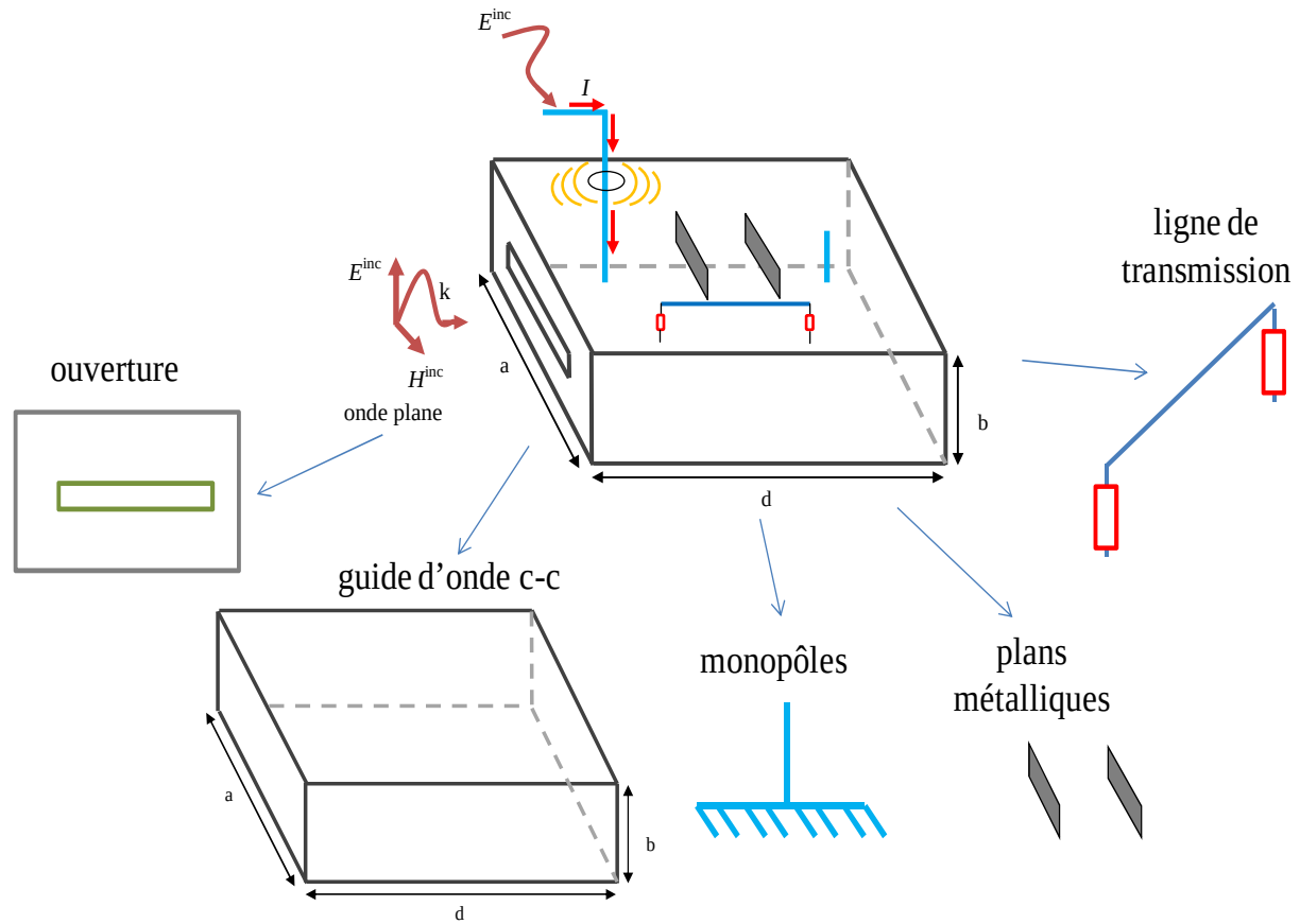
Figure I. 22: Découpage topologique de la structure.
