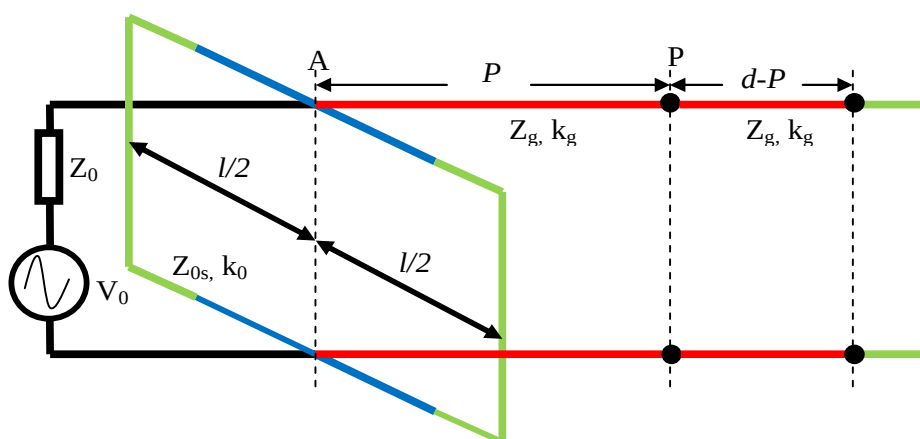
Figure III. 8: Circuit équivalent de Robinson [12].
