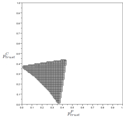
Figure 2.20 – Service de détection pour un seuil 0.8
