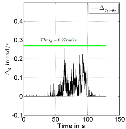
Figure 5.15 – Faute logicielle sur le filtre de Kalman 1 : Comparaison des sorties de Gyro_1 et Gyro_2
