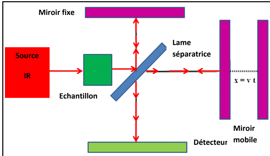
Figure 2.24: Principe de l'interféromètre de Michelson
