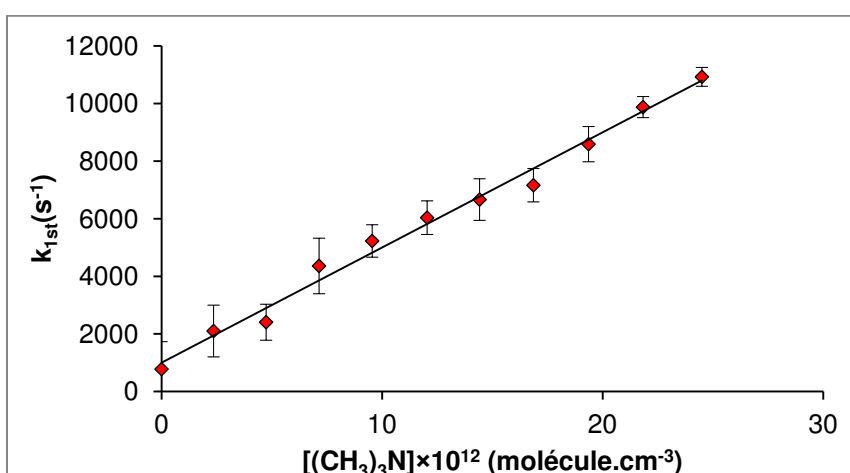
Graphique du second ordre pour la réaction \text{CN} + (\text{CH}_3)_3\text{N} à 71.6 K dans Hélium [\text{He}] = 6.01 \times 10^{16} \text{ cm}^{-3}
