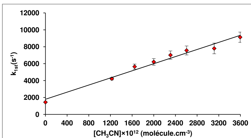
Graphique du second ordre pour la réaction CN + CH 3 CN à 141.6 K dans l'argon [Ar]= 6.95×10 16 cm -3
