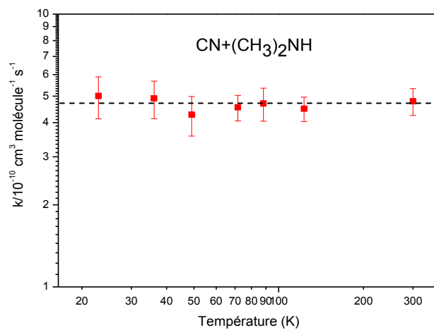
Figure 5.9 : Variation de la constante de vitesse pour la réaction de CN + (CH 3 ) 2 NH en fonction de la température
