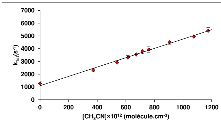
Graphique du second ordre pour la réaction CN + CH 3 CN à 132.9 K dans l'argon à 0.62 mbar [Ar]= 3.39×10 16 cm -3
