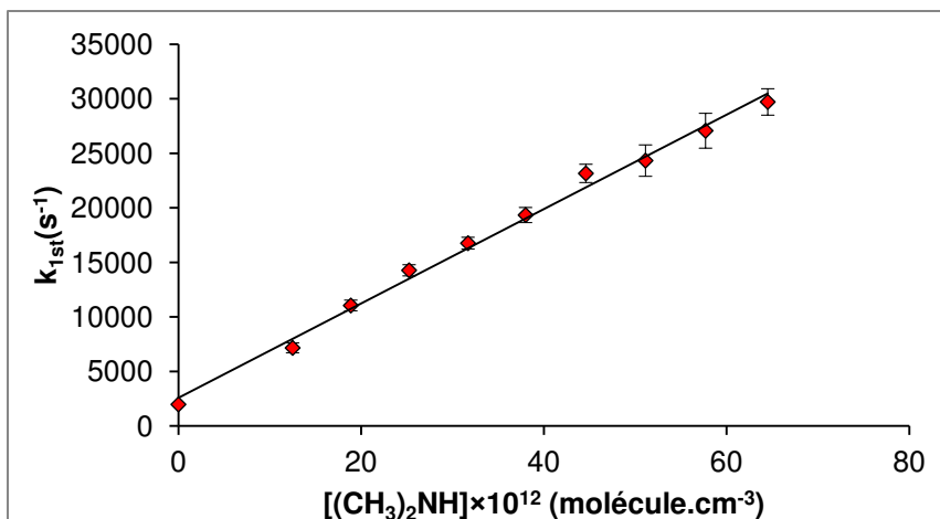
Graphique du second ordre pour la réaction CN + (CH 3 ) 2 NH à 49.1 K dans Hélium [He]= 10.4×10 16 cm -3
