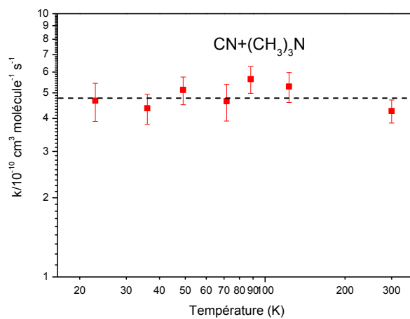
Figure 5.10 : Variation de la constante de vitesse pour la réaction de CN + (CH 3 ) 3 N en fonction de la température
