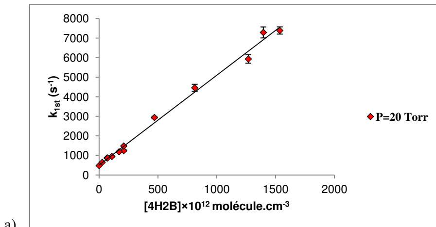
Annexe 3.1 : Droite représentant la variation des constantes de vitesse de pseudo premier ordre en fonction de la concentration du 4H2B à : a) 20 Torr, b) 40 Torr, c) 80 Torr, d) 330 Torr
