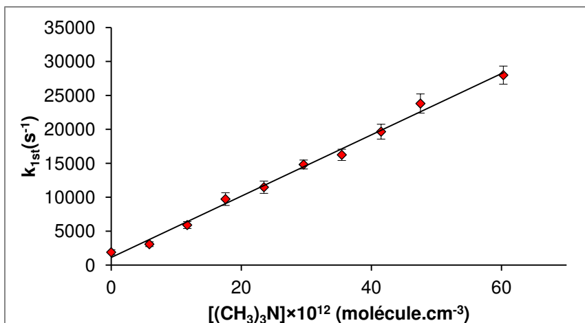
Graphique du second ordre pour la réaction \text{CN} + (\text{CH}_3)_3\text{N} à 49.1 K dans Hélium [\text{He}] = 10.4 \times 10^{16} \text{ cm}^{-3}
