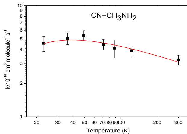
Figure 5.8 : Variation de la constante de vitesse pour la réaction de CN + CH 3 NH en fonction de la température
