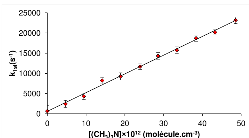
Graphique du second ordre pour la réaction \text{CN} + (\text{CH}_3)_3\text{N} à 123 K dans Hélium [\text{He}] = 12.7 \times 10^{16} \text{ cm}^{-3}
