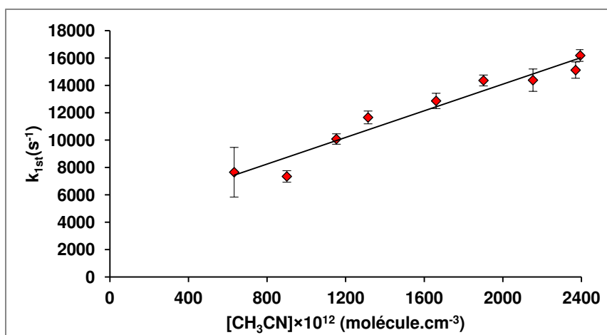
Graphique du second ordre pour la réaction CN + CH 3 CN à 136.2 K dans l'argon [Ar]= 11.92×10 16 cm -3
