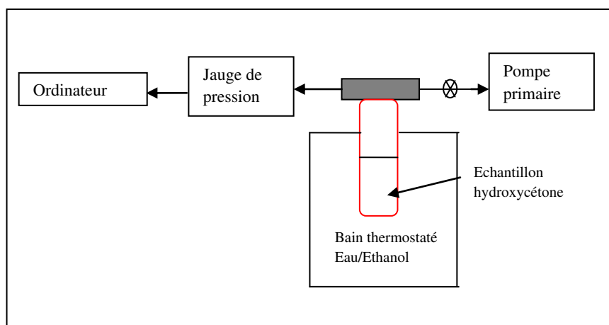
Figure 3.2: Dispositif expérimental pour la mesure de la pression de vapeur à Rennes
