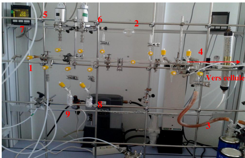
Figure 2.23: Photo du système d'introduction des réactifs utilisé à UCLM
