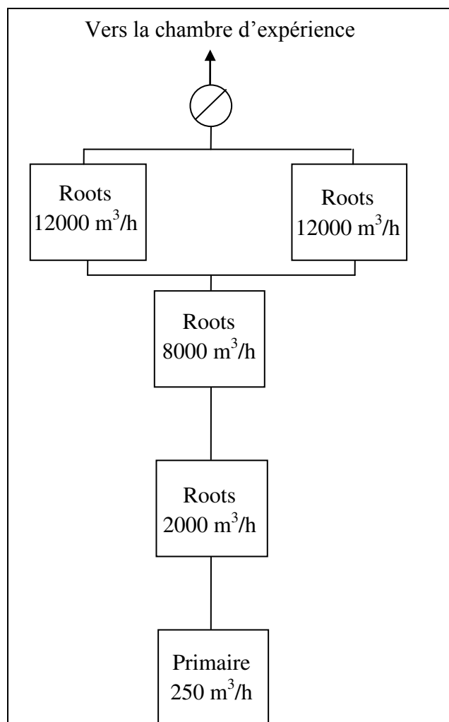
Figure 2.8 : Principe du groupe de pompage CRESU de Rennes (24000 m 3 /h)
