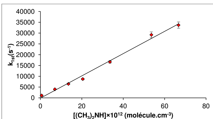
Graphique du second ordre pour la réaction CN + (CH 3 ) 2 NH à 71.6 K dans Hélium [He]= 6.01×10 16 cm -3
