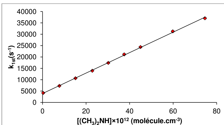
Graphique du second ordre pour la réaction CN + (CH 3 ) 2 NH à 123 K dans Hélium [He]= 12.7×10 16 cm -3
