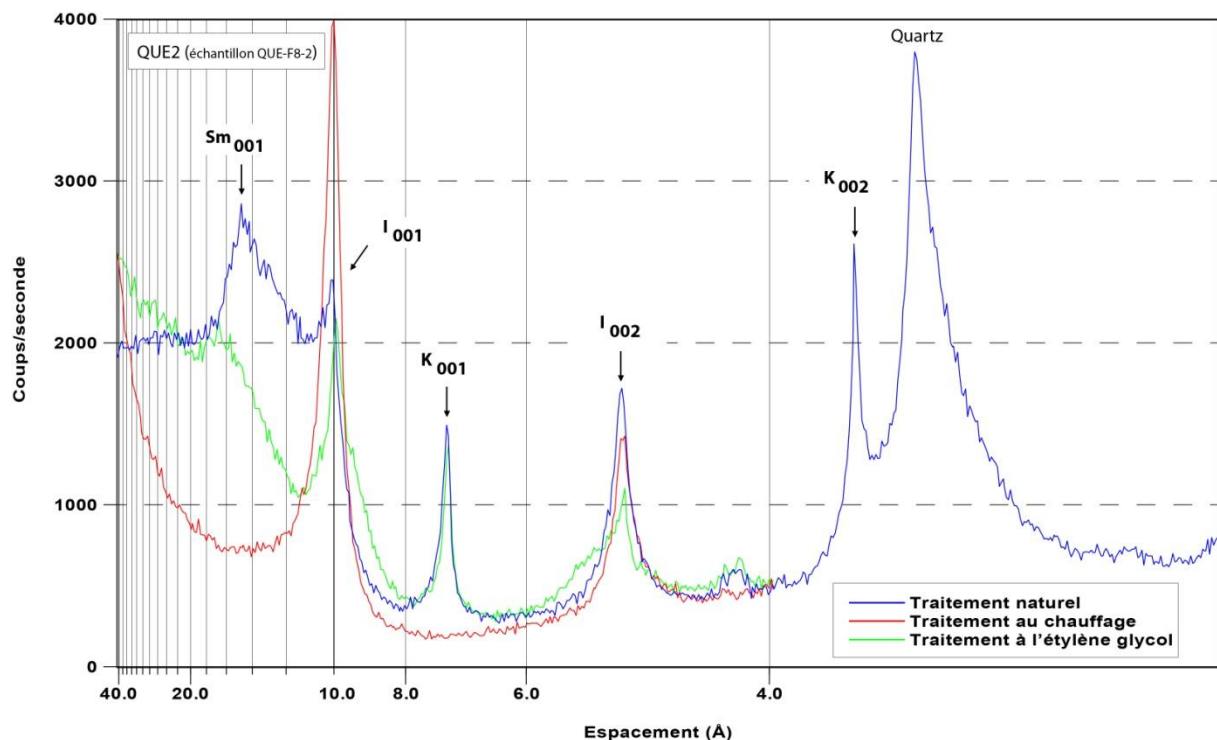
Figure 5. Exemple de spectre de diffraction DRX d'un échantillon de la nappe de Quétiéville.
