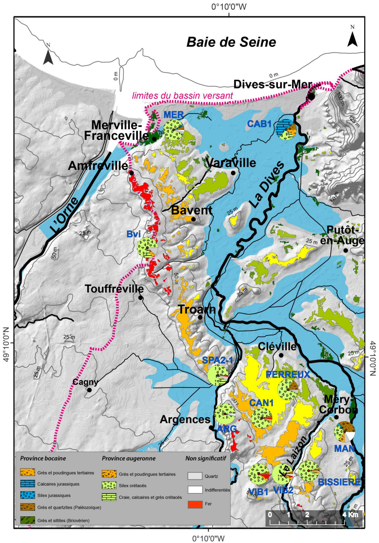
Figure III.110 Cartographie et pétrographie des dépôts fluviaux quaternaires du cours de la Dives, entre Quétiéville et Dives-sur-Mer
