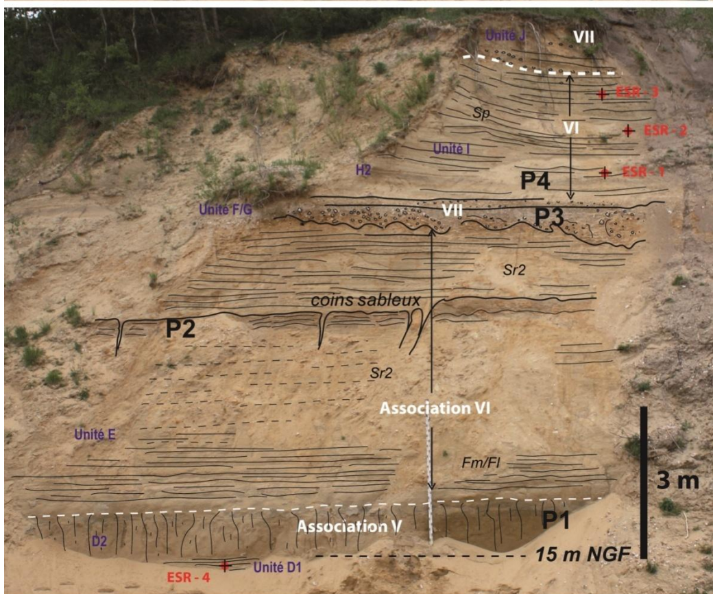
Figure III.38 Unité moyenne de Tourville-la-Rivière (photo: Jamet, 2014). P1 à 4 : paléosols, association V : estran vaseux avec pédogenèse, association VI : barre sableuse tidale et association VII : estran sableux tidal avec apports de versant ; Unités lithologiques d'après Lautridou (1985).
