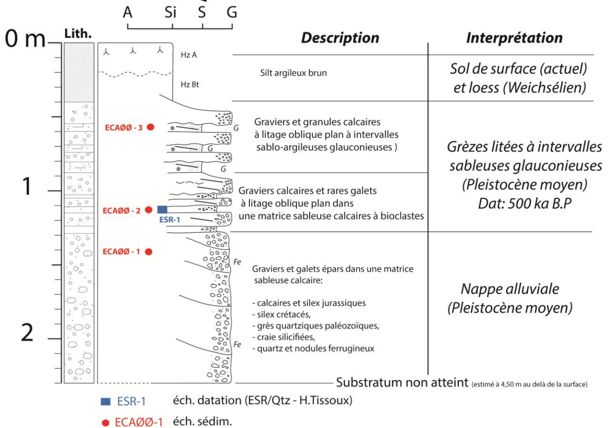
Figure III.94 Photographie (Jamet) et coupe sédimentologique de la terrasse d'Ecajeul au liedit « La Grotte »
