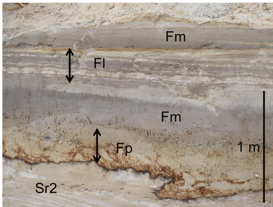
Figure III.32 Photographie des faciès fins silto-argileux des unités D1 à D3 (photo : Jamet, 2012)
