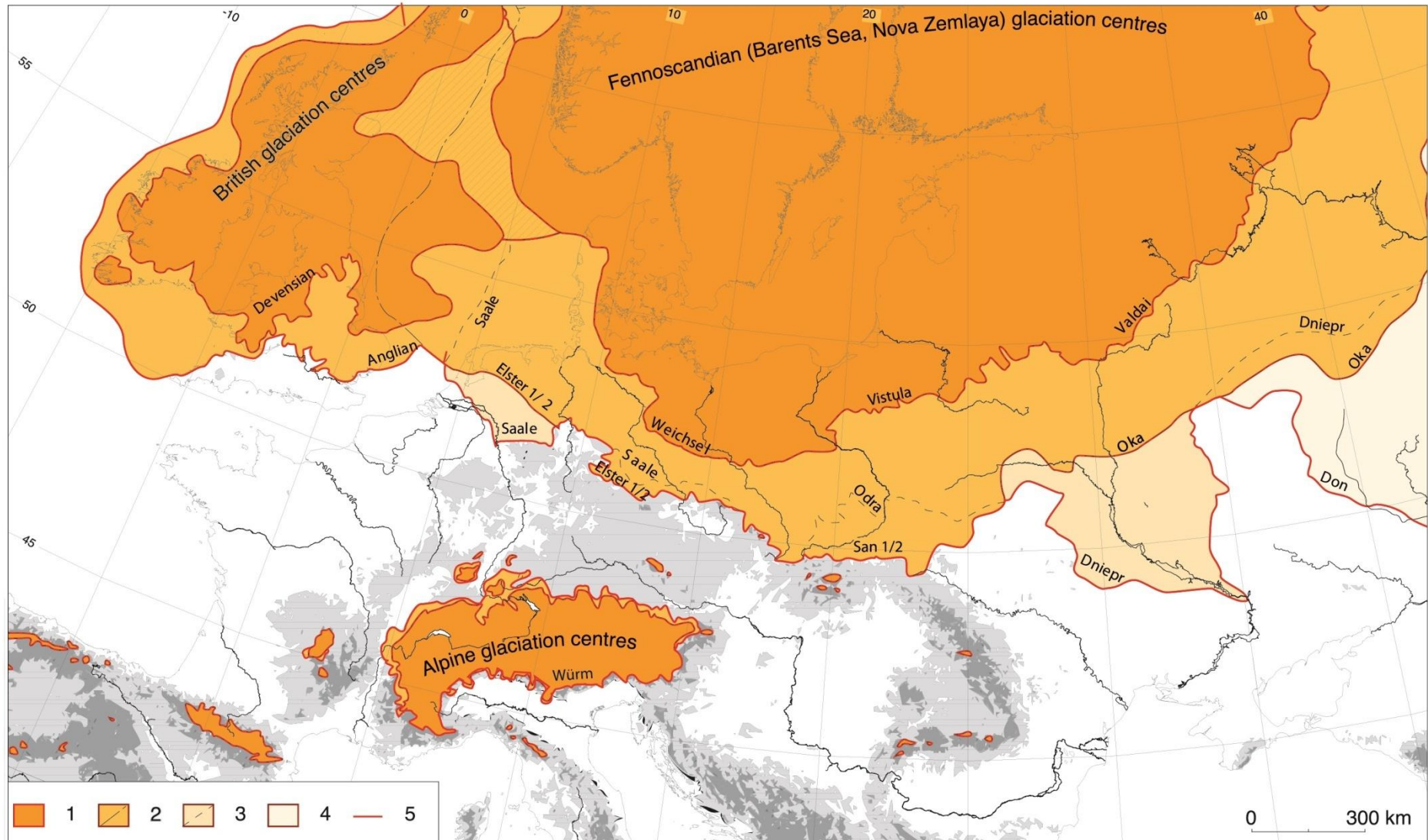
Figure I.13. Extension des glaciations quaternaires en Europe du Nord-Ouest et centrale (in Gijssel, 2006) Légende : Extension des glaces (1) au Weichsélien (Würm), (2) à l'Elstérien (Mindel), (3) au Saalien (Riss) ; (4) : zones non englacées au Weichsélien (5) Limite maximale des glaciations pléistocènes.
