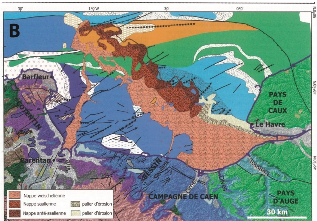
Figure III.8 Cartographie des trois nappes alluviales anté-saaliennes, saaliennes et weichséliennes du remplissage pléistocène de la paléovallée de la Seine (Benabdellouahed, 2011). (voir figure III.4 pour la légende de la carte géologique)
