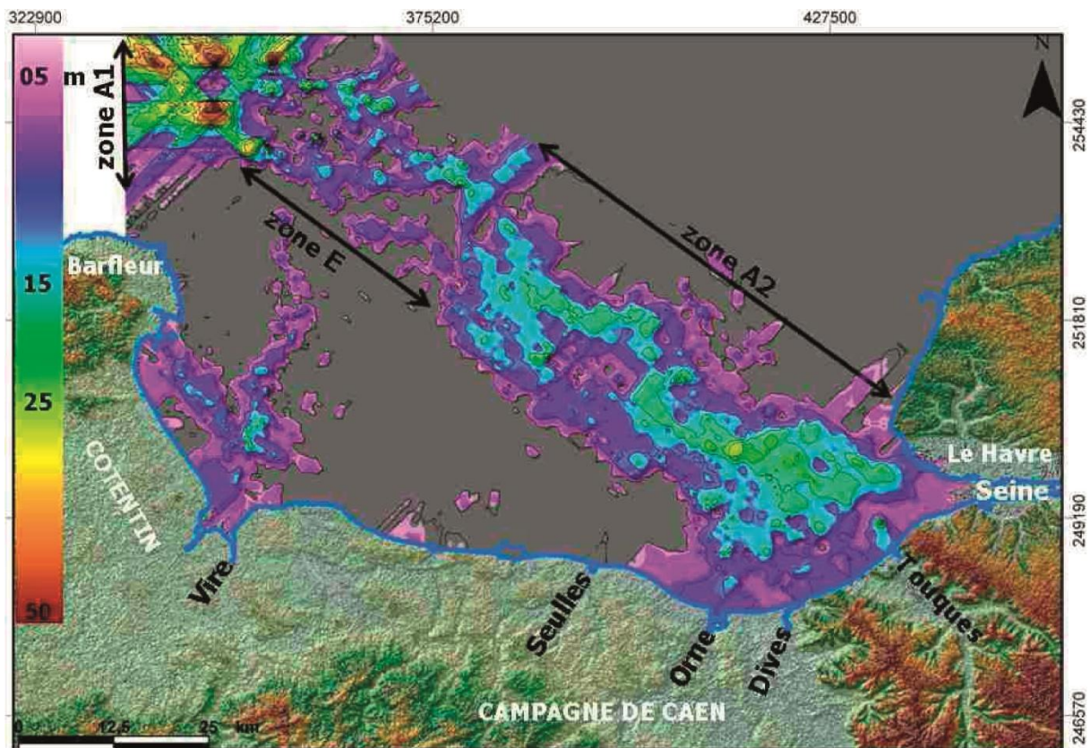
Figure III.23 Carte des isopaques des nappes alluviales pléistocènes et des dépôts holocènes en baie de Seine (Benabdellouahed 2011). Zones A1 et A2 : accumulation sédimentaire, zone E : zone en érosion.
