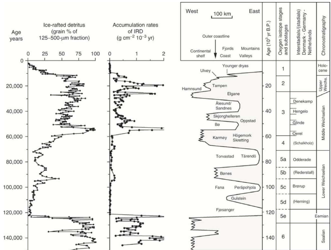
Figure I.16 Corrélation entre les stades isotopiques de l'oxygène, les taux de grains de sables transportés par radeaux de glace et les fluctuations de la calotte fennoscandienne occidentale depuis la fin du Saalien (in Mangerud et al. , 2011). À droite, la courbe montre les fluctuations de la marge occidentale de la calotte fennoscandienne. À gauche, les courbes montrent le nombre et les taux d'accumulation des sables glaciaires dans les carottes de sédiments en mer de Norvège.
