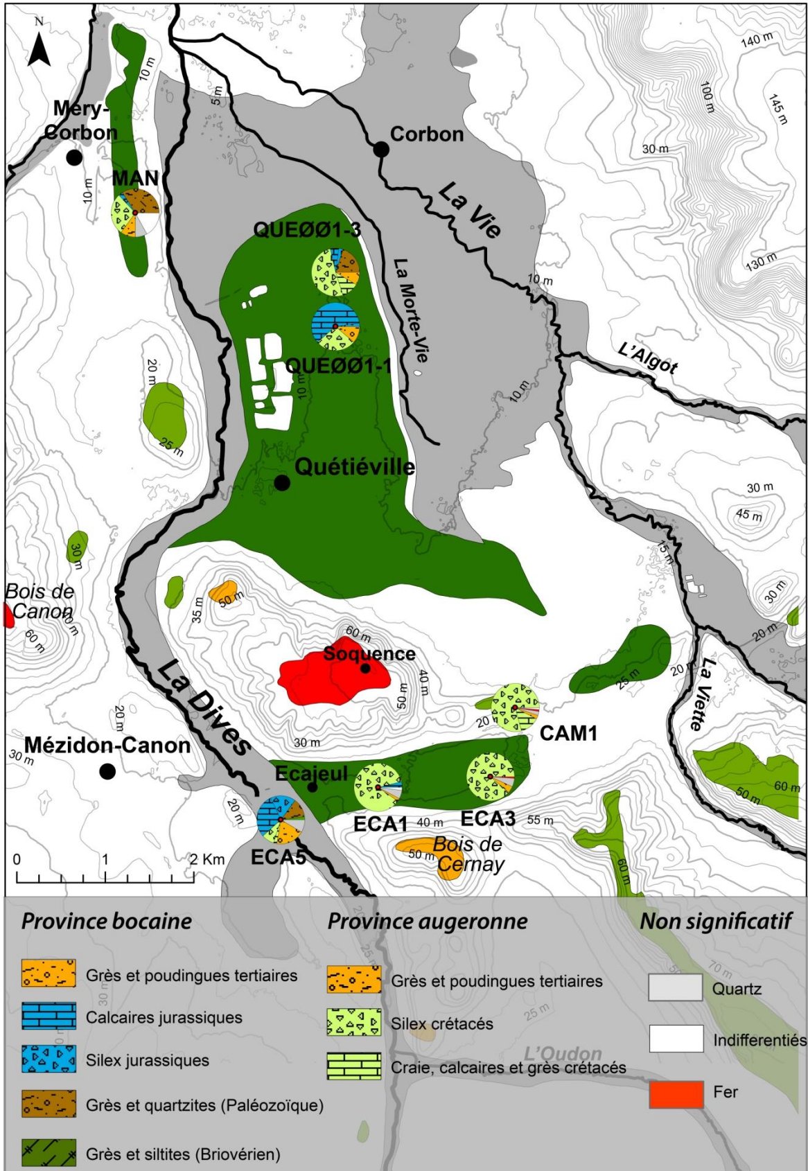
Figure III.100 Cartographie et pétrographie des dépôts fluviaux du cours moyen de la Dives, entre Ecajeul et Quétiéville
