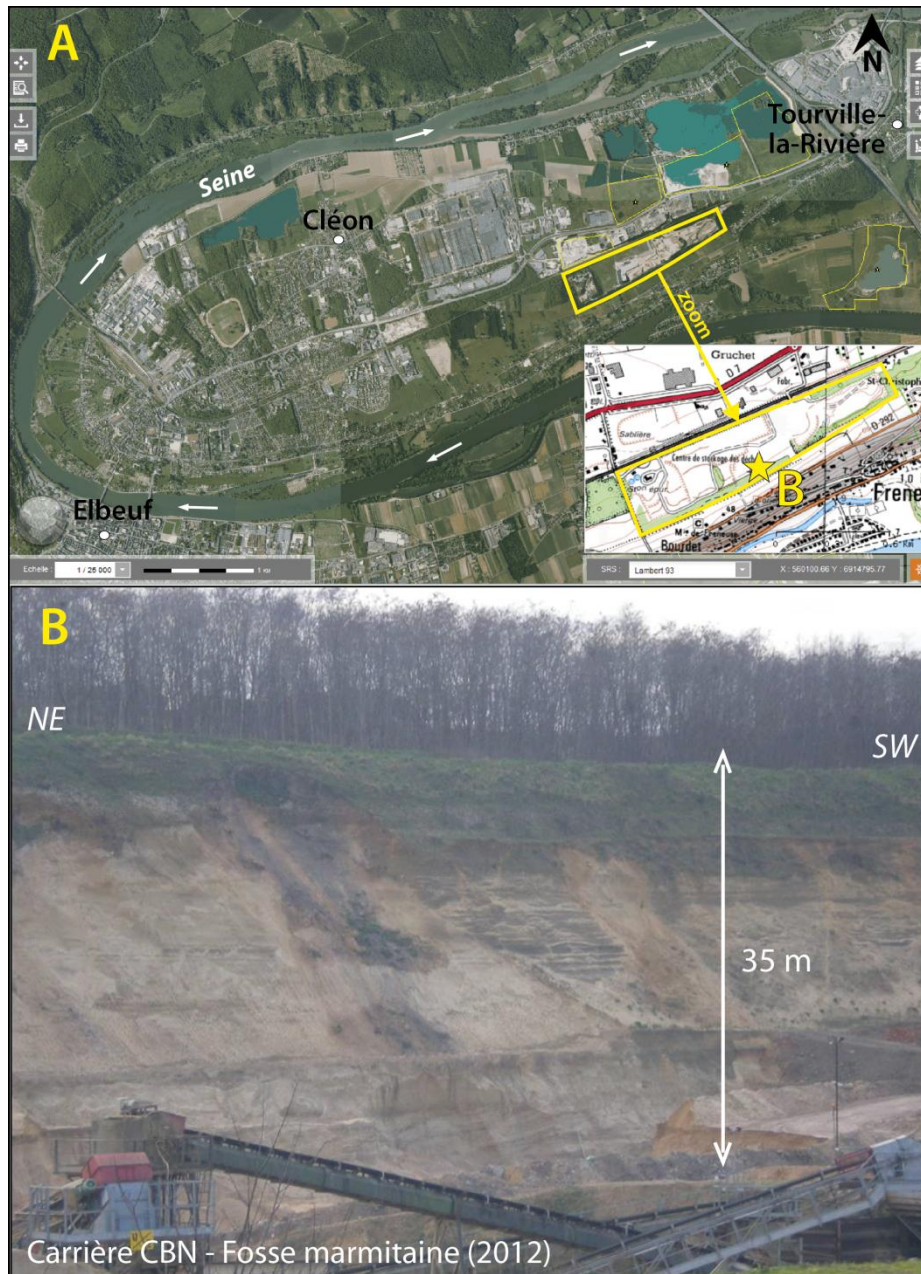
Figure III.25 Localisation du site d'étude. A: Orthophotographie du méandre d'Elbeuf avec localisation en jaune de la carrière CBN (d'après infoterre.brgm.fr), flèches blanches : écoulement actuel de la Seine, étoile jaune: front de taille. B: photographie du front de taille de la carrière étudiée (photo : Jamet, 2012)
