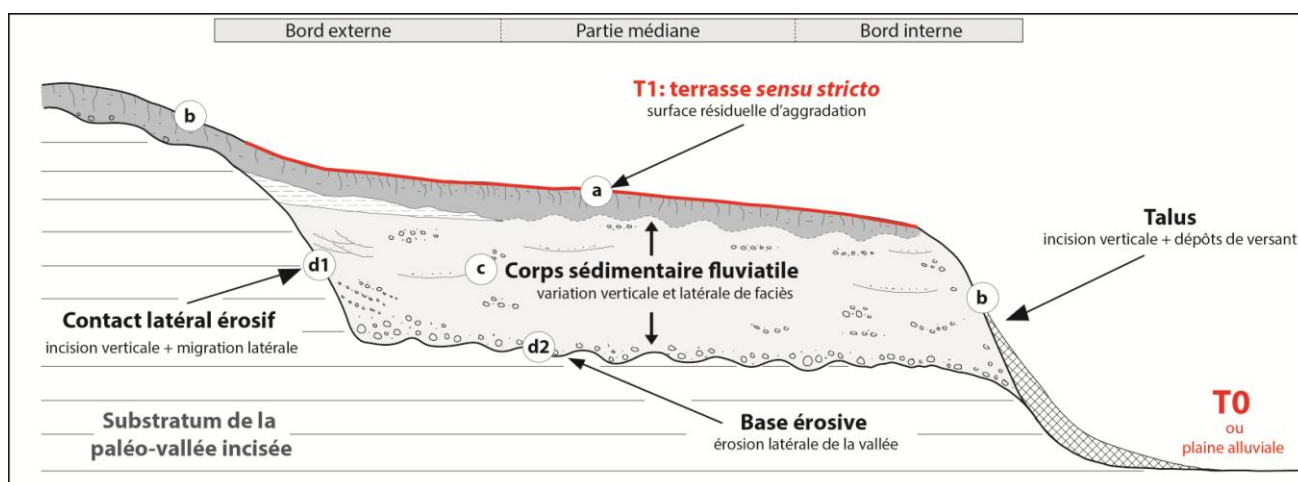
Figure II.26 Coupe transversale schématique d'une terrasse alluviale illustrant les éléments descriptifs géomorphologiques et sédimentaires (Connell et al. , 2007 modifié)
