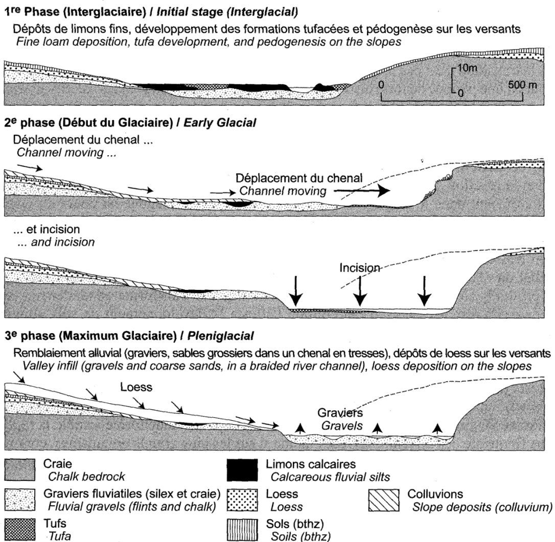
Figure II.28 Evolution synthétique de la formation des terrasses fluviatiles de la Somme (Antoine et al. , 2000)
