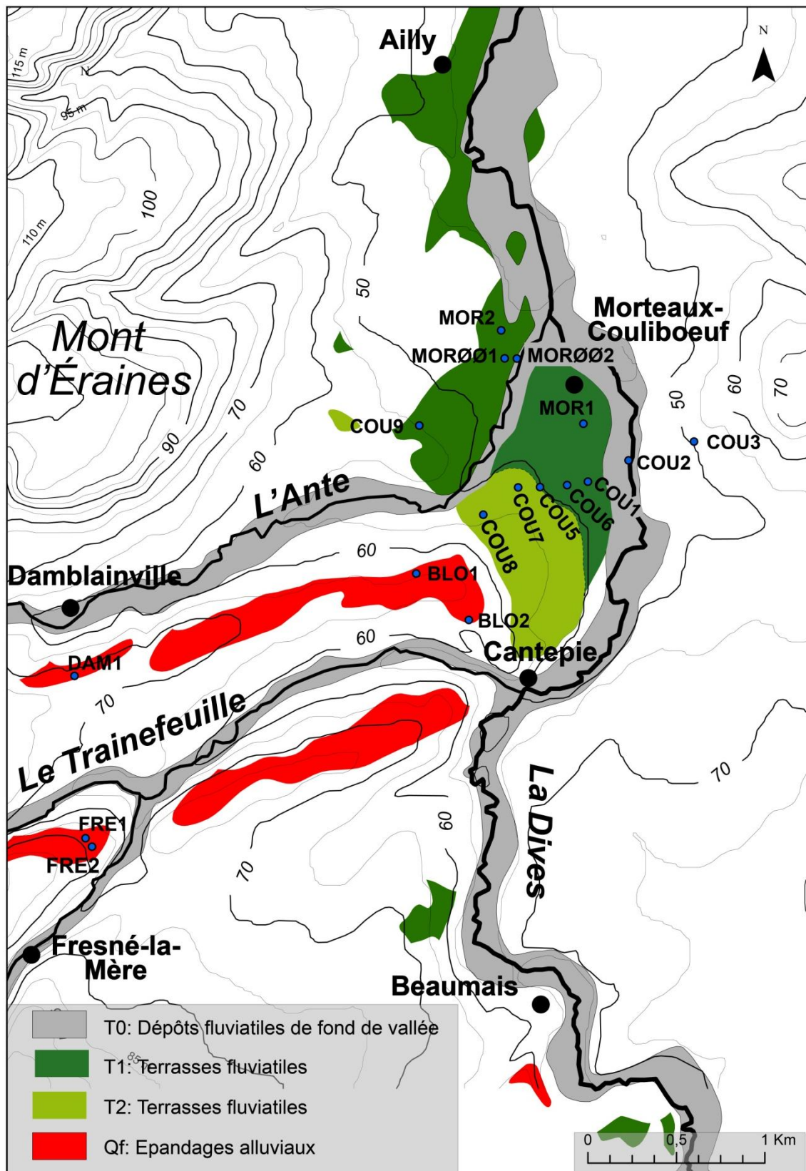
Figure III.84 Cartographie des dépôts fluviatiles du cours amont de la Dives, entre Courménéil et Morteaux-Couliboëuf
