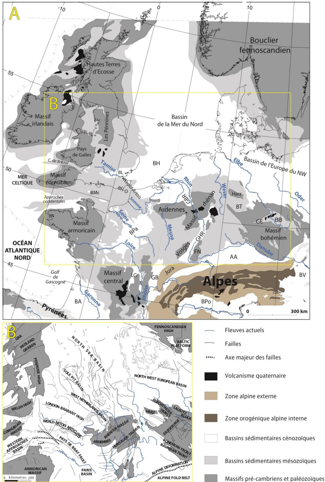
Figure 1.6 Le domaine NW-européen - A : Les grandes unités géologiques du NW de l'Europe (in Gijssels, 2006 modifié) Abréviations : BPa : Bassin de Paris, BMC : bassin de la Manche centrale, BL : bassin de Londres, BH-D : bassin du Hampshire et de Dieppe, BH : bassin hollandais occidental, GBR : Graben du bas-Rhin, GHR : Graben du Haut-Rhin, GL : Graben de Limagne, BG : Graben de la Bresse, FN : Forêt Noire, BA : bassin aquitain, BPo : Bassin du Pô, AA : avant fosse molassique alpine, BV : bassin viennois, BB : Bassin bohémien, GE : Graben d'Eger, BT : Bassin thuringien. B : Cadre structural cénozoïque du NW de l'Europe (Gibbard, 1988 modifié).
