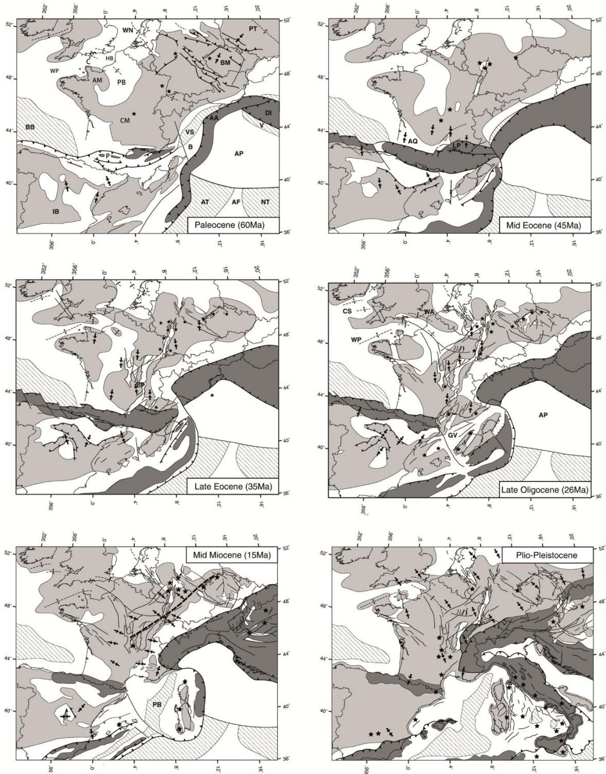
Figure I.1 Cartes paléogéographiques simplifiées de l'Europe du NW, au cours du Cénozoïque (d'après Ziegler & Dèzes, 2007 modifié). Légende: gris sombre : zone orogénique; gris clair : terres émergées; blanc : bassin sédimentaire / plate-forme marine ; blanc hachuré: bassins océaniques ; étoile : zone volcanique ; flèche: direction de compression horizontale maximum ; tracé pointillé épais: axe de faille lithosphérique.
