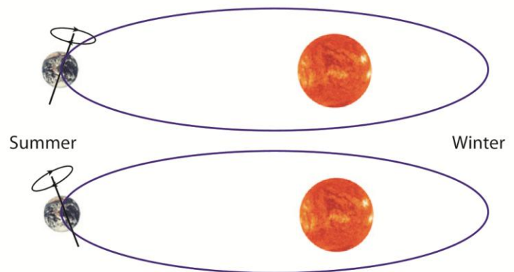
Figure I.18 Cycles orbitaux régulant l'insolation de la Terre (Nisancioglu, 2009)
