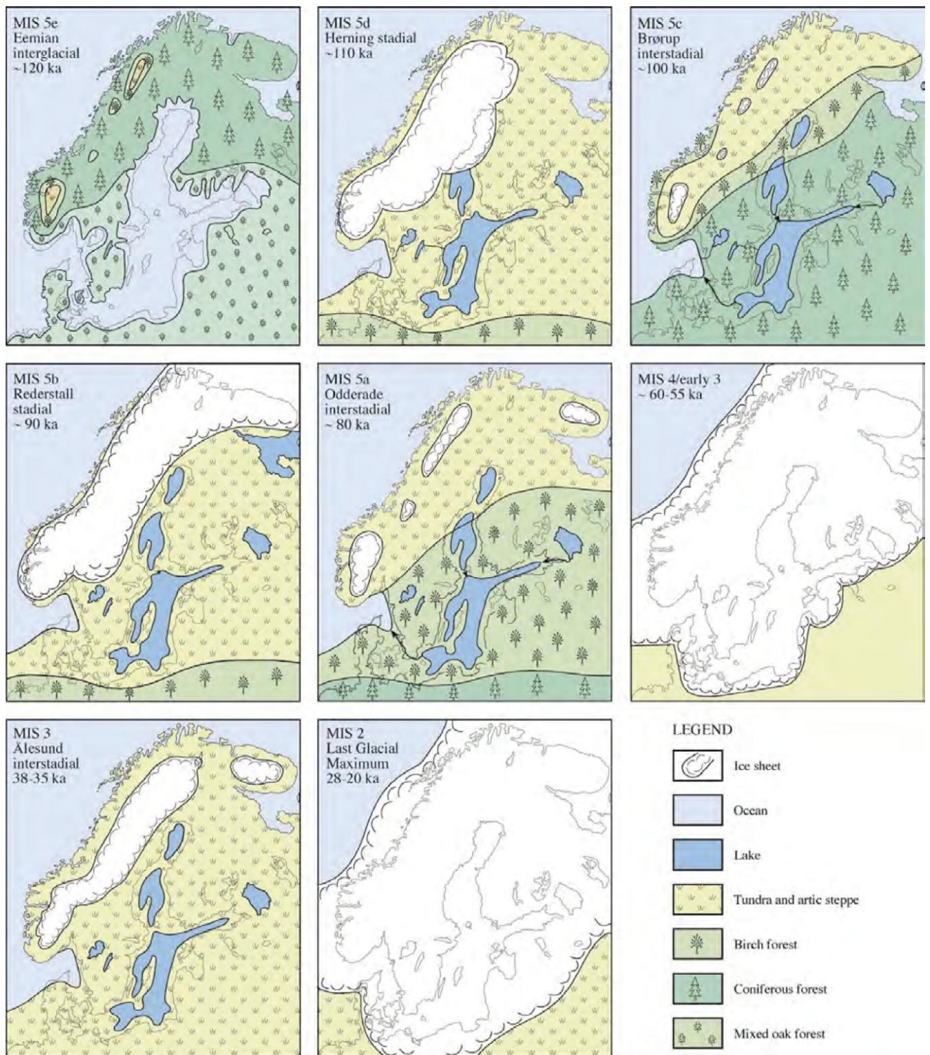
Figure I.15 Développement de la calotte glaciaire scandinave et des environnements associés en Europe du Nord à partir du dernier interglaciaire (Éémien, MIS 5e) et jusqu'au dernier maximum glaciaire (Weichsélien, MIS 2) (Mangerud, 2004).
