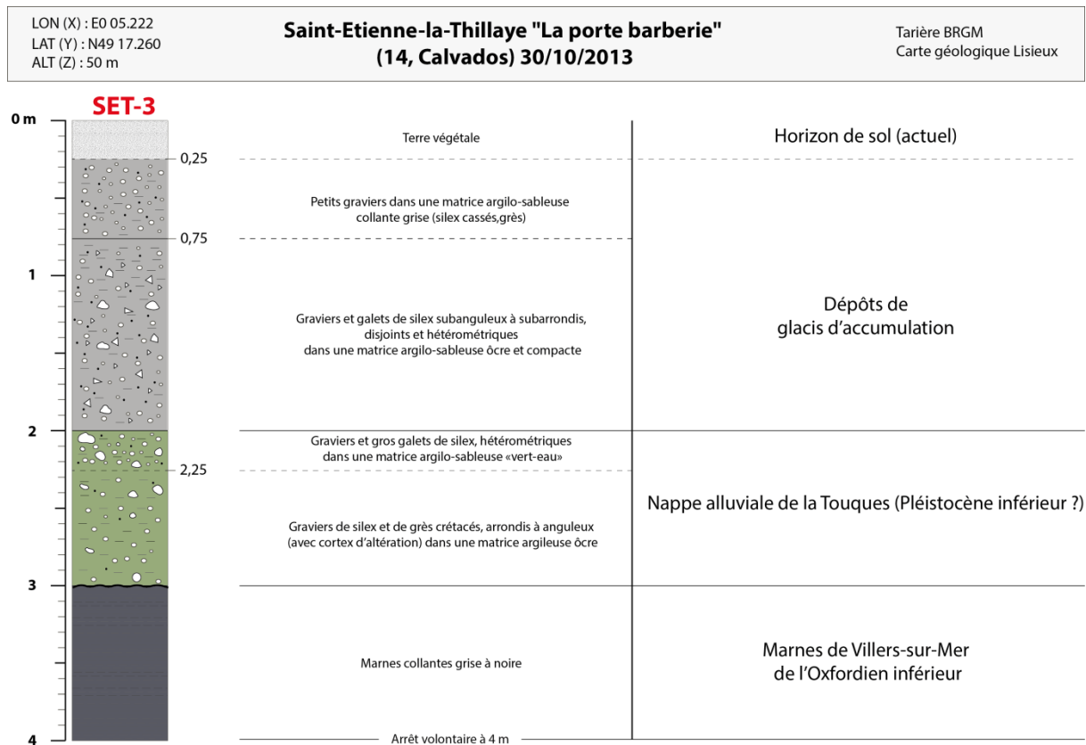
Figure III.63 Coupe stratigraphique du forage de la nappe de Saint-Etienne-la-Thillaye (SET-3)
