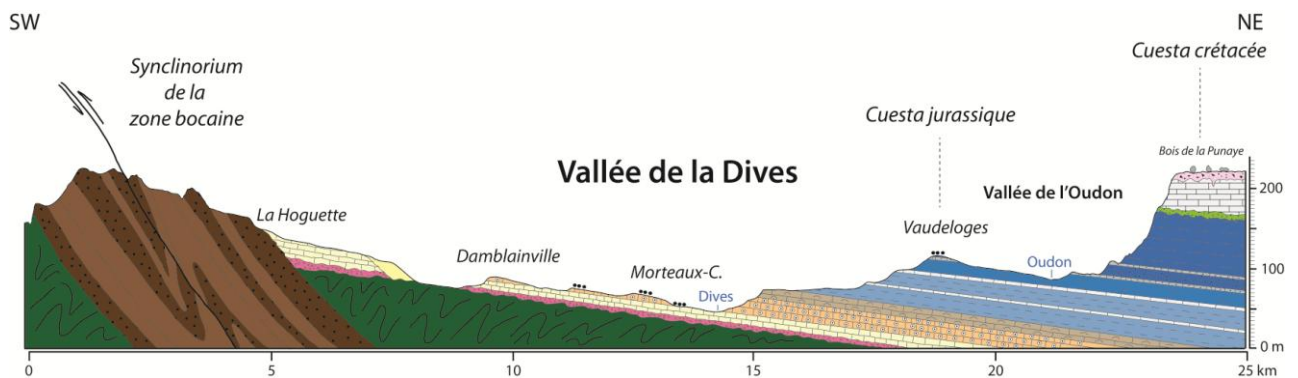
Figure III.82 Coupe transversale SW-NE de la vallée de la Dives, à Morteaux-Coulibœuf
