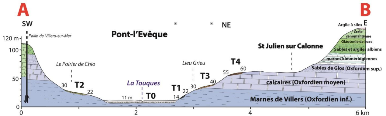
Figure III.61 Cartographie des terrasses fluviales étagées (T0 à T4) dans le secteur de Pont-l'Évêque et profil transversal (A-B) de la vallée de la Touques en relation avec la géologie du substratum (légende cf. Figure III.54)
