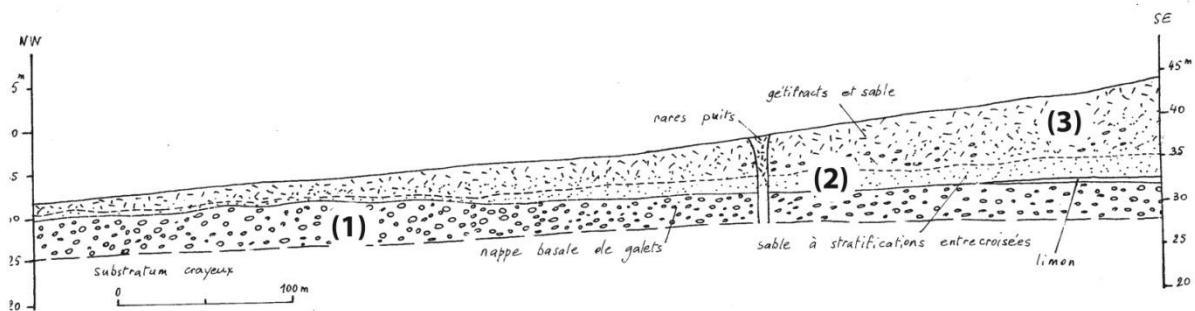
Figure III.44 Coupe transversale synthétique NW-SE de la terrasse de Saint-Pierre-lès-Elbeuf aux Fiefs Mancels (Lefébvre et al. , 1986)
