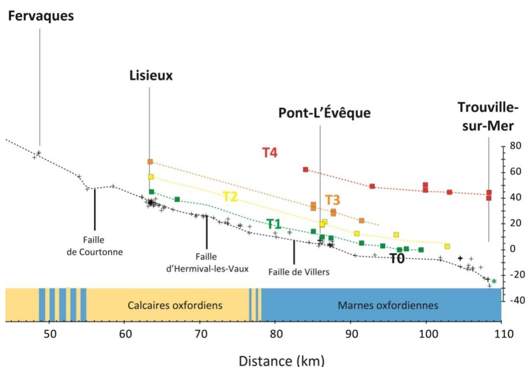
Figure III.72 Profils longitudinaux des terrasses fluviales (T0 à T4) de la Touques, entre Fervaques et Trouville-sur-Mer (environ 60 km)
