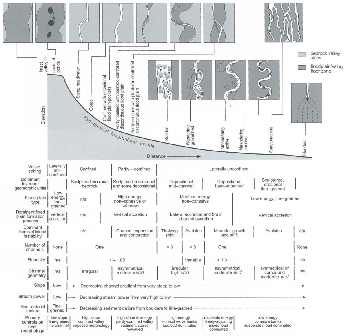
Figure II.2 Profil longitudinal théorique présentant l'évolution amont-aval des styles fluviaux et des paramètres morphologiques (in Fryirs & Brierley, 2013)
