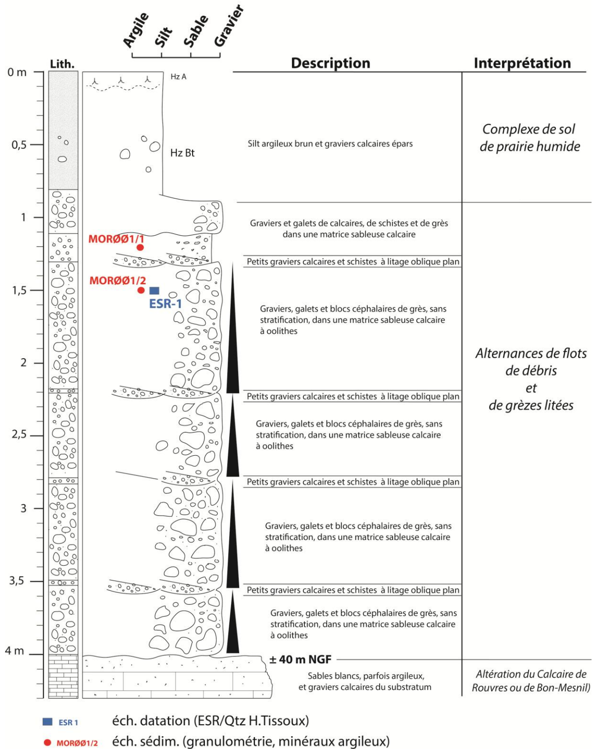
Figure III.87 Coupe sédimentologique de la terrasse T1 à Morteaux-Couliboef
