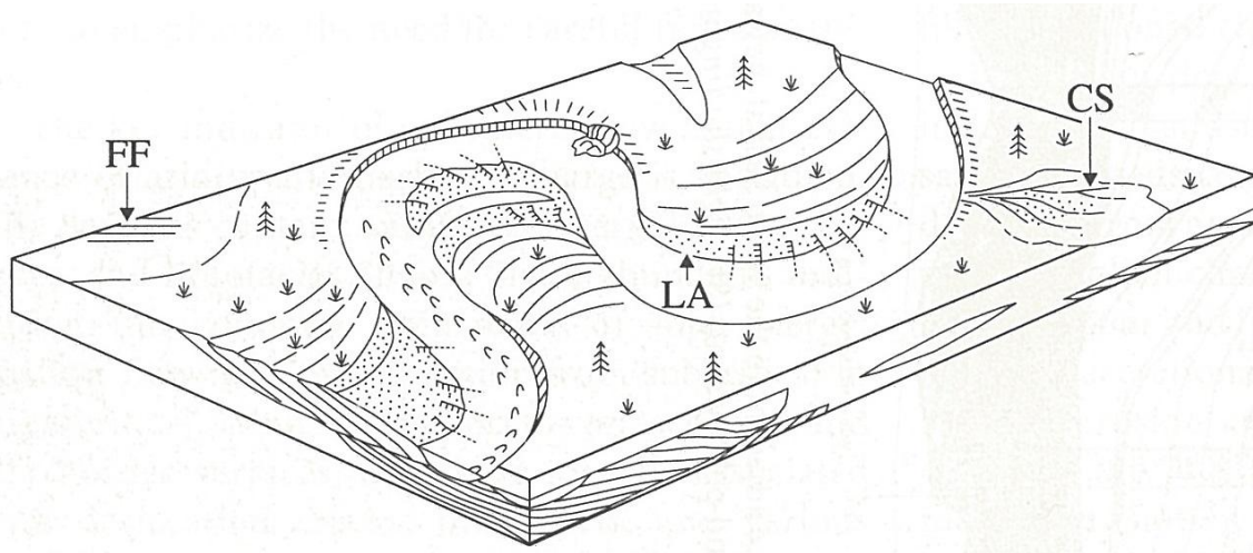
Figure II.19 Modèle de faciès de rivière sableuse méandrique (Miall, 1996). LA : accrétion latérale ( Lateral accretion ), CS : lobe de crevasse ( Crevasse splay ) et FF : dépôts de berge, de marécages ou de plaine d'inondation ( Floodplain fines )
