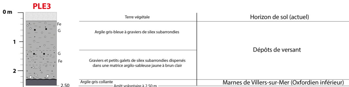
Figure III.66 Coupe stratigraphique du forage de la nappe résiduelle du Lieu Lesniès à Pont-l'Évêque (PLE3)
