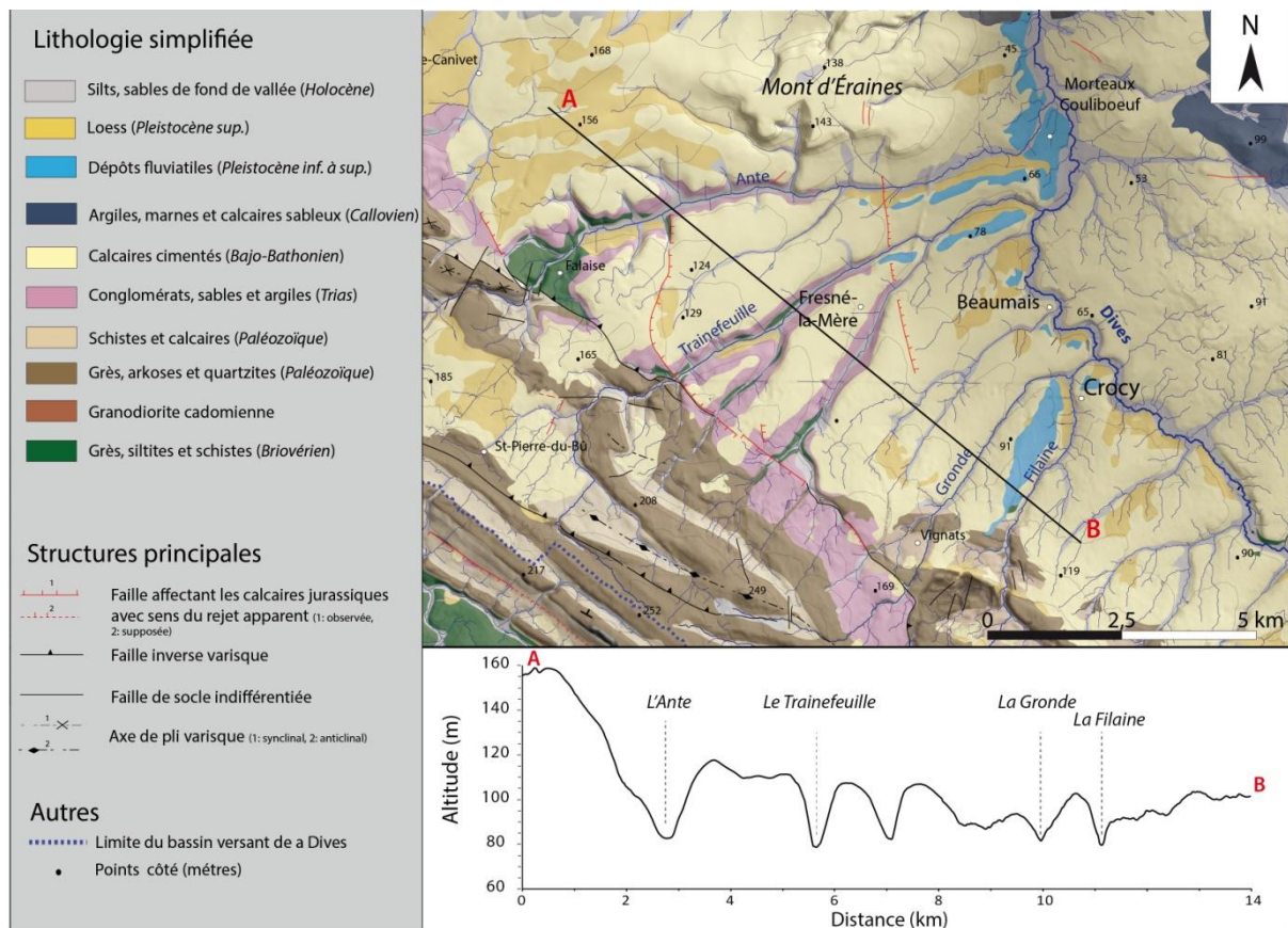
Figure III.80 Carte géologique simplifiée (d'après Gigot et al. , 1999 modifié) au contact de la zone bocaine et de la plaine calcaire de Trun-Falaise, représentant le réseau des talwegs, entre Falaise et Morteaux-Couliboëuf. Coupe AB : profil topographique transversal NW-SE des affluents de la rive gauche de la Dives moyenne.
