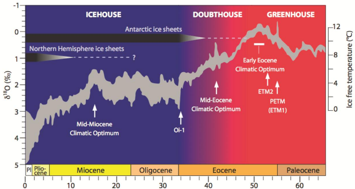
Figure 1.3 Évolution du \delta^{18}\text{O} des foraminifères benthiques au Cénozoïque et représentation des tendances climatiques (Greenhouse/Icehouse) (Zachos et al. , 2008 in Huyghe, 2010).
