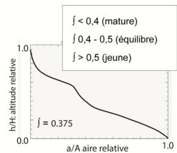
Figure 6. Exemples de différents descripteurs géomorphométriques pour l'analyse du relief et du drainage des bassins versants
