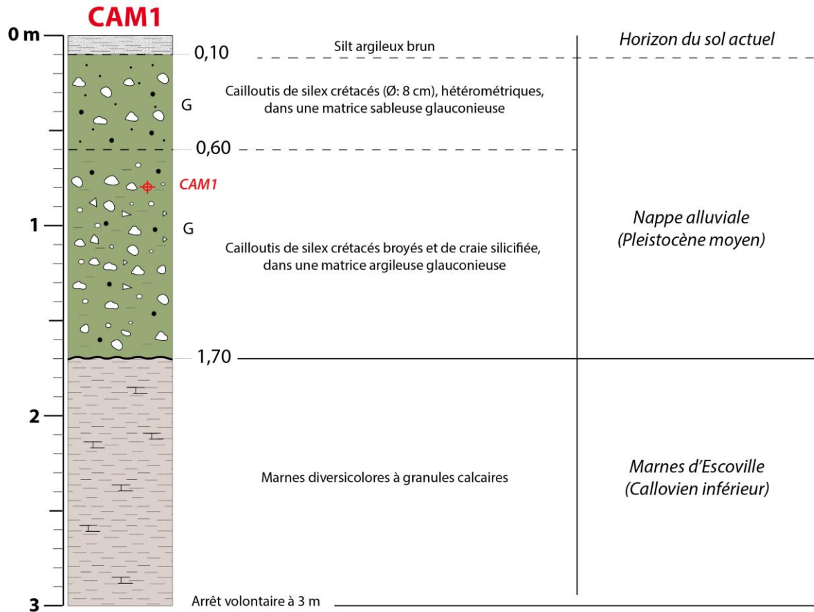
Figure III.92 Coupe stratigraphique du forage CAM1 dans la nappe alluviale T3 au lieu dit «les Campigny »
