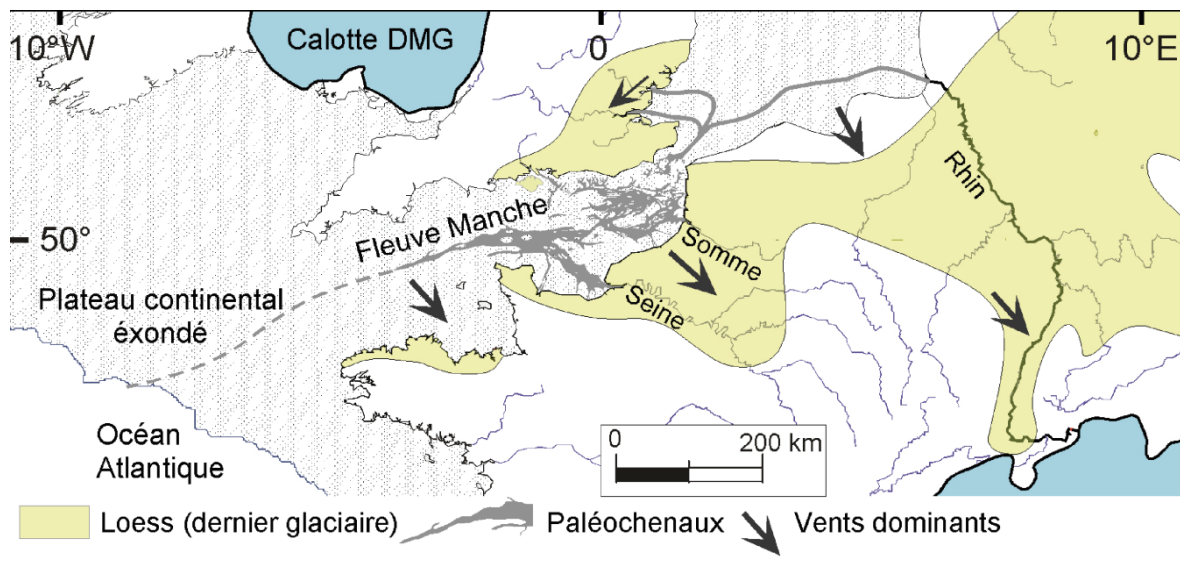
Figure I.14 Extension simplifiée des lœss NW-européens au cours du Weichsélien (Antoine, comm. pers. ) Légende : DMG calotte du dernier maximum glaciaire, tracés des paléochenaux (d'après Auffret et al. , 1982)
