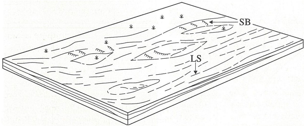
Figure II.22 Modèle de faciès de rivière sableuse à écoulements évènementiels (Miall, 1996). SB : barres sableuses ( Sand bars ) et LS : nappes sableuses à litages horizontaux ( Laminated Sand Sheets )
