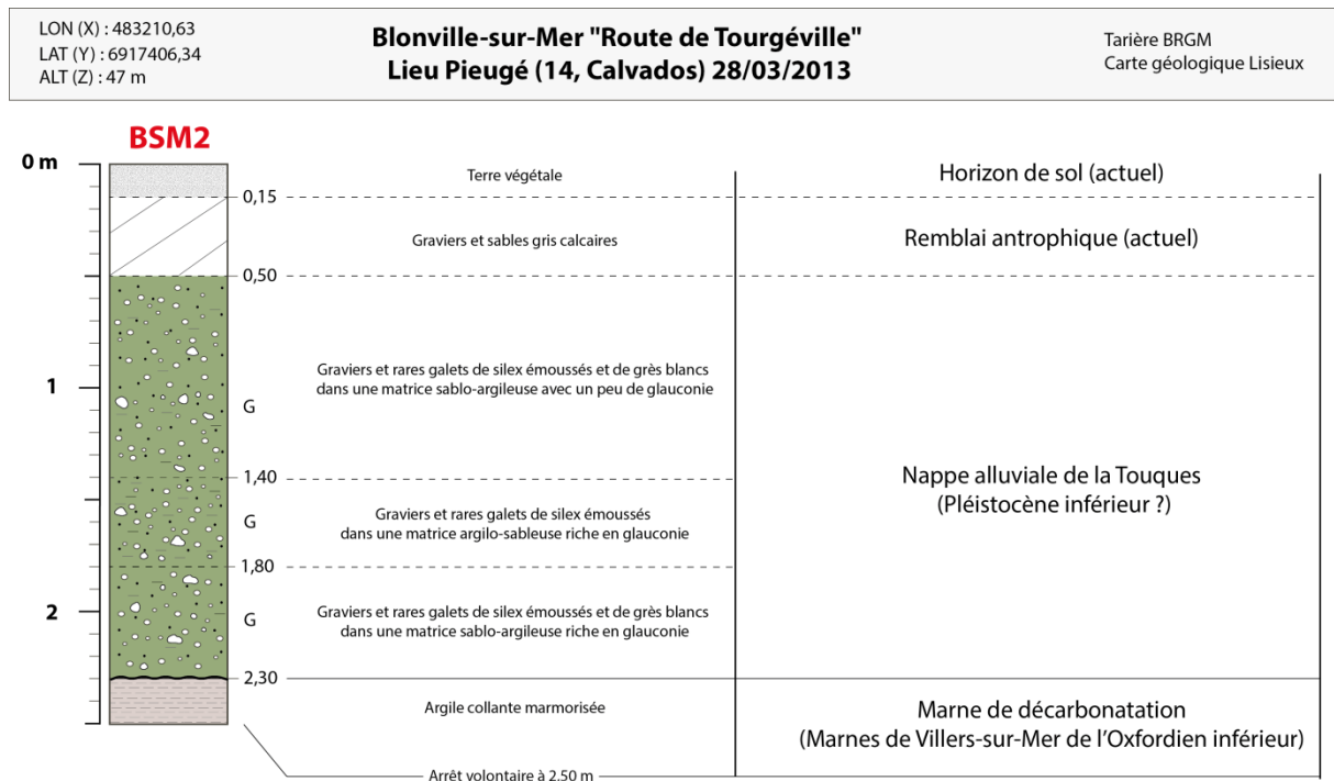
Figure III.64 Coupe stratigraphique du forage de la nappe de Blonville-sur-Mer (BSM2)
