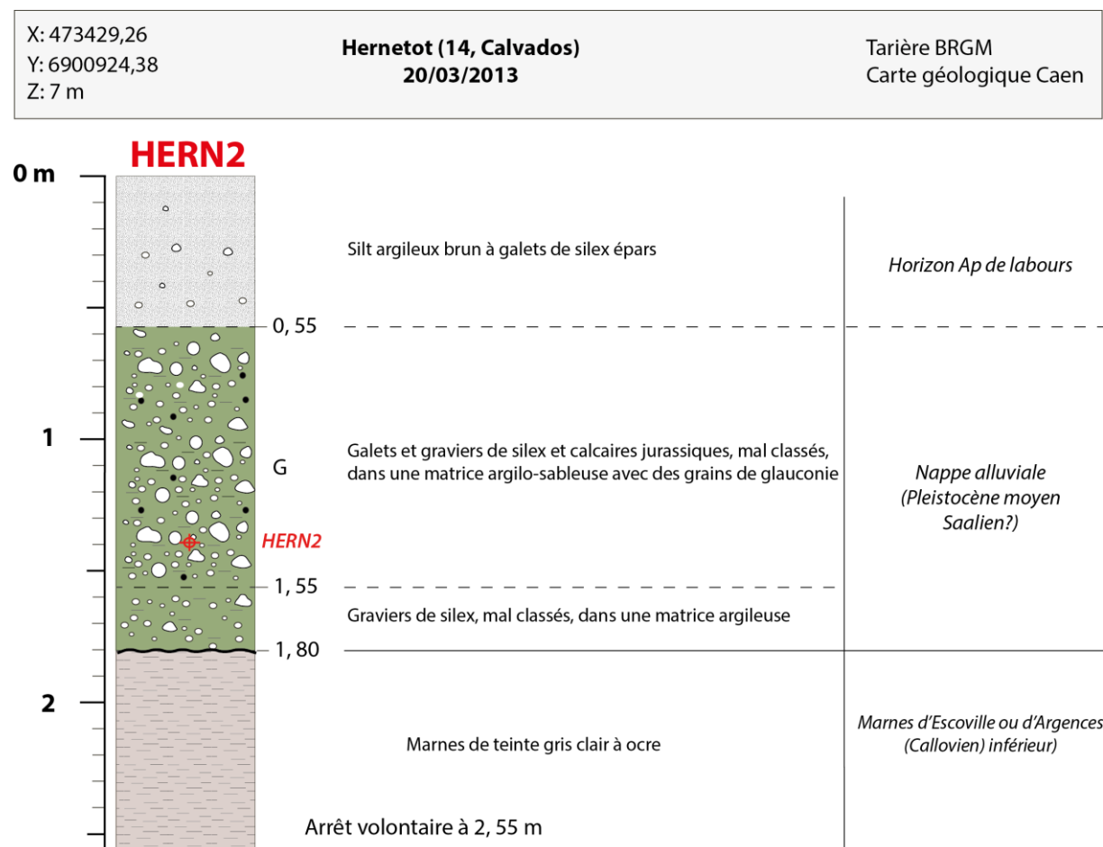
Figure III.107 Coupe stratigraphique du forage HERN2 dans la nappe alluviale de Hernetôt à proximité de Cléville
