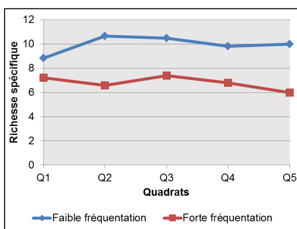
Figure 45. Richesse spécifique en fonction des quadrats (campagne 2013)
