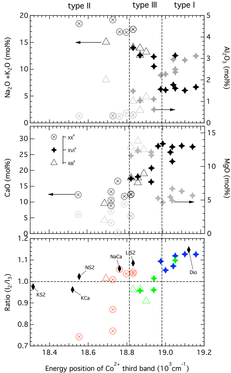
FIGURE 6.5 – (haut) Composition molaire totale en alcalins \text{Na}_2\text{O}+\text{K}_2\text{O} (noir, ordonnée de gauche) et en \text{Al}_2\text{O}_3 (gris, ordonnée de droite) en fonction de la position en énergie de la troisième bande du \text{Co}^{2+} . (milieu) Composition molaire en \text{CaO} (noir, ordonnée de gauche) et \text{MgO} (gris, ordonnée de droite) en fonction de la position de la troisième bande du \text{Co}^{2+} . (bas) Ratio entre l'intensité de la bande à 15\,500\text{ cm}^{-1} et la bande à 16\,800\text{ cm}^{-1} en fonction de la position de la troisième bande. La forme des marqueurs indique l'époque des échantillons. La couleur indique le type de verre défini selon les critères de composition chimique : type I (HLLA, bleu), type II (sodique, rouge), type III (potassique, vert). Les résultats sont comparés à ceux des verres modèles (diamants noirs) de composition simplifiée étudiés au chapitre 5.
