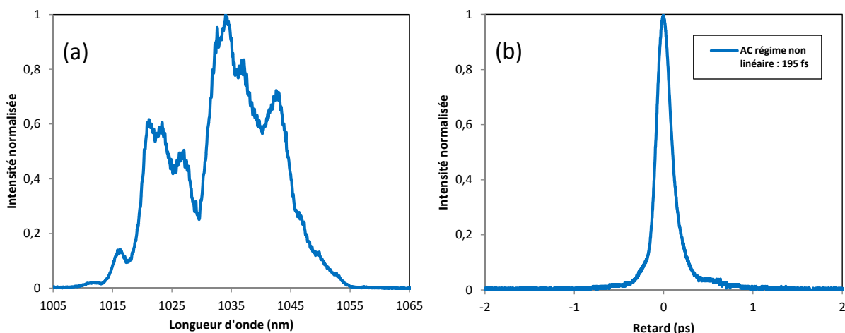
FIGURE III-18 : (a) Spectre et (b) trace d'autocorrélation de l'impulsion recombinaisonnée après mise en phase des canaux spectraux pour un régime d'amplification non-linéaire.
