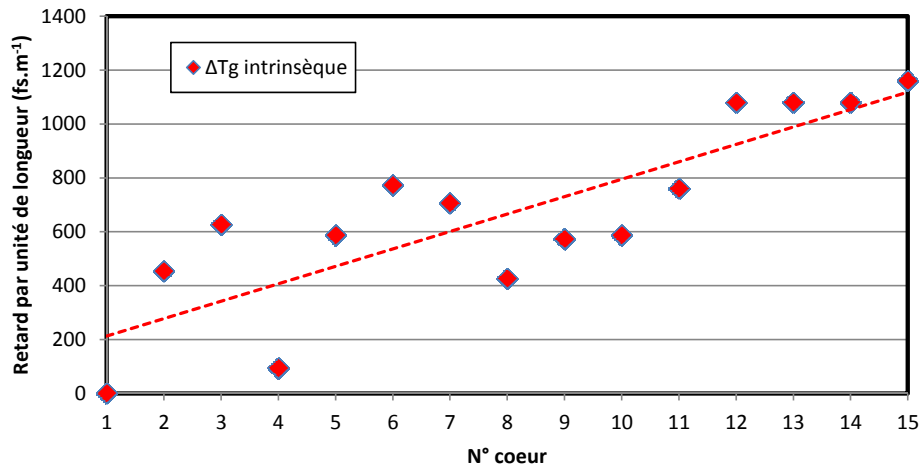
FIGURE III-2 : Différences de temps de groupe entre cœurs mesurées par rapport au cœur numéro 1 de la fibre à 15 cœurs espacés de 24 \mu\text{m} . Les douze cœurs successifs permettant d'atteindre un écart-type de temps de groupe minimal (260 fs) sont pris entre les cœurs numéro 2 et 13.
