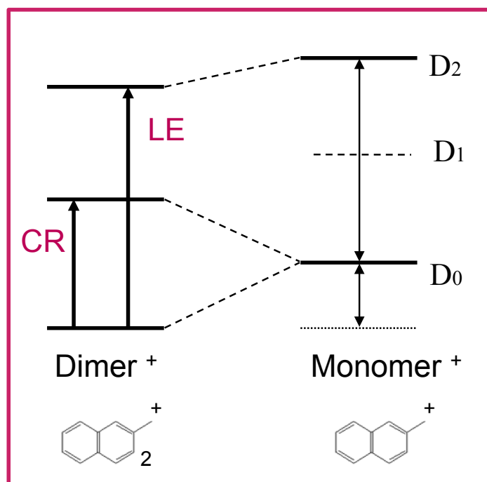
FIGURE 1.10: Schéma de niveaux qualitatif des premiers états électroniques d'un cation PAH + et du dimère cation (PAH) 2 + correspondant.
