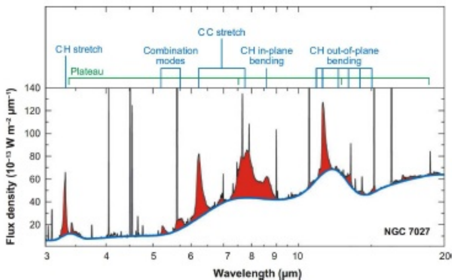
FIGURE 1.7: Spectre d'émission dans l'infrarouge moyen de la source NGC 7027. Les AIBs, renforcées en rouge, s'inscrivent sur un continuum dû à la phase solide (grains). L'identification des modes aromatiques est indiquée dans la partie supérieure de la figure [Tielens, 2008].
