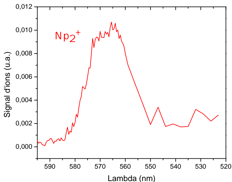
FIGURE 4.9: Spectre visible du cation dimère Naphtalène.
