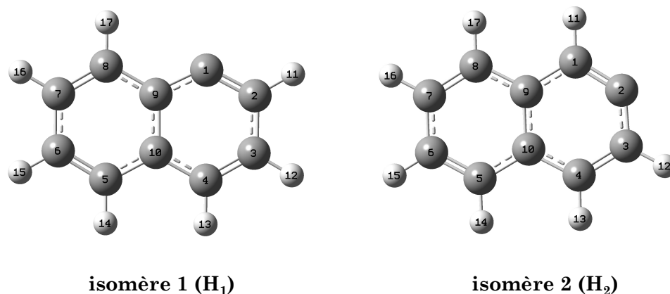
FIGURE 2.2: Structures des isomères H_1 et H_2 du naphthalène une fois déshydrogéné.
