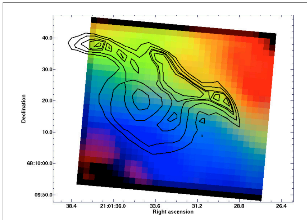
FIGURE 1.9: Carte de l'objet NGC 7023-North West : les spectres attribués aux PAH + (en bleu), PAH (en vert) et VSG (en rouge) se succèdent sans coïncider [Berné et al., 2007].
