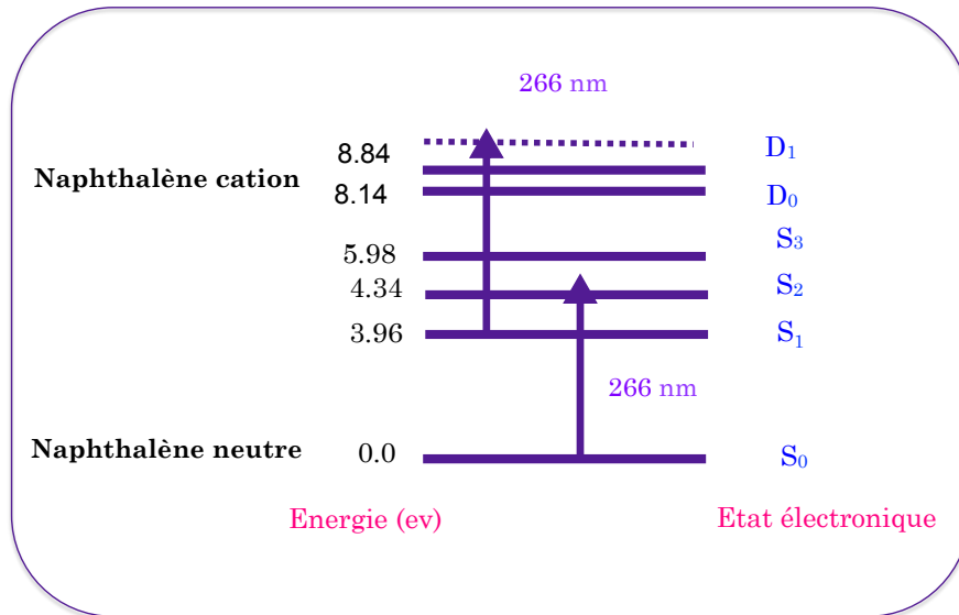
FIGURE 3.5: Etat électronique, énergie et nombre de photons absorbés au cours de la photoionisation UV à 266 nm de l'espèce Naphthalène.
