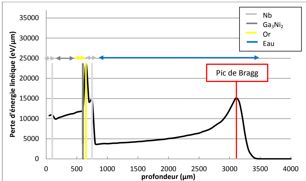
Figure 4.8- Perte d'énergie linéique de protons de 23 MeV dans une cible composée de 100 μm de niobium (Nb), 520 μm de Ga 3 Ni 2 et 50 μm d'or. Le pic de Bragg se trouve à 3 mm de profondeur dans l'eau de refroidissement
