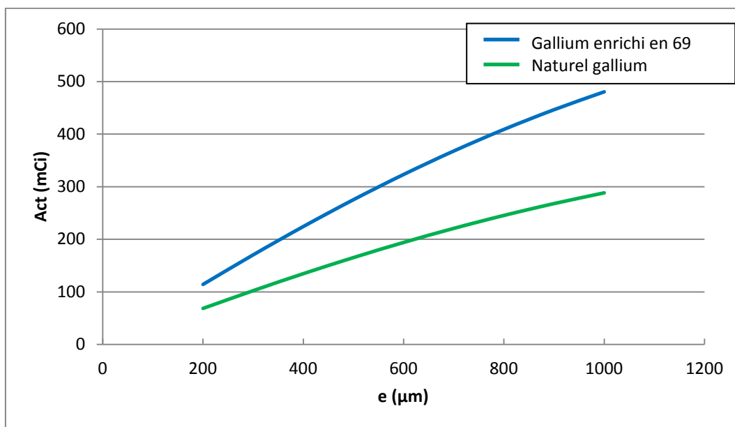
Figure 4.2- Activités de 68 Ga en fonction de l'épaisseur de l'alliage de Ga 3 Ni 2 . La courbe bleue correspond à l'activité calculée à partir de la cible contenant du gallium enrichi en 69 tandis que la courbe verte a été calculée à partir du gallium naturel
