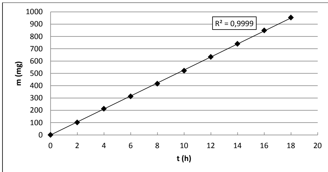
Figure 3.15- Courbe d'étalonnage de la masse de dépôts en fonction de la durée d'électrodeposition. Le coefficient de détermination de la droite de régression linéaire a été déterminé
