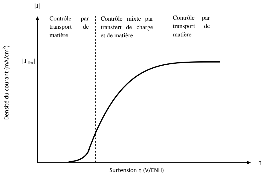
Figure 2.2- Morphologie d'une courbe intensité/potentiel associée à un système irréversible limité par la diffusion
