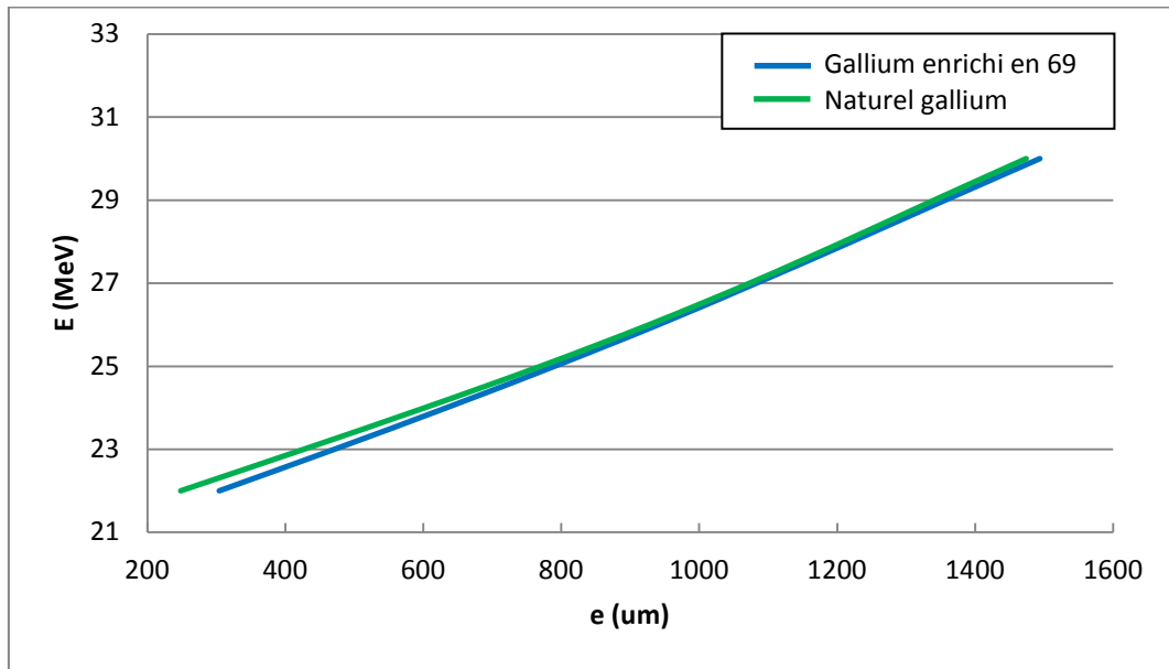
Figure 4.5- Épaisseur de l'alliage de Ga_3Ni_2 en fonction de l'énergie d'entrée du faisceau de protons
