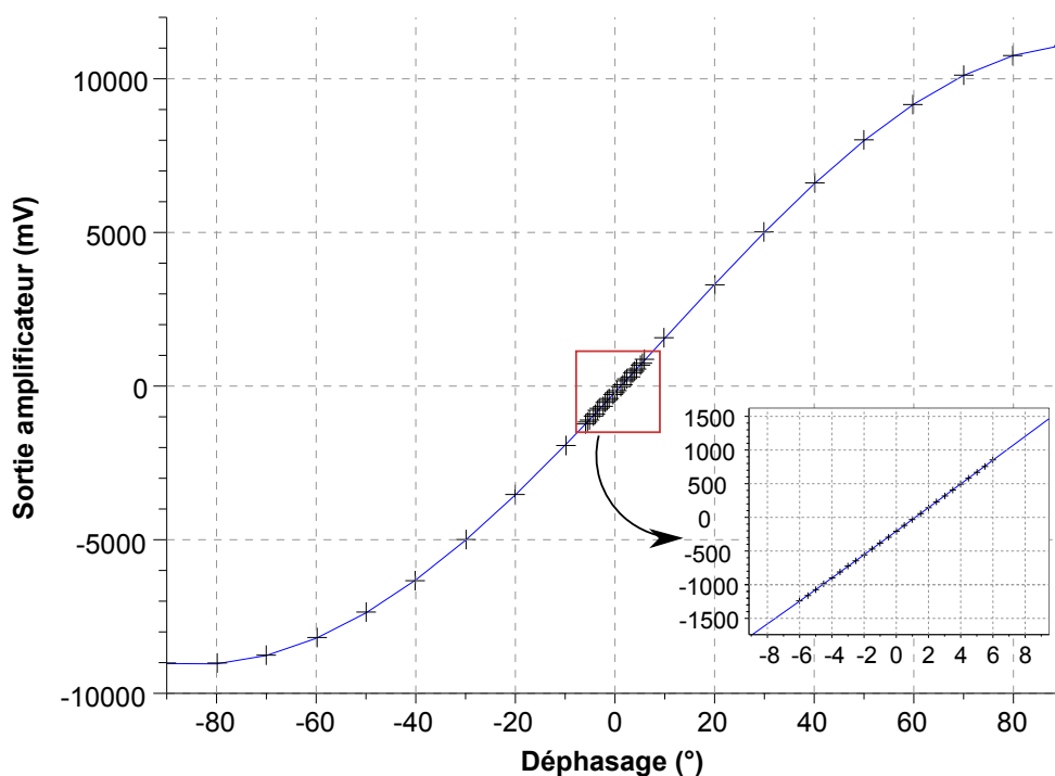
FIGURE 3.22 – Courbe mesurée de sensibilité du mélangeur.
