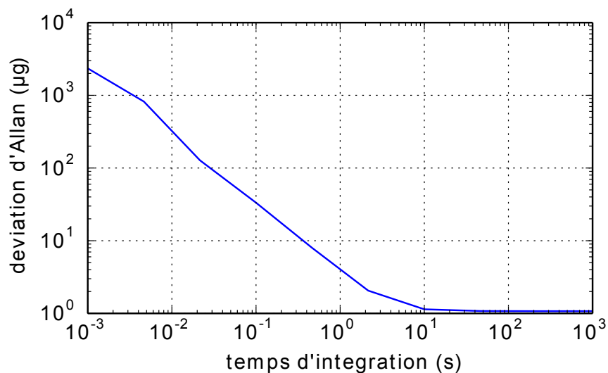
FIGURE 4.5 – Résolution accélérométrique pour un capteur MEMS de type VIA.
