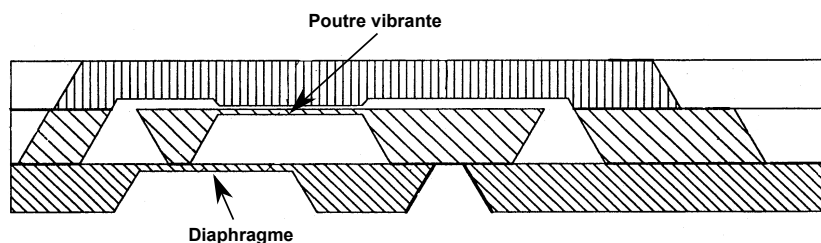
FIGURE 1.8 – Représentation du capteur de pression breveté par Thalès.
