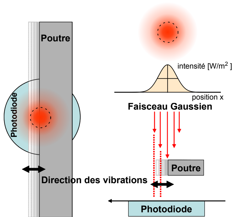
FIGURE 2.15 – Détection par obscuration du faisceau.
