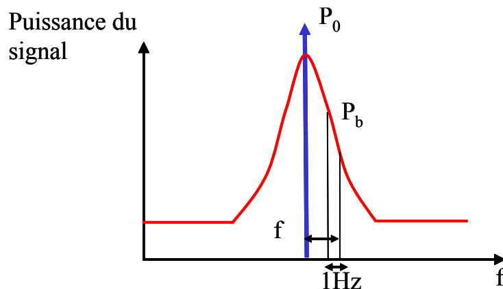
FIGURE 1.15 – Représentation du spectre de l'oscillateur.
