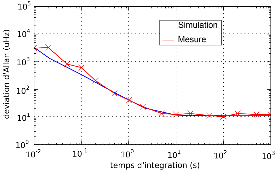
FIGURE 3.30 – Superposition de la déviation d'Allan mesurée et simulée pour la cellule VIA.
