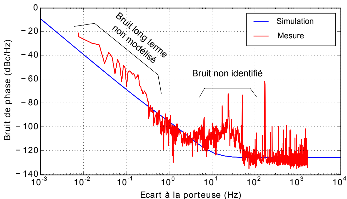
FIGURE 3.28 – Superposition du bruit de phase mesuré et simulé pour la cellule VIA.
