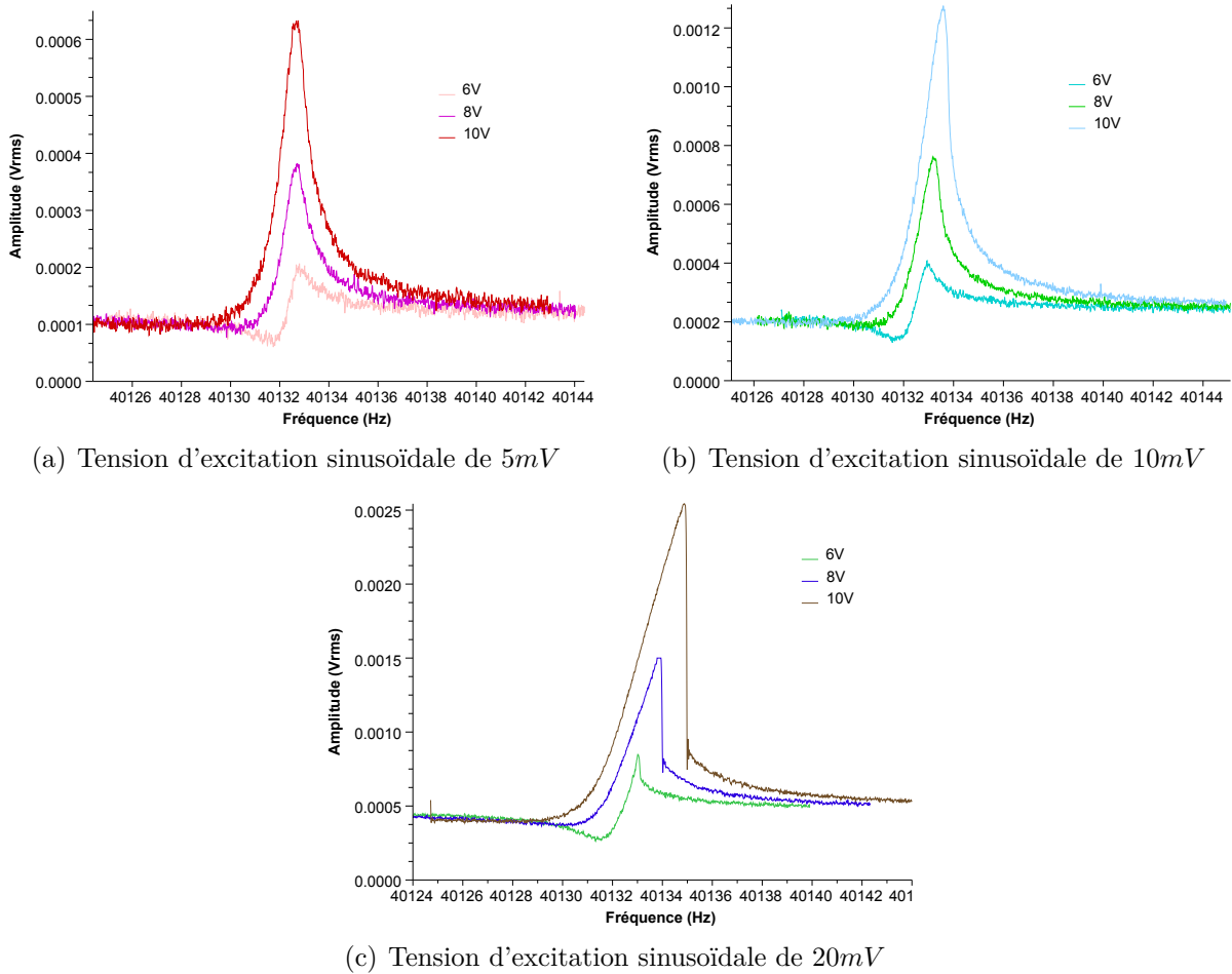
FIGURE 3.12 – Mesure de la réponse de la cellule pour différents niveaux d'excitation.
