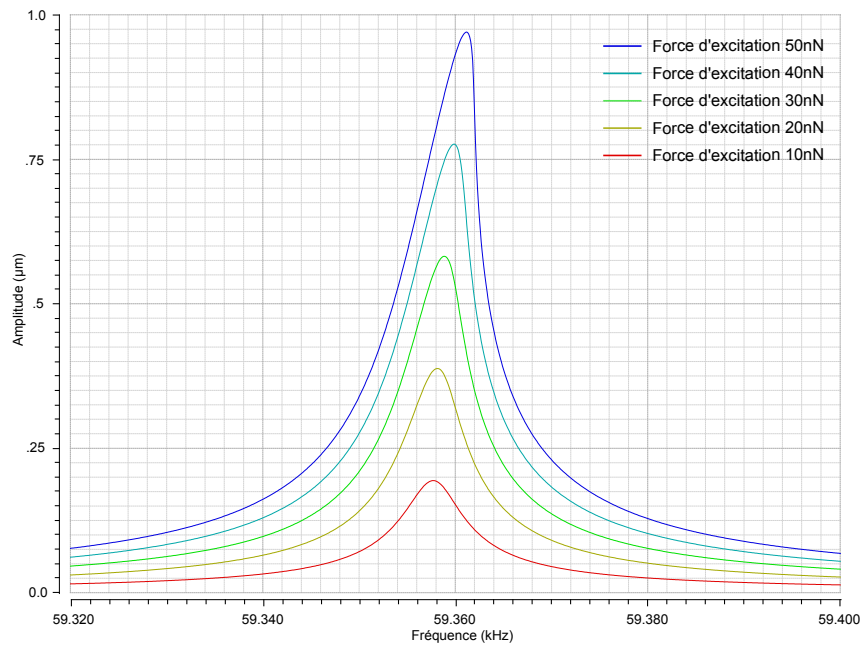
(a) Amplitude du résonateur
