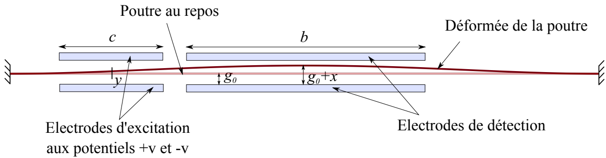
FIGURE 2.13 – Schéma de la poutre vibrante avec les électrodes d'excitation et de détection.
