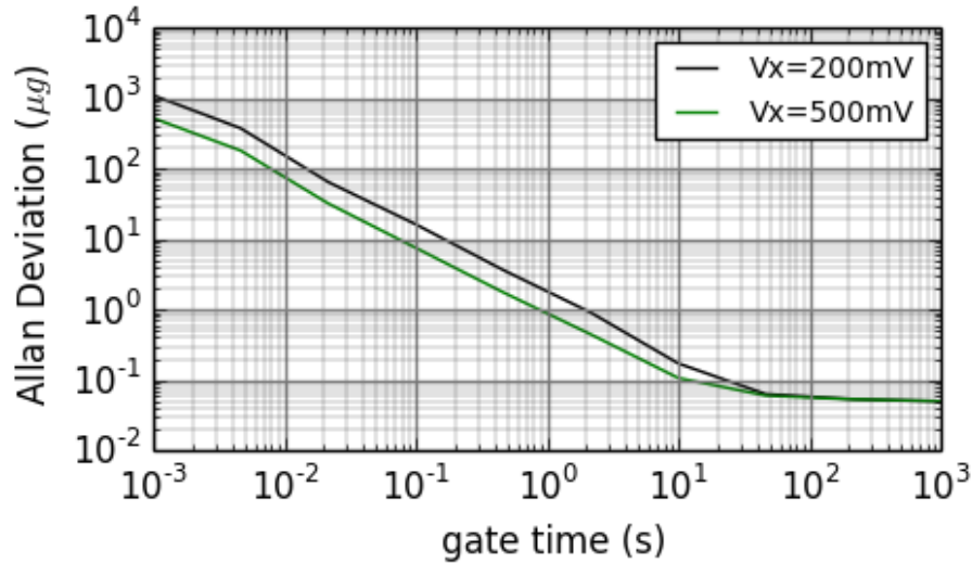
FIGURE 4.11 – Deviation d'Allan en accélération d'un VIA dans la zone linéaire et suivant différentes amplitudes d'excitation.
