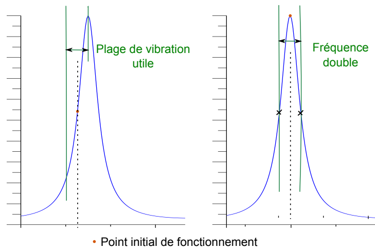
FIGURE 2.20 – Influence de la position du point de fonctionnement pour la détection par interférométrie.
