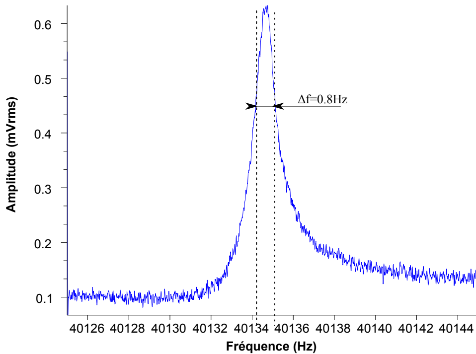
FIGURE 3.9 – Courbe expérimentale de la résonance de la cellule Aladin pour une excitation de 5mVp et 7V de polarisation
