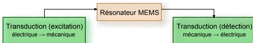
FIGURE 2.7 – Schéma représentant la transduction : l'excitation et la détection d'un résonateur.
