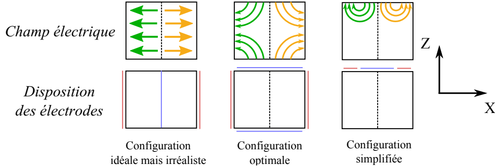
FIGURE 2.10 – Configurations d'électrodes pour la détection et l'excitation de la flexion pour le quartz (poutre vue en section).
