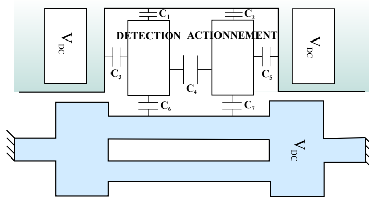
FIGURE 3.10 – Disposition des capacités parasites entre l'actionnement et la détection.
