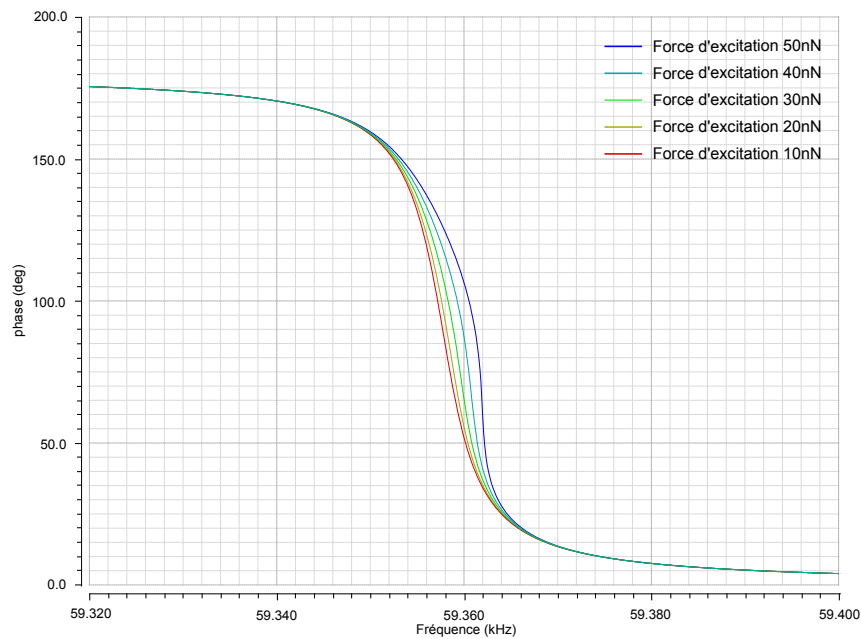
(b) Phase du résonateur
