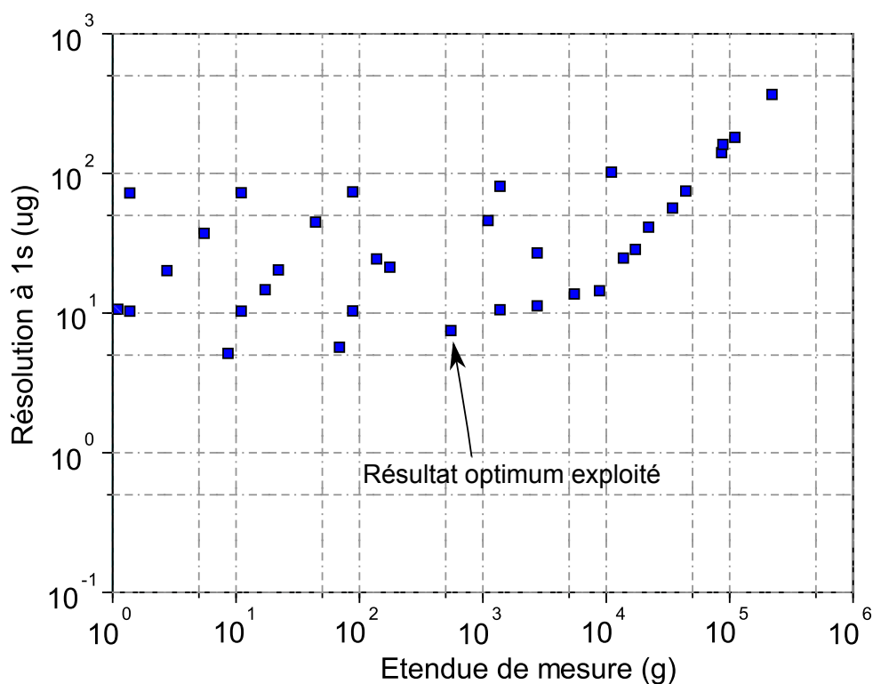
FIGURE 4.7 – Résolution des différents types de résonateur en fonction de l'étendue de mesure et pour épaisseur vibrante supérieure à 50\mu m
