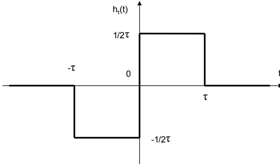
FIGURE 1.16 – Réponse impulsionnelle de la variance d'Allan.
