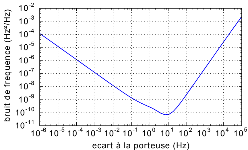
FIGURE 4.4 – Simulation du bruit de fréquence pour un capteur MEMS de type VIA
