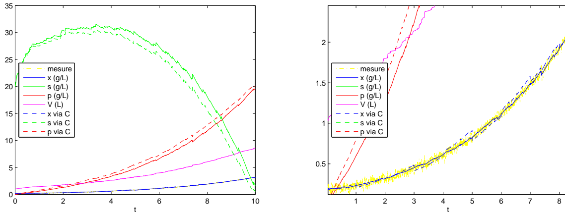
FIG. 8.15 – C(y) en présence de bruit ( \sigma = 0.1 ) avec modification de modèle toutes les heures.
