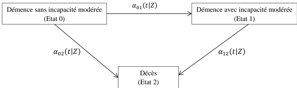
Figure 15 : Représentation graphique du modèle multi-état, où \alpha_{01}(t|Z) , \alpha_{02}(t|Z) , \alpha_{12}(t|Z) sont les intensités de transition.
