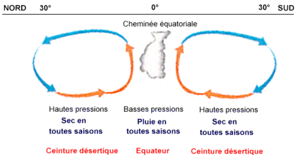
FIGURE 9 : COUPE MERIDIIONALE (NORD-SUD) DU MECANISME DES CELLULES DE HADLEY. DE PART ET D'AUTRE DE L'EQUATEUR UN TRANSPORT VERTICAL DES MASSES D'AIR CHAUDES ET HUMIDES EST REALISE VERS LATITUDES \pm 30^\circ . L'AIR PLUS FROID DE CES LATITUDES EST ENSUITE TRANSPORTE VERS L'EQUATEUR. LA POSITION DES ZONES DE SUBSIDENCE ET D'ASCENDANCE VARIENT AU COURS DU TEMPS. IL S'AGIT ICI D'UN SCHEMA PRESENTANT L'ETAT MOYEN. (SOURCE : IFREMER)
