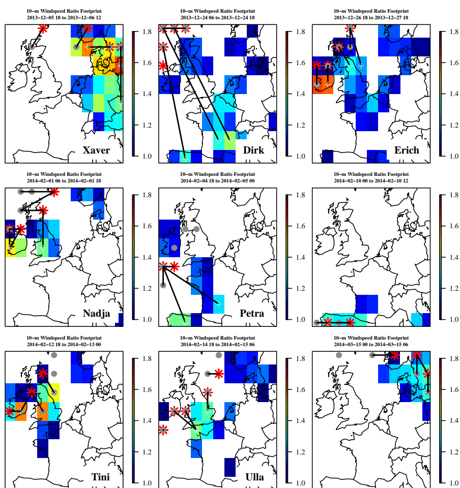
FIGURE 66 : CARTES DES 9 EVENEMENTS DETECTES AU COURS DE L'HIVER 2013-2014. LES POINTS GRIS INDIQUENT LES CENTRES DE VORTICITE RELATIVE, LES ETOILES ROUGES LES CENTRES D'ANOMALIE DE PRESSION ET LES CROIX BLANCHES LES CENTRES DU RATIO DE VENT. LES CENTRES DES TROIS VARIABLES SURVENANT AU MEME PAS DE TEMPS SONT LIES PAR UNE LIGNE NOIRE.
