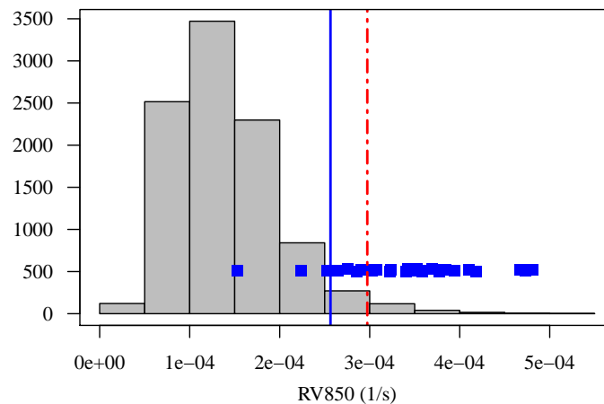
FIGURE 21 : HISTOGRAMME DES MAXIMA DE VORTICITE RELATIVE A 850 hPa DETECTES SUR LA PERIODE HIVERNALE CONSIDEREE. LES POINTS INDIQUENT LES VALEURS PRISES AU MOMENT DES NEUF EVENEMENTS. LE TRAIT PLEIN BLEU INDIQUE LE 96 E PERCENTILE DE LA DISTRIBUTION ET LE TRAIT TIRETE ROUGE INDIQUE LE 98 E PERCENTILE.
