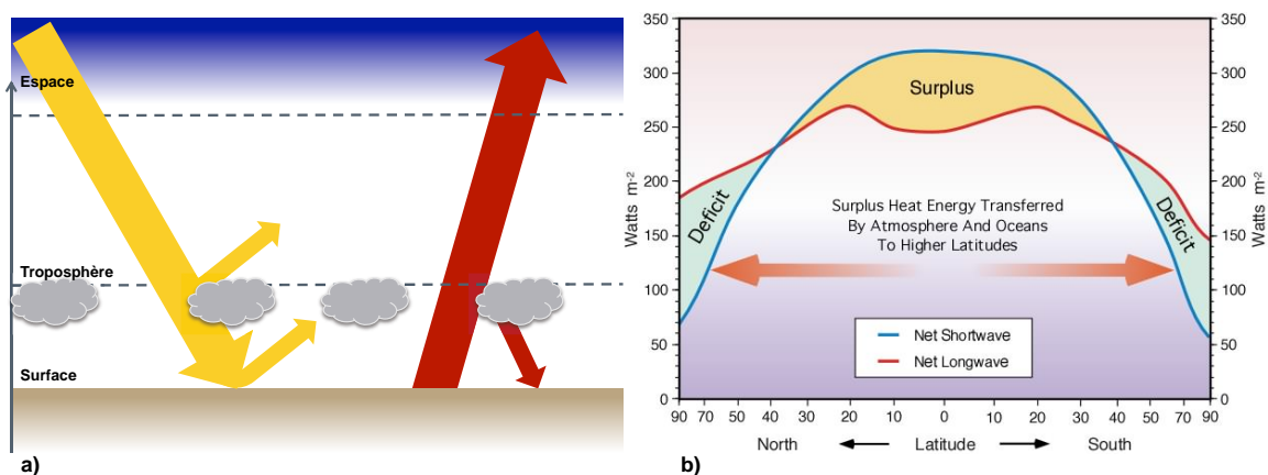
FIGURE 8 : GRAPHIQUE A : FLUX SOLAIRE INCIDENT EN JAUNE ET FLUX TERRESTRE EMIS EN ROUGE. GRAPHIQUE B : BILAN ENTRE LA MOYENNE DU FLUX ENTRANT NET (NET SHORTWAVE) ET DU FLUX SORTANT NET (NET LONGWAVE) ENTRE 90° SUD ET 90° NORD (SOURCE : ERBE).
