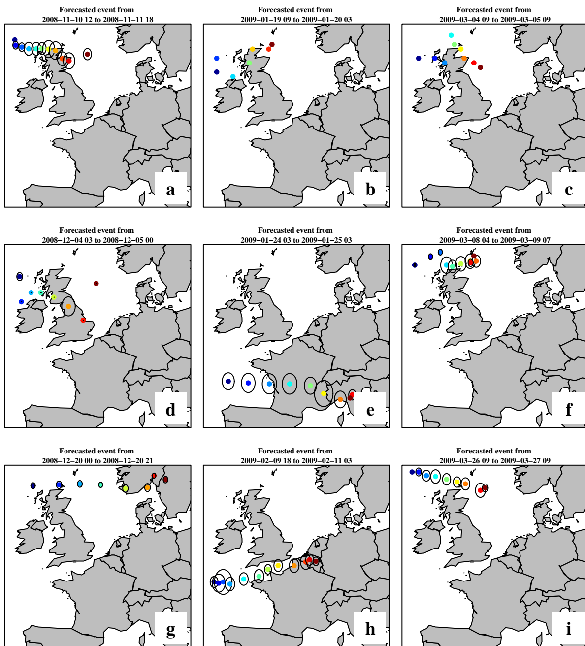
FIGURE 56 : ÉVÉNEMENTS AYANT DÉCLANCHÉS UNE ALERTE AU COURS DE LA PÉRIODE HIVERNALE ENTRE OCTOBRE 2008 ET MARS 2009. POUR CHAQUE ÉVÉNEMENT, LA TRAJECTOIRE MOYENNE EST TRACÉE AINSI QUE L'ÉCART-TYPE DE LA POSITION DE CHAQUE CENTRE. LES DEUX ÉVÉNEMENTS KLAUS ET QUINTEN ONT BIEN ÉTÉ DÉTECTÉS, RESPECTIVEMENT GRAPHIQUE E ET H.
