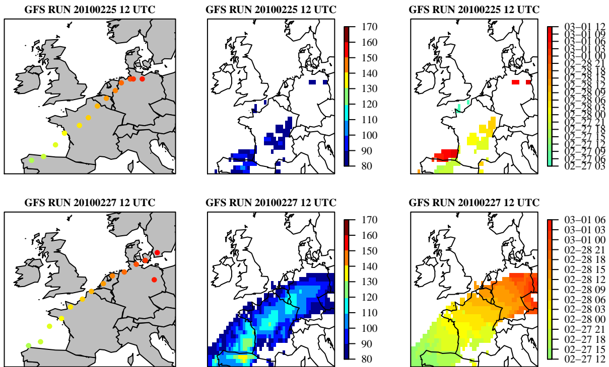
FIGURE 47 : RESULTATS DES ALERTES ISSUES DE L'ANALYSE DES PREVISIONS DU 25 FEVRIER 2010 12H (GRAPHIQUES SUPERIEURS) ET DU 27 FEVRIER 2010 12H (GRAPHIQUES INFERIEURS) : LA TRAJECTOIRE DE L'EVENEMENT (GAUCHE), L'EMPREINTE DE VENT (MILIEU) ET L'EMPREINTE TEMPORELLE DES VENTS SUPERIEURS A 80 KM/H (DROITE).
