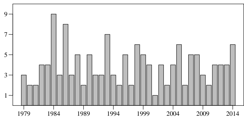
FIGURE 65 : DISTRIBUTION DU NOMBRE D'EVENEMENTS PAR AN POUR LES 142 EVENEMENTS DETECTES PAR LA METHODE MULTI-VARIABLE.
