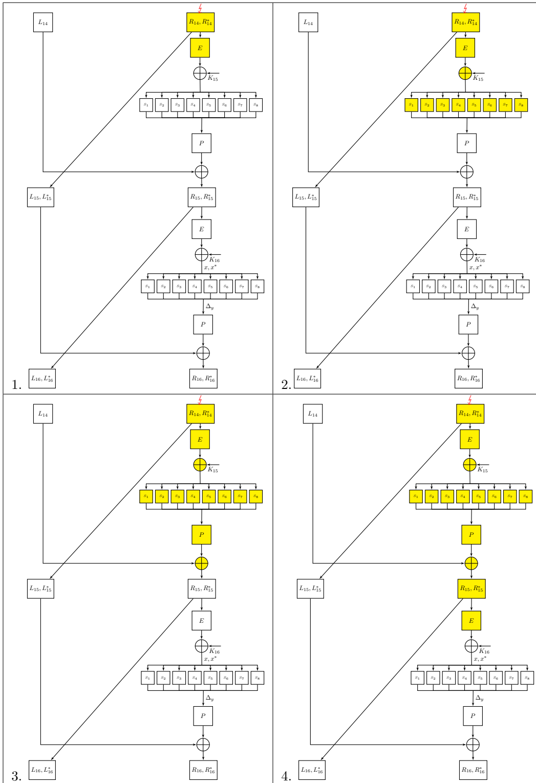
Figure 37 : Les différentes étapes importantes de la diffusion de la faute injectée
