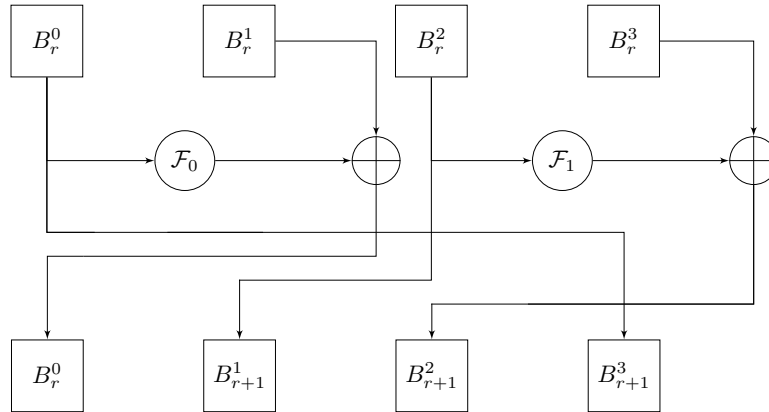
Figure 30 : Schéma de CLEFIA
