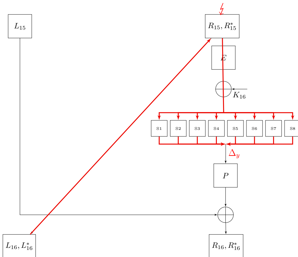
Figure 35 : Chemin d'attaque de FIRE
