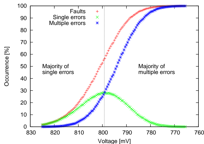
Figure 40 : Proportion de chiffrés fautés et proportion de chiffrés fautés dus à une faute mono-bit.
