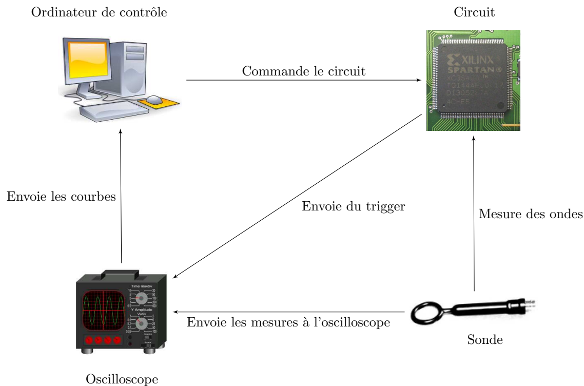
Figure 9 : Représentation schématique du banc EM.
