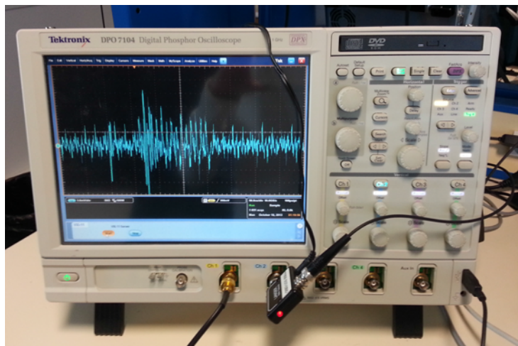
Figure 7 : Oscilloscope, sur l'écran nous pouvons voir l'exécution d'un AES.
