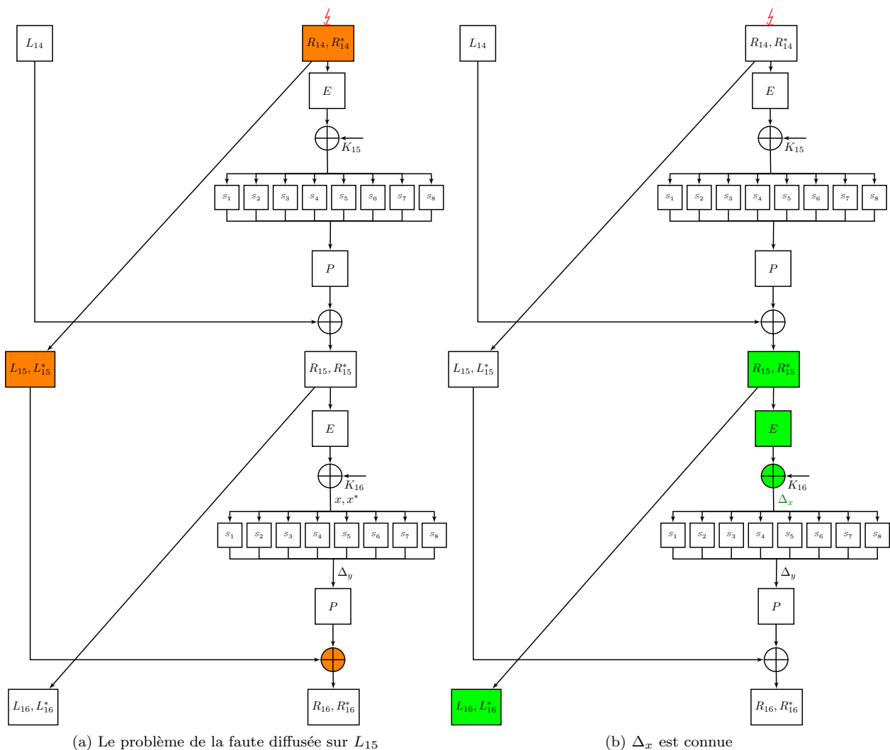
Figure 38 : Connaissance au dernier tour
