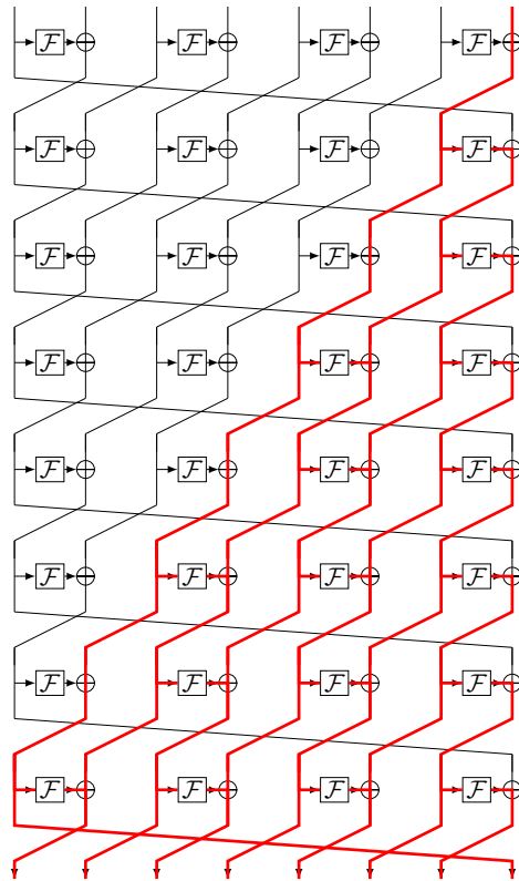
Figure 33 : Figure illustrant l'état de pleine diffusion d'un GFN.
