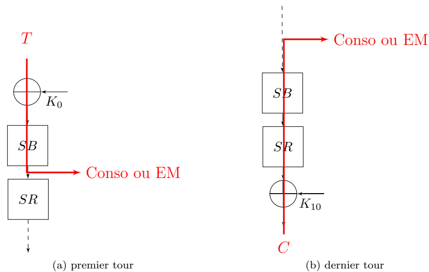
Figure 14 : Chemins d'attaques SCA sur AES
