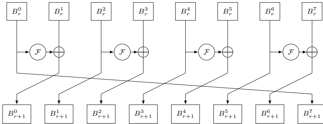
Figure 27 : Exemple de schéma de Feistel généralisé avec 8 blocs.
