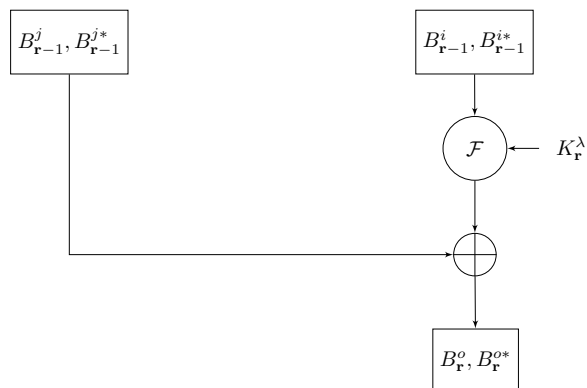
Figure 32 : Schéma d'attaque de type DFA dans un schéma de Feistel classique ou généralisé
