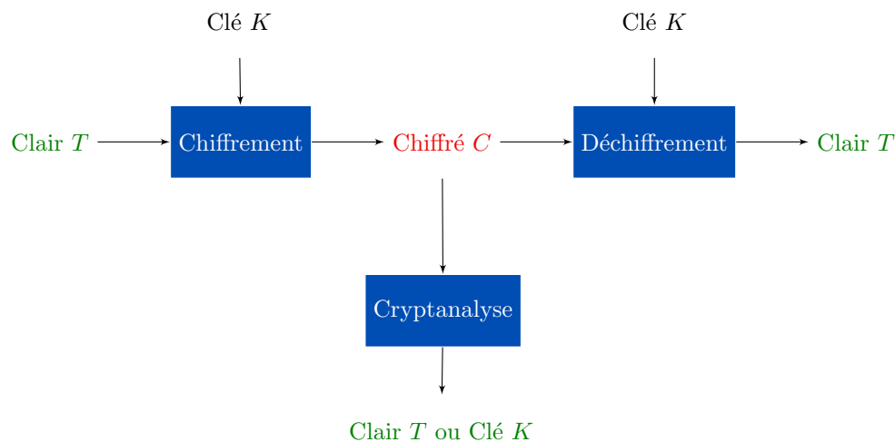
Figure 4 : Schéma de la cryptographie et de la cryptanalyse
