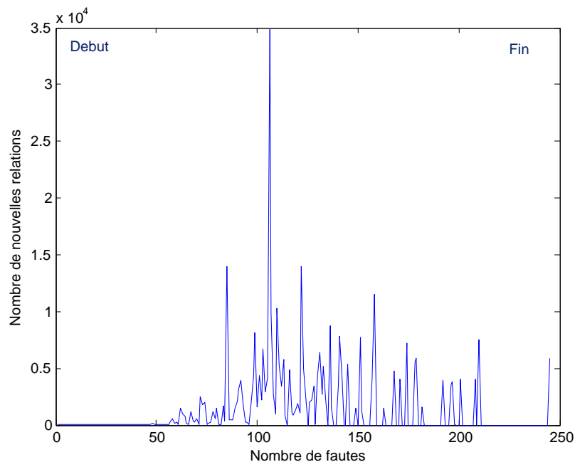
Figure 41 : Nombre de nouvelle(s) relation(s) (31) obtenue(s) à chaque faute injectée
