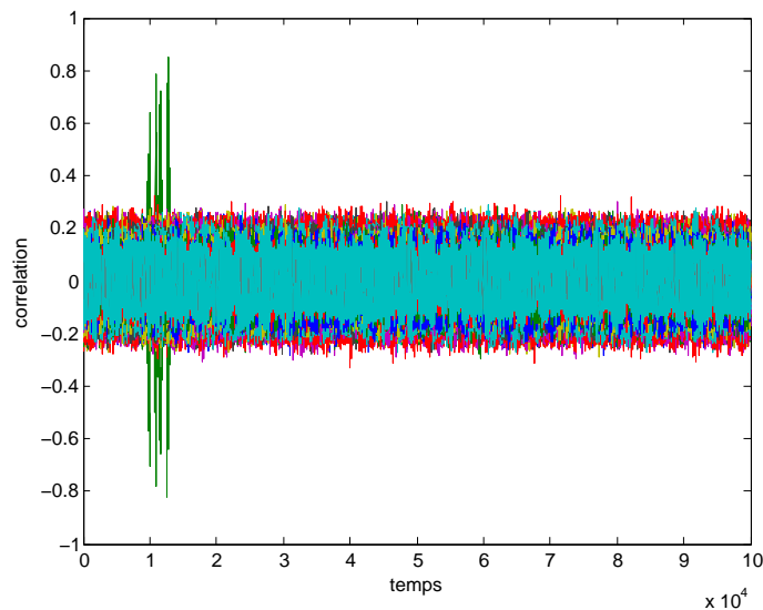
Figure 13 : Résultat d'une attaque CPA (Correlation Power Analysis) sur un AES implémenté dans un ATmega, du premier octet de clé du premier tour K_1^{0,0} . La bonne hypothèse de clé est associée à la courbe verte.
