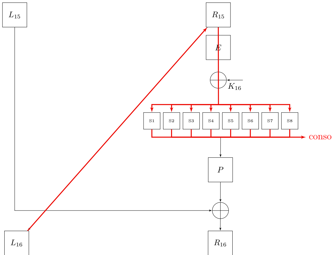
Figure 34 : Chemin d'attaque de SCARE
