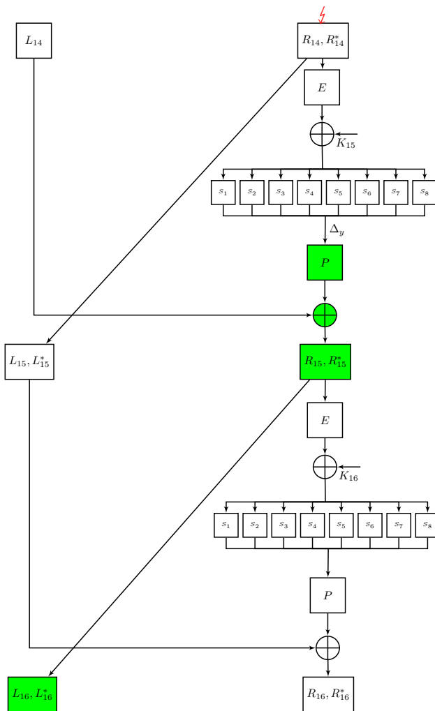
Figure 39 : Remontée au tour 15
