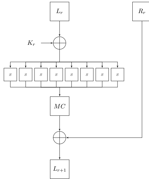
Figure 28 : Schéma de la fonction de Feistel du MIBS
