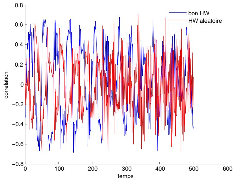
Figure 20 : Comparaison de la corrélation entre : les mesures et un vecteur de poids de Hamming aléatoire et les mesures et le bon vecteur de poids de Hamming pour une campagne de 10 textes. Les mesures sont issues d'un STM32.
