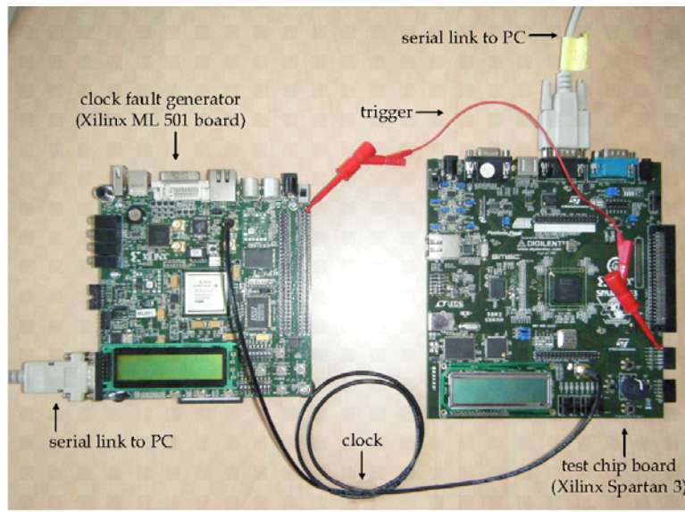
Figure 11 : Banc d'injection de fautes par glitches d'horloge
