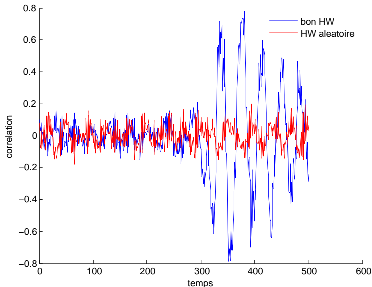
Figure 21 : Comparaison de la corrélation entre un vecteur de poids de Hamming aléatoire et le vecteur correct de poids de Hamming pour une campagne de 100 textes. Les mesures sont issues d'un STM32
