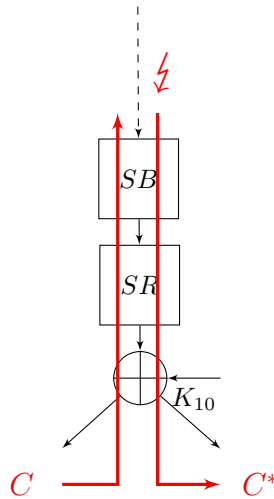
Figure 15 : Chemin d'attaque par injection de fautes sur AES au dernier tour
