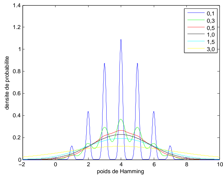
Figure 23 : Densités de probabilité des poids de Hamming bruités en fonction des différentes valeurs d'écart type \sigma . ( \sigma \in \{0,1; 0,2; 0,3; 0,5; 1; 1,5; 2; 3\} )
