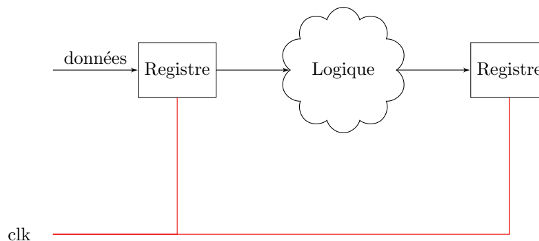
Figure 6 : Représentation de la logique synchrone
