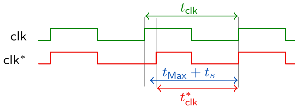
Figure 10 : Schéma du glitch d'horloge théoriquement injecté
