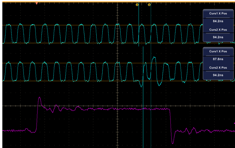
Figure 12 : Capture d'oscilloscope d'un glitch d'horloge
