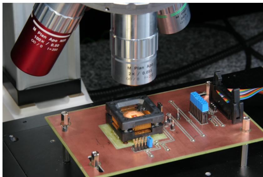
Figure 5 : Le laser, un outil semi-invasif pour injecter des fautes et réaliser des attaques. Le laser présenté ici, provient de la plateforme Micro-Packs .
