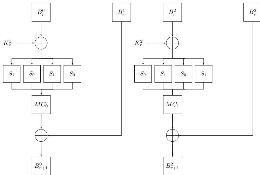
Figure 31 : Les fonctions de tours \mathcal{F}_0 et \mathcal{F}_1 de CLEFIA.
