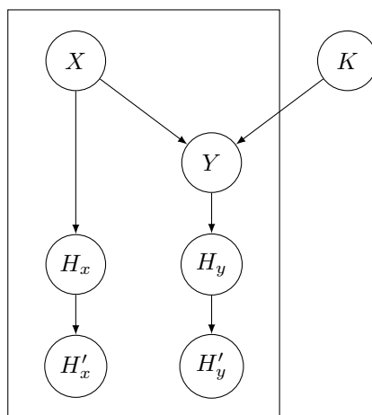
Figure 22 : Modélisation du problème par un graphe
