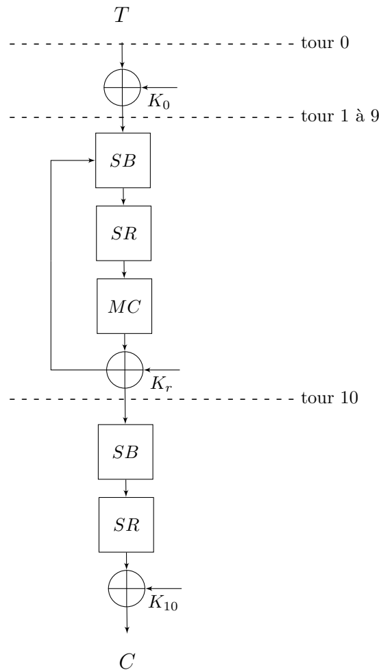
Figure 3 : Schéma de l'AES de 10 tours
