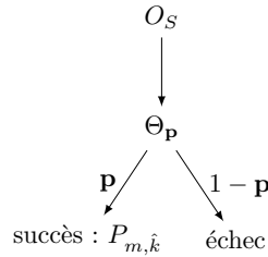
Figure 18 : Oracle avec une probabilité d'erreur \mathbf{p}
