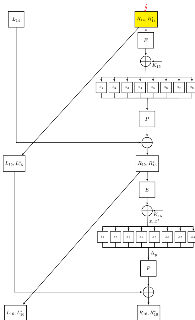
Figure 36 : Injection de la faute dans R_{14}
