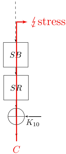
Figure 16 : Chemin d'attaque de la FSA sur AES.
