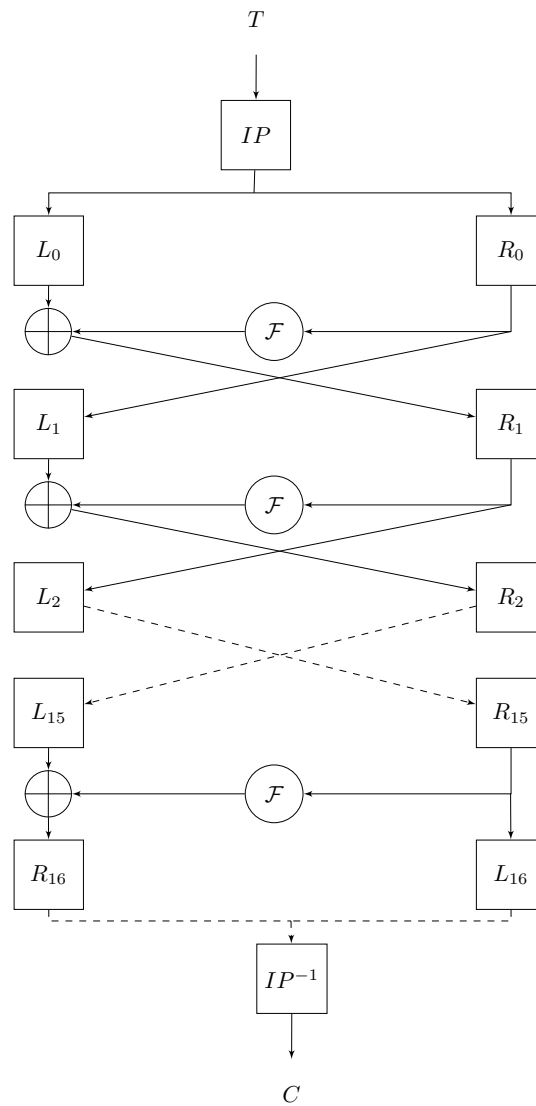
Figure 1 : Schéma général du Data Encryption Standard.
