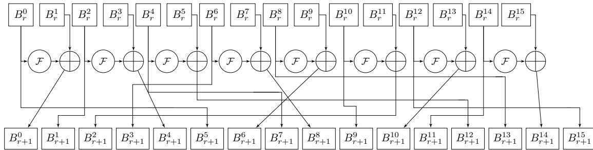
Figure 29 : Schéma de TWINE
