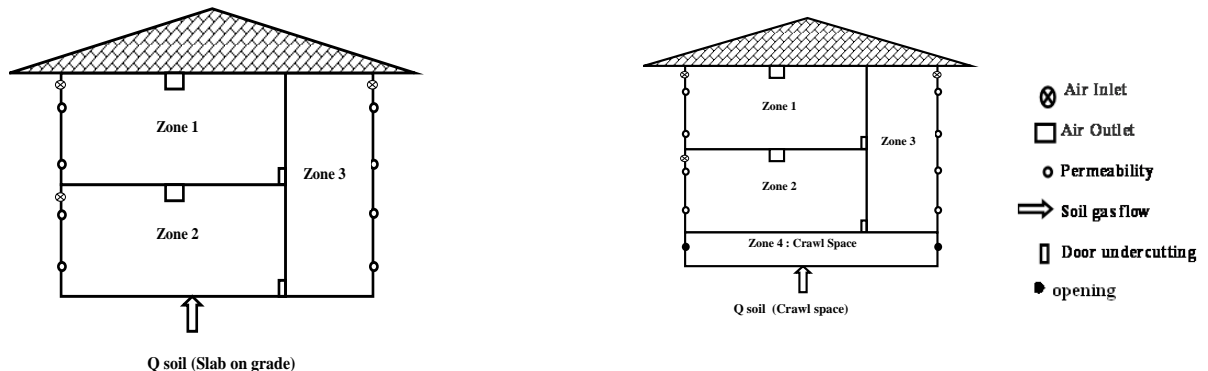
Figure 2.38 : schéma aéraulique (Diallo et al., 2012 )
