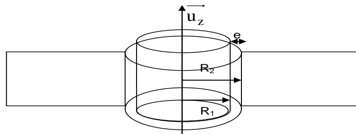
Figure 2.35 : écoulement entre deux cylindres coaxiaux
