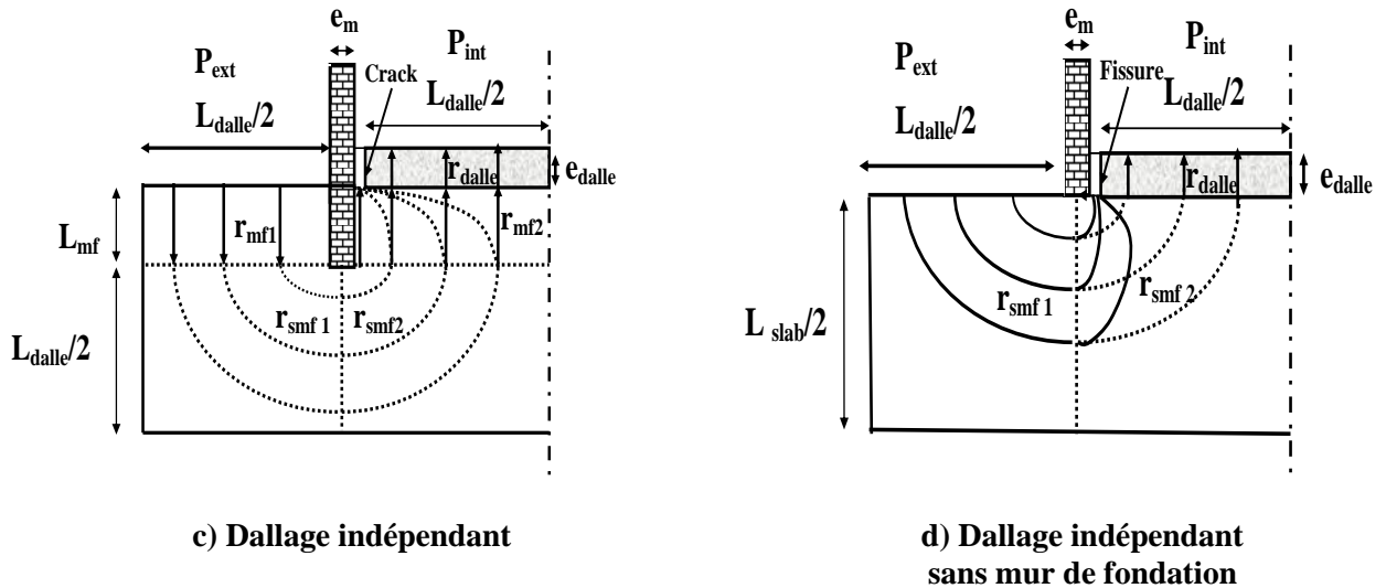
Figure 2.10 : Typologies sans murs enterrés, a) sol nu/vidé sanitaire, b) dalle portée, c) dallage indépendant d) dallage indépendant sans mur de fondation
