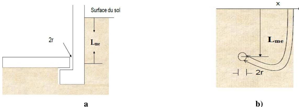
Figure 1.13 : Entrée d'air du sol vers le soubassement a) joint plancher-mur ; b) cylindre enterré avec un axe horizontal (Nazaroff, 1988 ; Abdelouhab, 2011).
