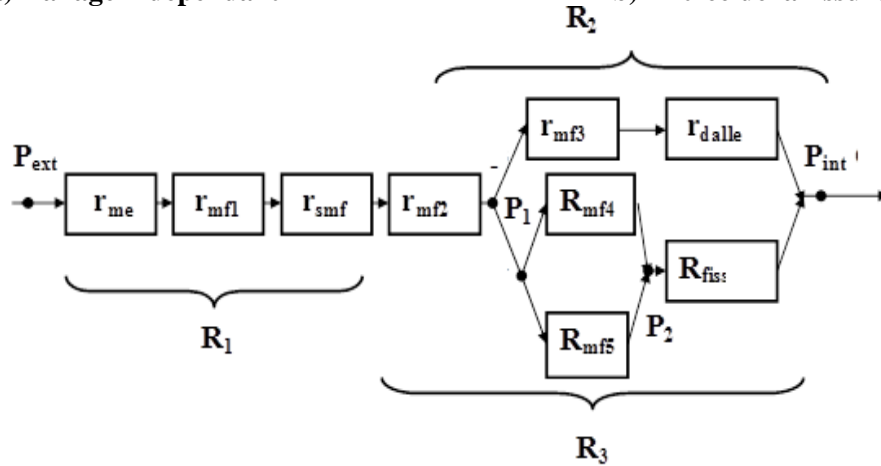
c) Réseau de résistances
