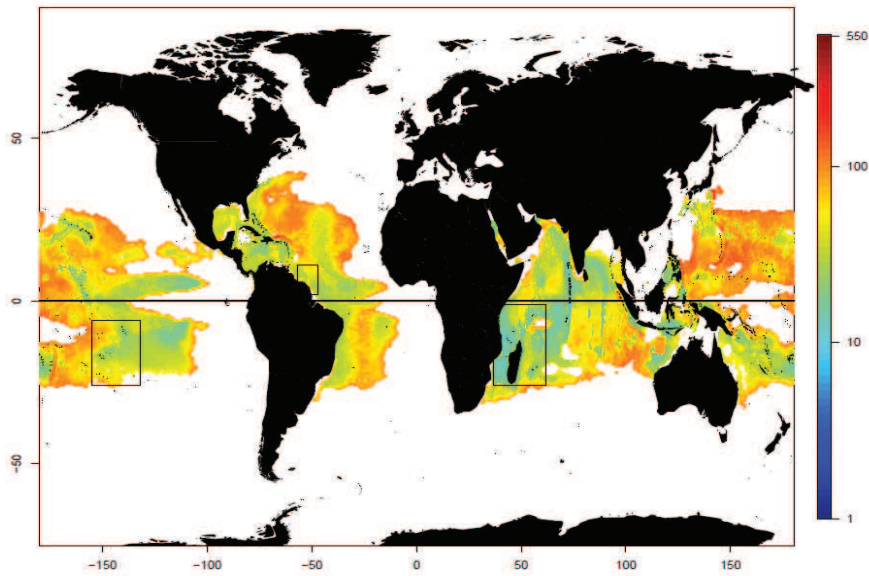
b Globicephalinae
