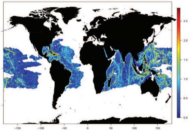
Slope (°) (square-root transformation)
