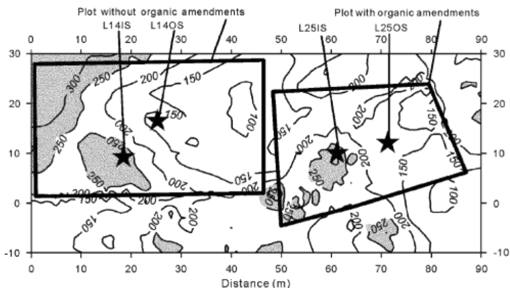
Figure 19 : Emplacement des points de suivis en fonction de la conductivité des sols. [AC10]. Les casiers à riz sont les mêmes qu'en Figure 17.
