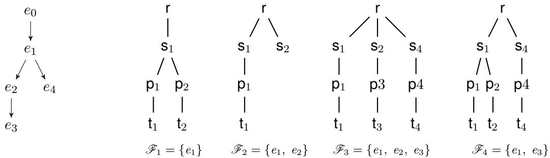
FIGURE B.3 – a) graphe d'espace de versions ; (b) 4 versions et leurs valeurs de vérité
