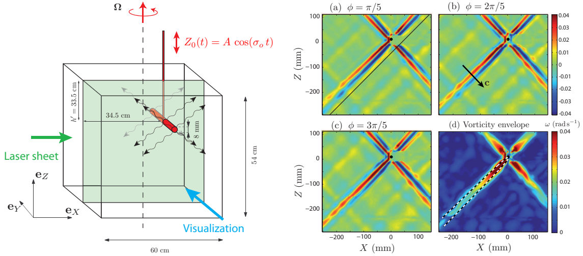
FIGURE 1.3 – Gauche : Vue schématique de l'expérience. Un cylindre de 8 mm de diamètre est oscillé verticalement selon Z_0(t) = A \cos(\sigma_0 t) avec A = 2 mm et \sigma_0/2\pi = 0.2 Hz. Des mesures de PIV sont réalisées dans le plan vertical (X, Z) dans le référentiel tournant. Droite : Champ de vorticité \omega_Y pour \sigma_0/2\Omega = 0.67 à différentes phases (a) \phi = \pi/5 , (b) \phi = 2\pi/5 et (c) \phi = 3\pi/5 . La ligne noire dans la figure (a) indique la direction de propagation prédite par la relation de dispersion. (d) montre l'enveloppe des oscillations de vorticité. La ligne pointillée noire et blanche reporte la prédiction de l'épaisseur du faisceau selon la théorie de similitude.
