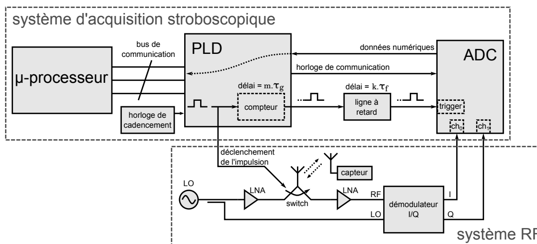
FIGURE 4.6 – Schéma de principe du prototype de la méthode stroboscopique pour l'interrogation de lignes à retard à ondes élastiques, utilisées comme capteur, par méthode de RADAR impulsionnel.
