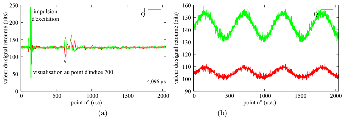
FIGURE 4.15 – Acquisition des signaux en phase et en quadrature de phase de la réponse de la ligne à retard en temps-réel pour une durée de 4,096 μs (a) et visualisation des variations des signaux, au point de mesure d'indice 700, sur 2048 acquisitions (b).
