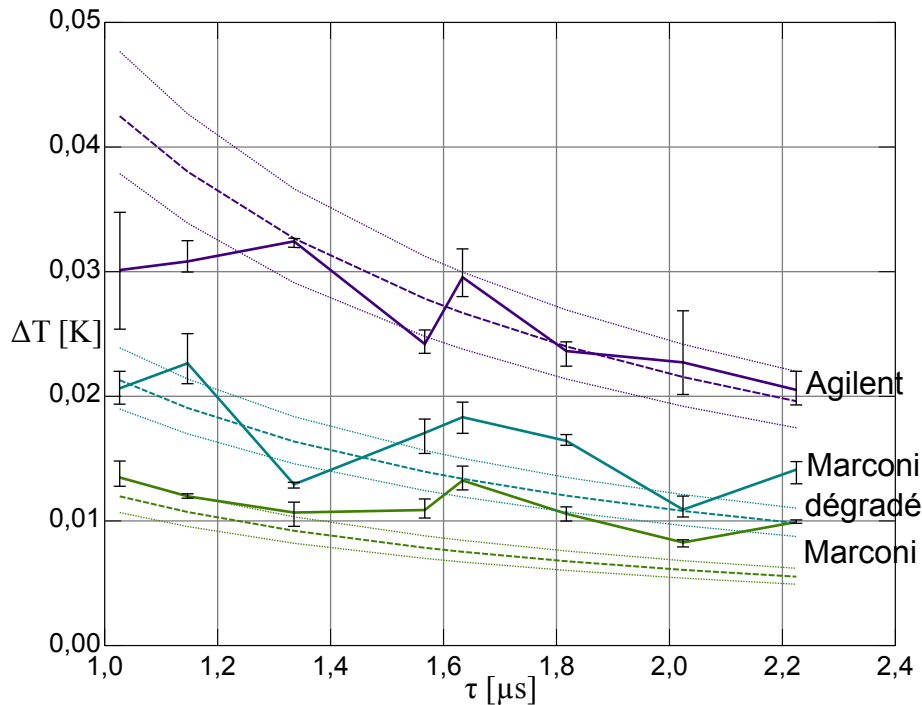
FIGURE 2.10 – Fluctuations de température correspondant aux fluctuations de phase ainsi que les valeurs théoriques des résolutions de mesure imposées pour L(f) = -135 \pm 1 \text{ dBc.Hz}^{-1} , L(f) = -130 \pm 1 \text{ dBc.Hz}^{-1} , L(f) = -124 \pm 1 \text{ dBc.Hz}^{-1} .
