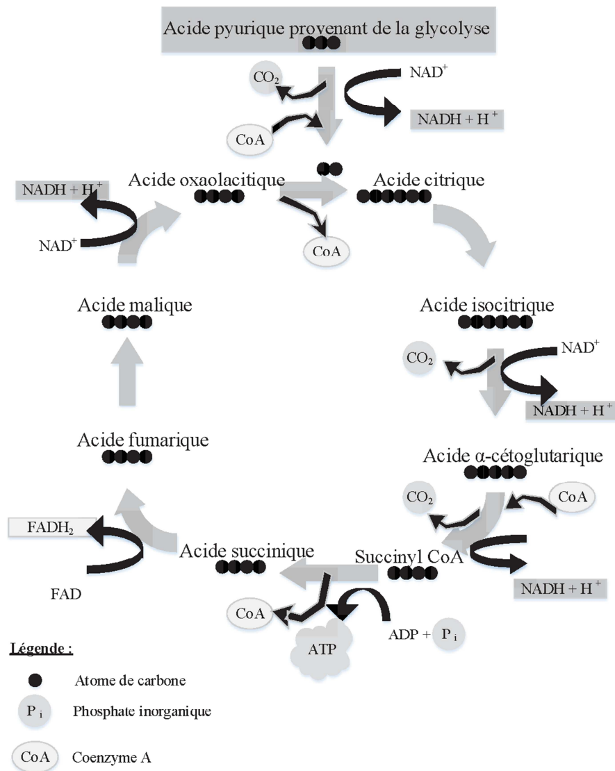
Figure 4. Cycle de l'acide citrique (cycle de Krebs).
