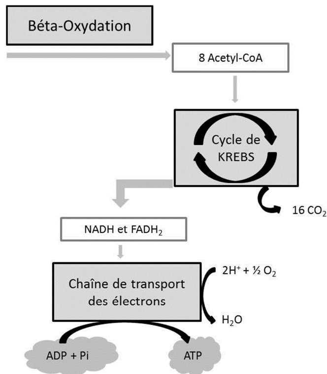
Figure 5. Oxydation totale des acides gras non estérifiés.
